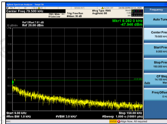
GSM1900-512-0-0.009~0.15MHz-PASS
