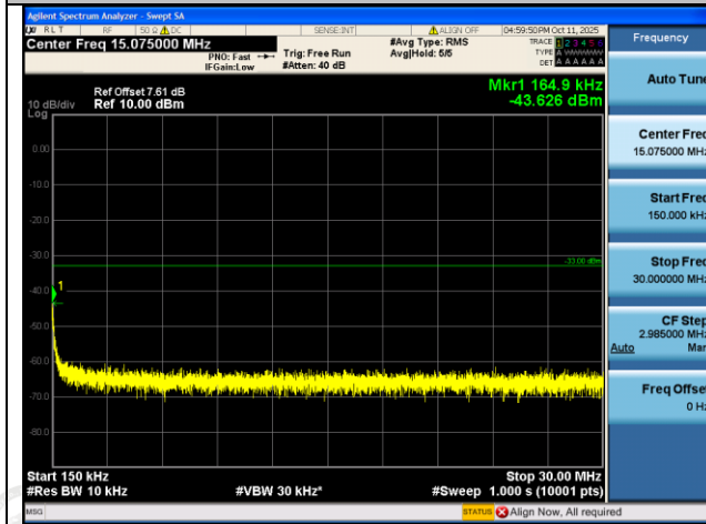
GSM1900-512-0-0.15~30MHz-PASS
