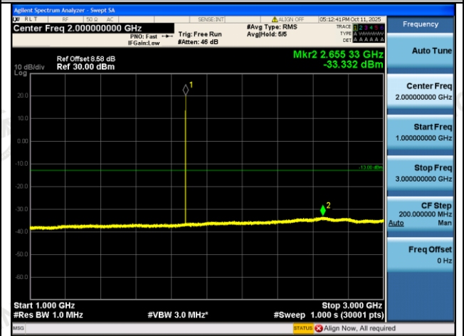
GPRS1900-661-0-1000~3000MHz-PASS
