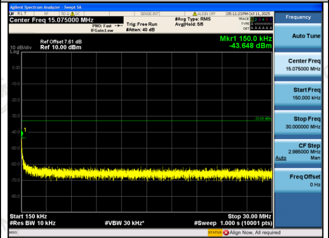
GPRS1900-512-0-0.15~30MHz-PASS
