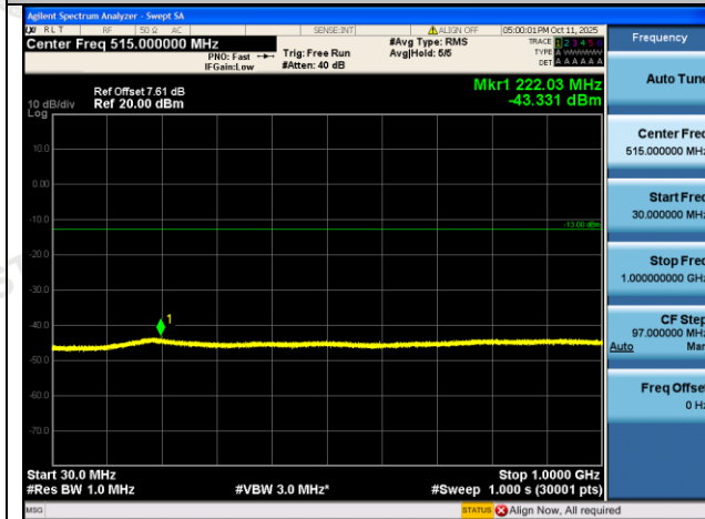
GSM1900-512-0-30~1000MHz-PASS
