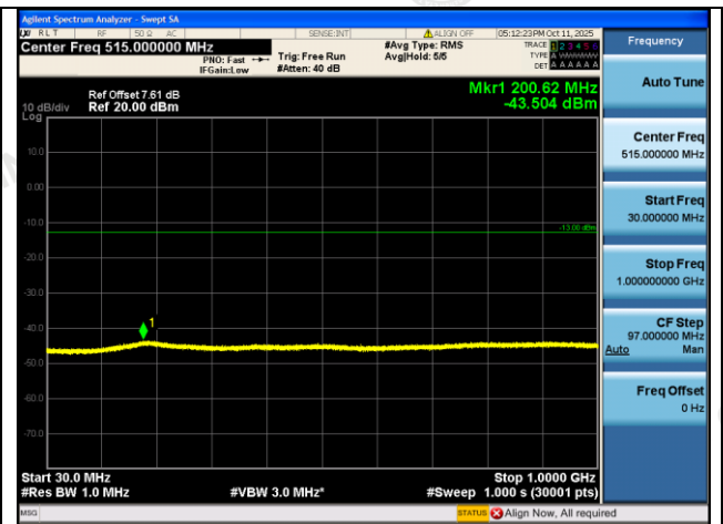
GPRS1900-661-0-30~1000MHz-PASS
