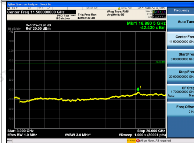
GSM1900-661-0-3000~20000MHz-PASS
