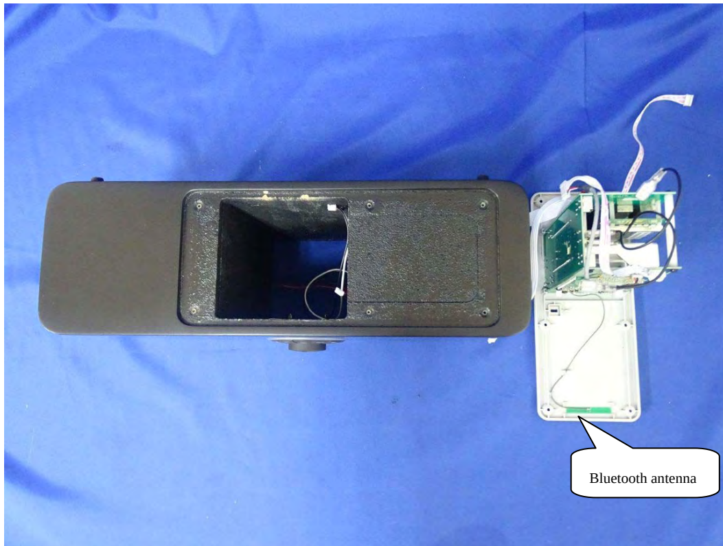
(13) EUT Photo
