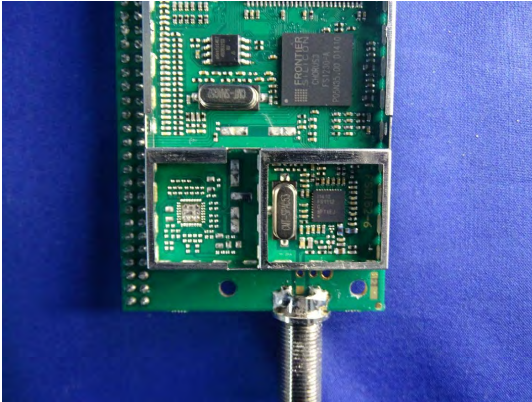
(37) EUT Photo
