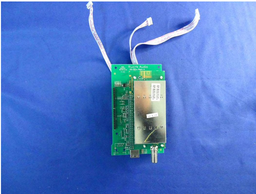
(30) EUT Photo
