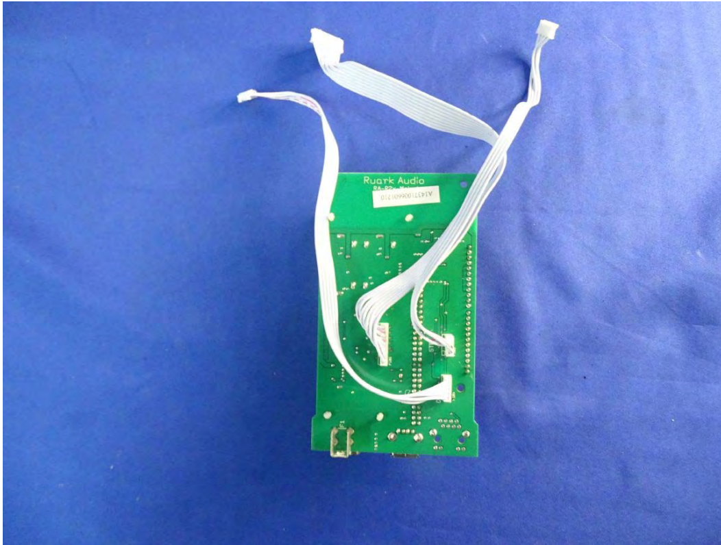
(33) EUT Photo
