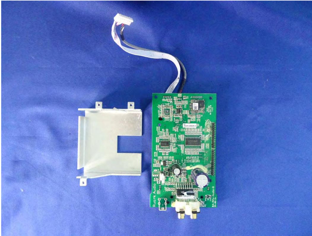
(21) EUT Photo
