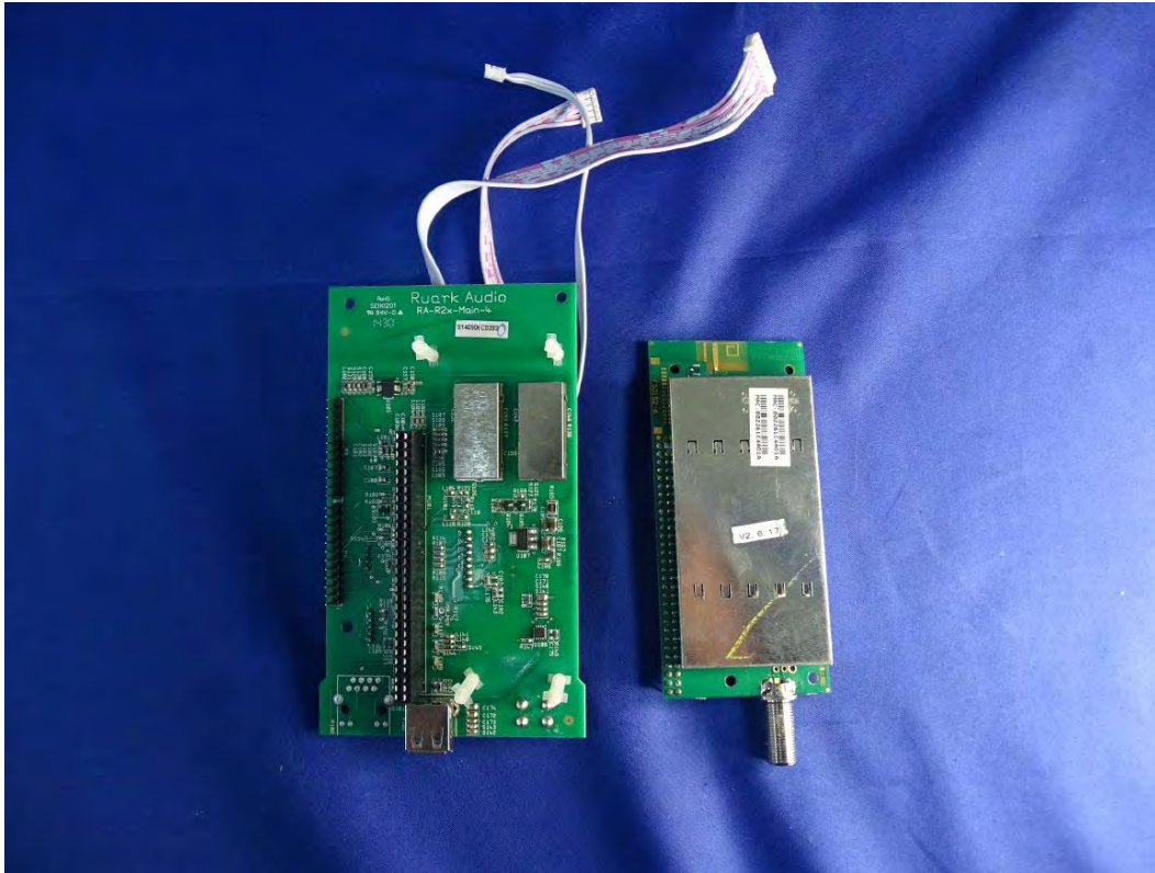
(31) EUT Photo
