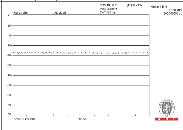
802.11n (HT40)
