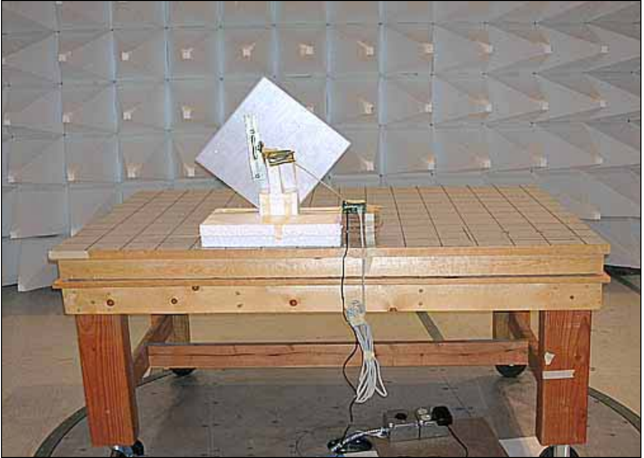
15.247(d) 23dBi Antenna Back
