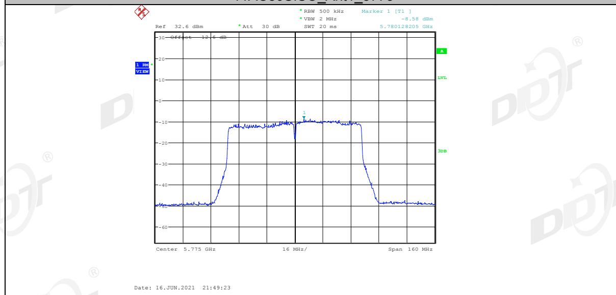
11AC80SISO_Ant1_5775
