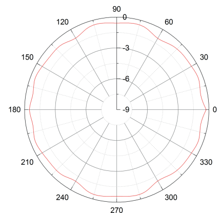
H-Plane
