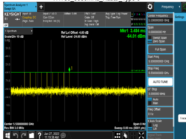
VHT80_5530MHz_Radar_Type 6
