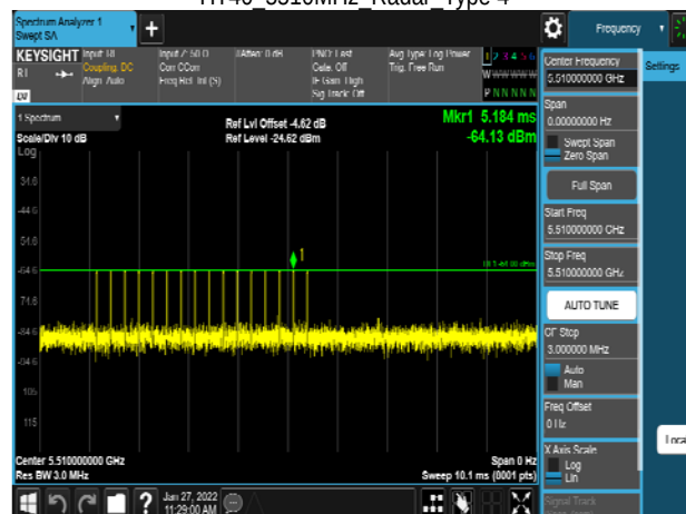
HT40_5510MHz_Radar_Type 4
