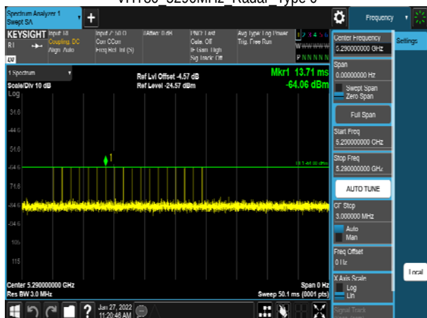
VHT80_5290MHz_Radar_Type 0
