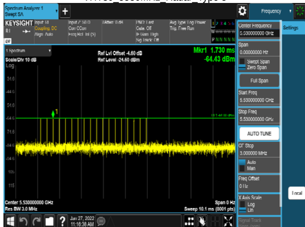
VHT80_5530MHz_Radar_Type 3
