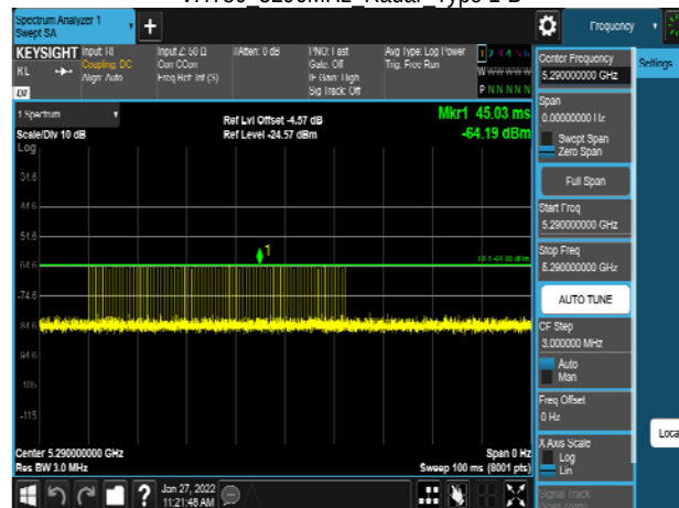
VHT80_5290MHz_Radar_Type 2
