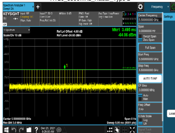
HT20_5500MHz_Radar_Type 2
