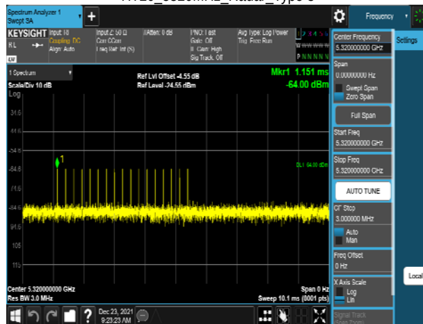
HT20_5320MHz_Radar_Type 4
