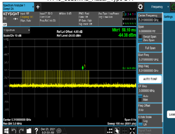
HT40_5310MHz_Radar_Type 1-A
