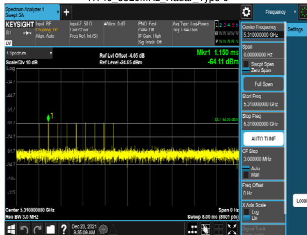
HT40_5310MHz_Radar_Type 6
