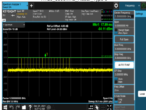
HT20_5500MHz_Radar_Type 0
