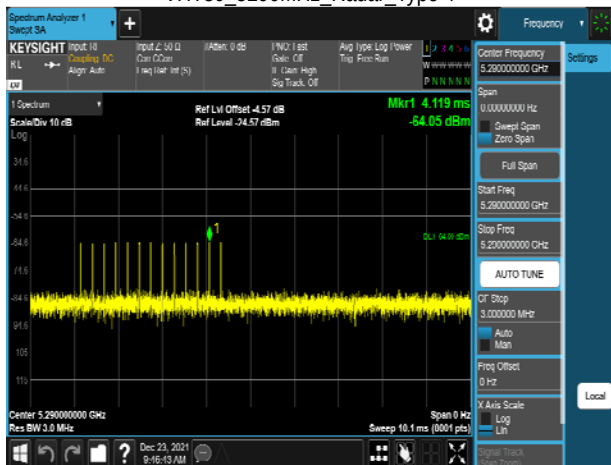
VHT80_5290MHz_Radar_Type 5
