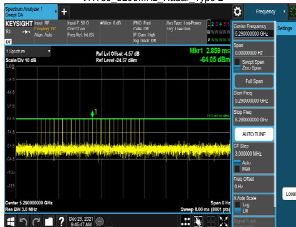
VHT80_5290MHz_Radar_Type 2
