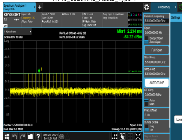
HT40_5510MHz_Radar_Type 4
