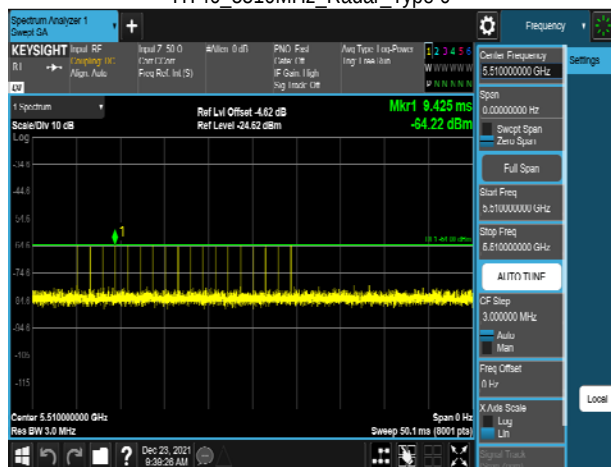
HT40_5510MHz_Radar_Type 1-A
