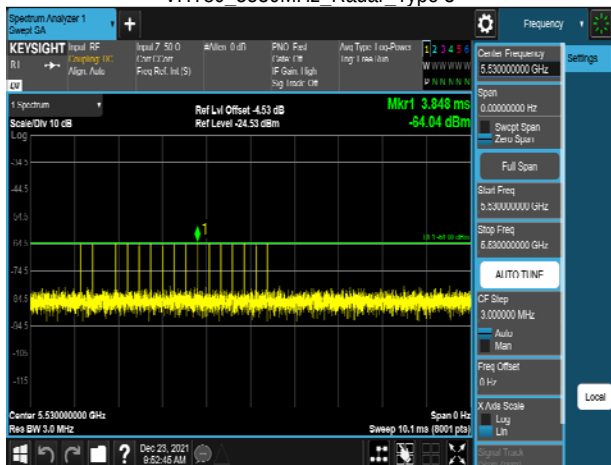
VHT80_5530MHz_Radar_Type 3
