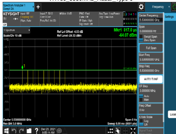
VHT80_5530MHz_Radar_Type 6
