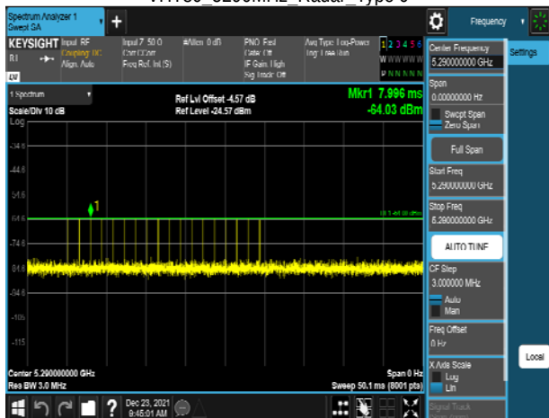
VHT80_5290MHz_Radar_Type 0
