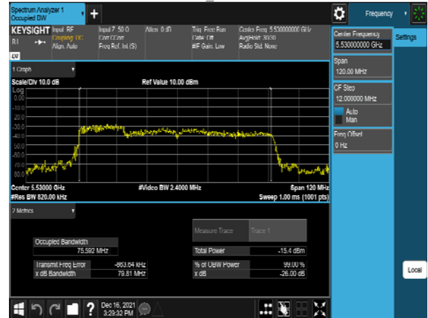
VHT80_5530MHz
