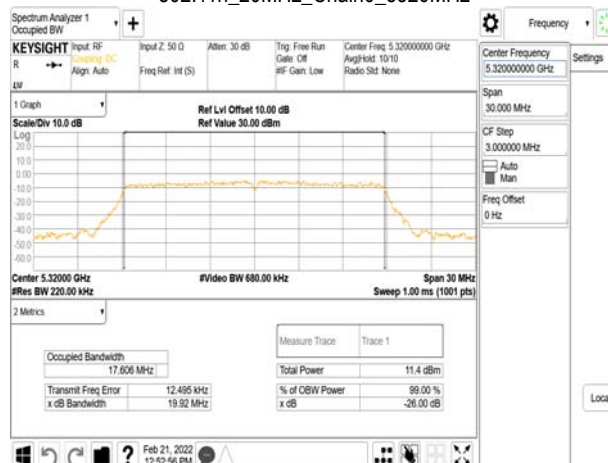
802.11n_20MHz_Chain0_5320MHz
