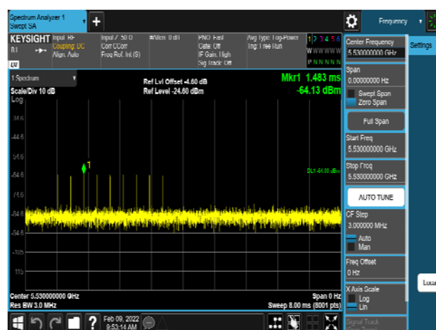
VHT80_5530MHz_Radar_Type 6
