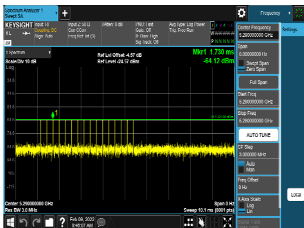
VHT80_5290MHz_Radar_Type 5
