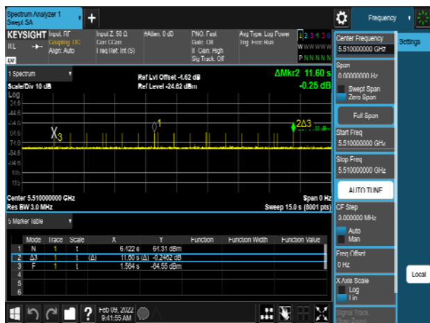
HT40_5510MHz_Radar_Type 6
