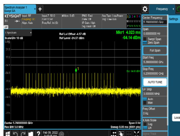
VHT80_5290MHz_Radar_Type 2
