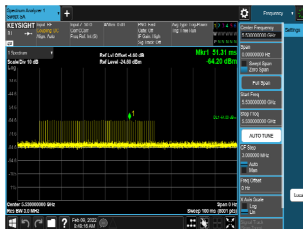
VHT80_5530MHz_Radar_Type 1-A
