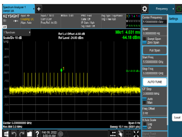
VHT80_5530MHz_Radar_Type 3
