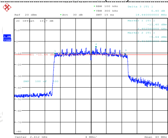
802.11ax(HT20)
