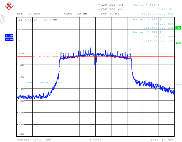
802.11n(HT40)
