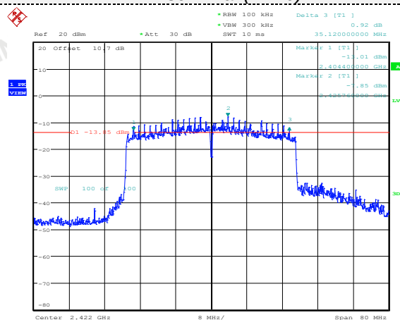
802.11ax(HT40)
