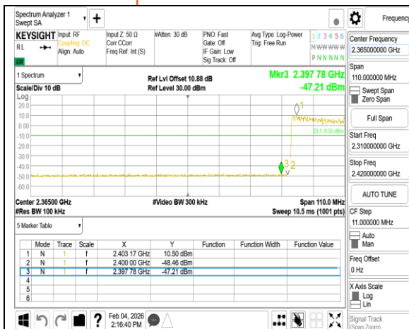
Hopping Band Edge 8DPSK 3M DH5 2402MHz
