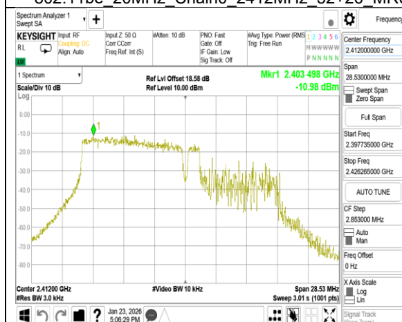
802.11be 20MHz Chain0 2412MHz 106+26 MRU1
