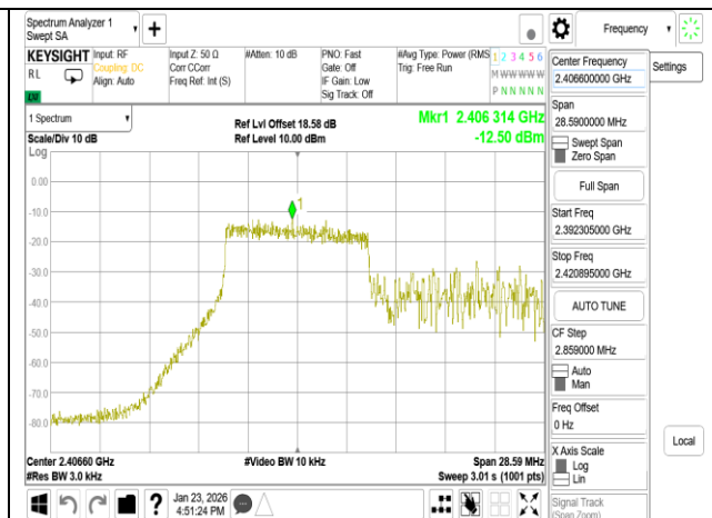
802.11be 20MHz Chain1 2412MHz RU106 53
