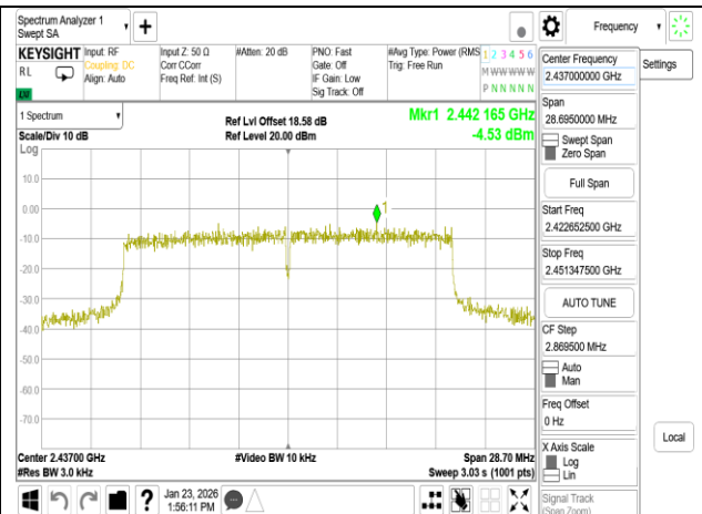
802.11be 20MHz Chain1 2437MHz RU242
