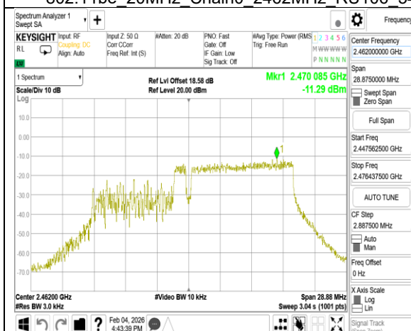
802.11be 20MHz Chain0 2462MHz 106+26 MRU2
