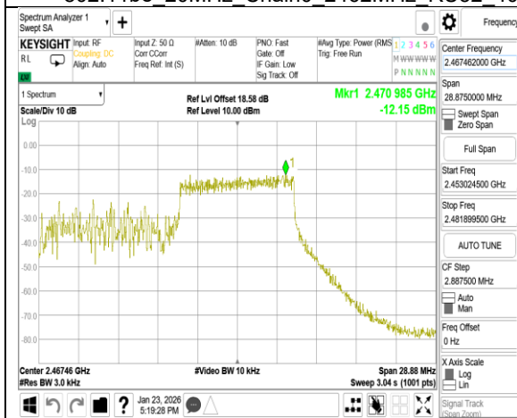
802.11be 20MHz Chain0 2462MHz RU106_54
