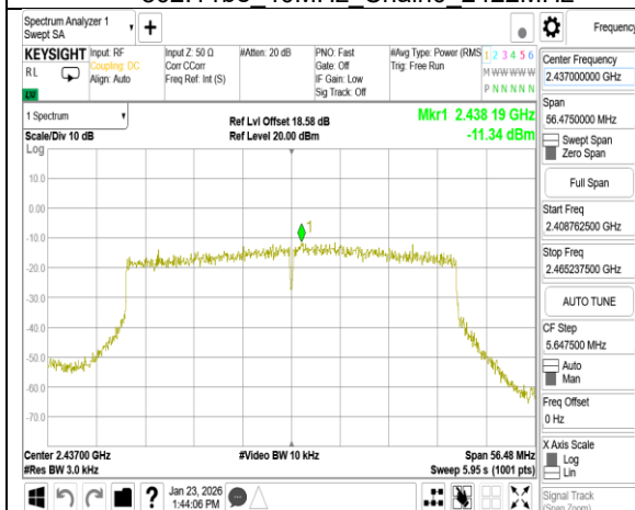
802.11be 40MHz Chain0 2437MHz
