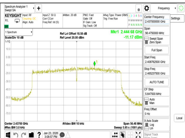
802.11be 40MHz Chain0 2437MHz RU484
