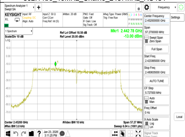
802.11be 40MHz Chain0 2452MHz RU484
