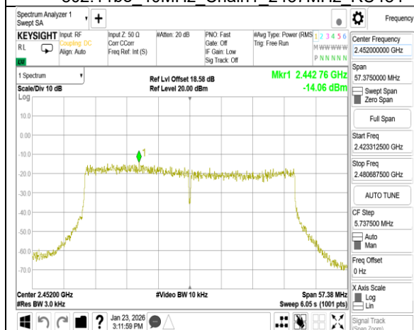
802.11be 40MHz Chain1 2452MHz RU484
