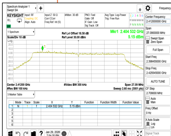
802.11be_20MHz_Chain0_2412MHz
