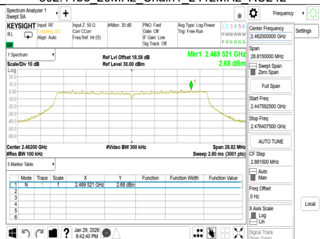
802.11be 20MHz Chain1 2462MHz RU242
