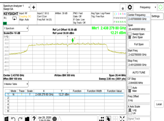
802.11be_20MHz_Chain0_2437MHz
