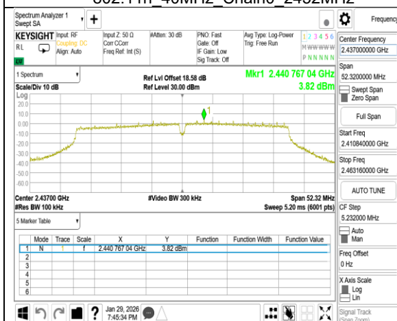
802.11n 40MHz Chain1 2437MHz
