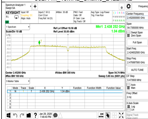
802.11n 40MHz Chain0 2452MHz
