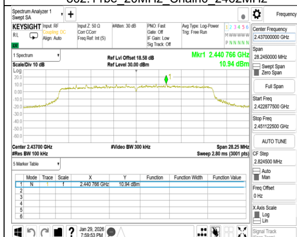
802.11be_20MHz_Chain1_2437MHz
