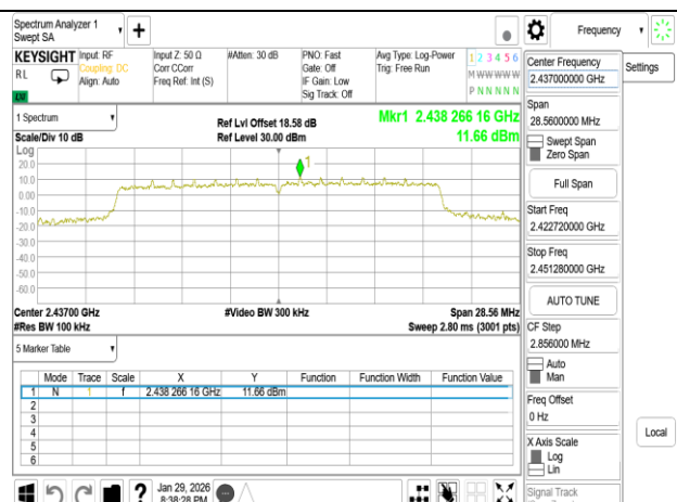
802.11be 20MHz Chain0 2437MHz RU242
