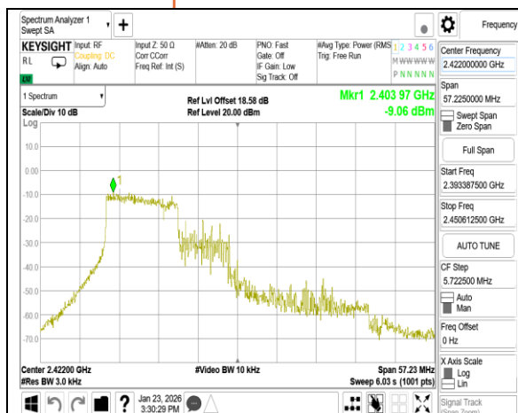
802.11be 40MHz Chain1 2422MHz 106+26 MRU1
