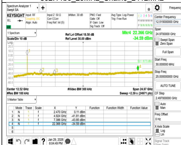
802.11be_20MHz_Chain0_2462MHz
