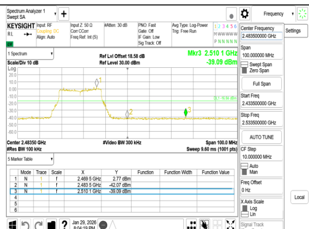
802.11be 20MHz Chain1 2462MHz
