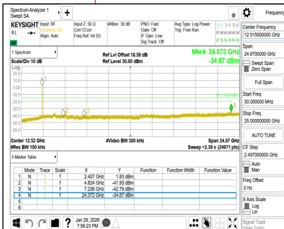
802.11be_20MHz_Chain0_2412MHz
