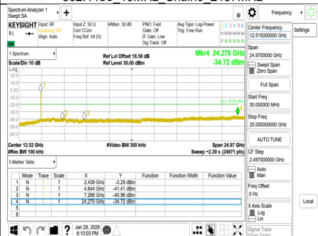
802.11be 40MHz Chain1 2422MHz
