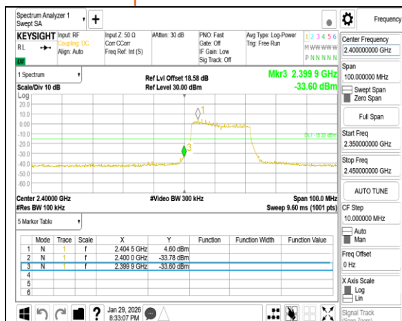
802.11be 20MHz Chain0 2412MHz RU242
