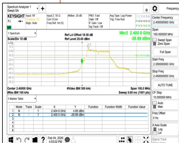
802.11g_20MHz_Chain1_2412MHz
