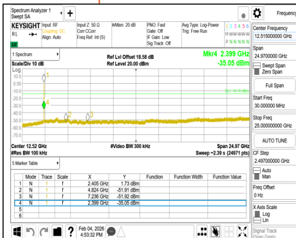
802.11g 20MHz Chain0 2412MHz
