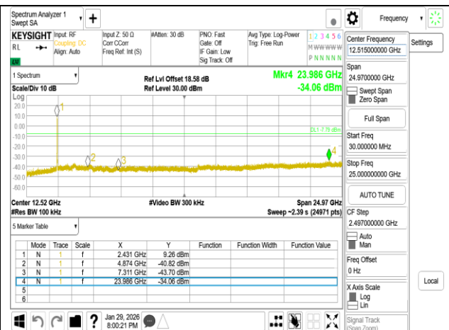
802.11be_20MHz_Chain0_2437MHz
