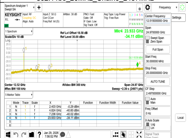
802.11be_20MHz_Chain1_2412MHz
