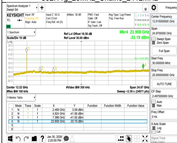
802.11g 20MHz Chain0 2462MHz
