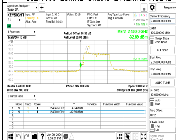
802.11be 20MHz Chain1 2412MHz RU242
