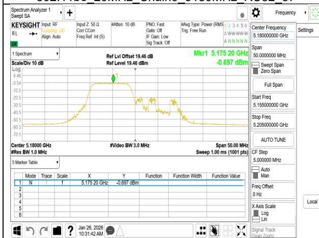
802.11be 20MHz Chain0 5180MHz RU106 53
