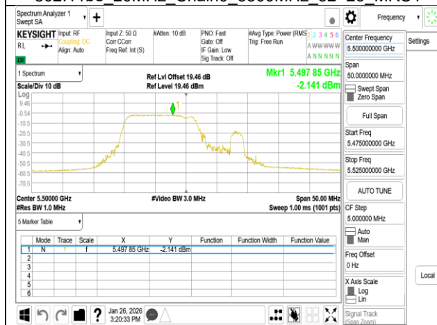
802.11be 20MHz Chain0 5500MHz 106+26 MRU1
