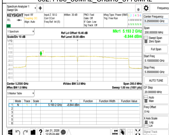
802.11be_160MHz_Chain0_5250MHz
