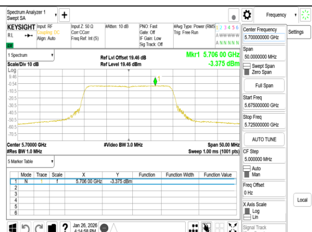
802.11be 20MHz Chain1 5700MHz RU242
