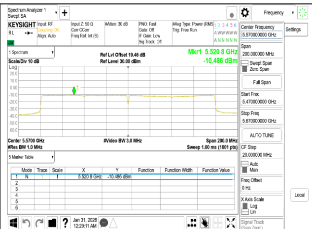
802.11be_160MHz_Chain1_5570MHz
