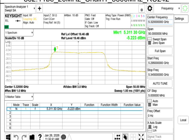
802.11be 20MHz Chain1 5320MHz RU242
