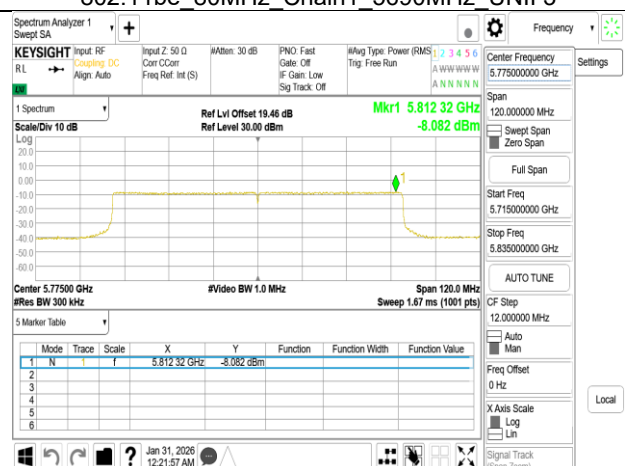
802.11be_80MHz_Chain1_5775MHz
