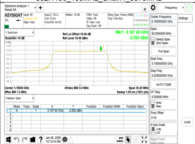
802.11be_20MHz_Chain1_5180MHz_RU242
