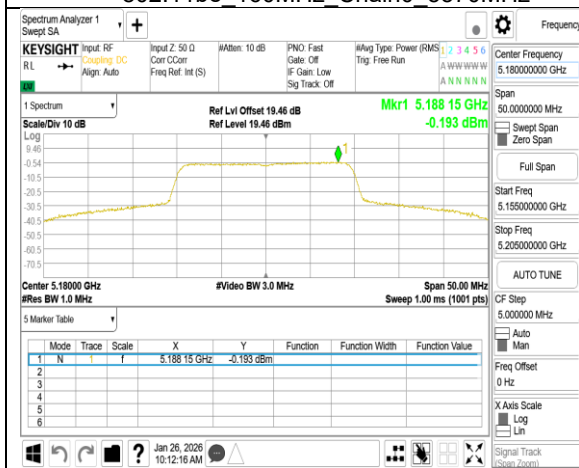
802.11be_20MHz_Chain0_5180MHz_RU242
