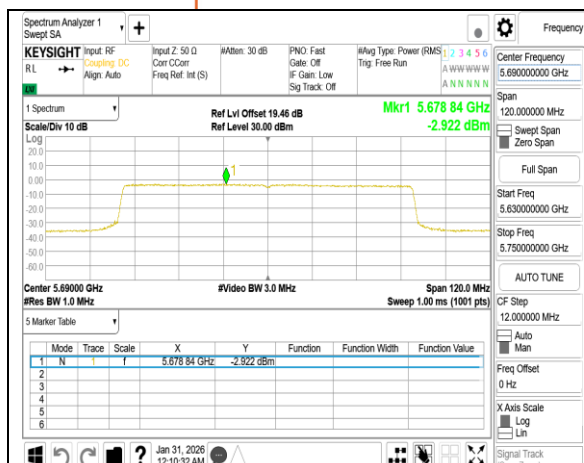
802.11be_80MHz_Chain1_5690MHz_UNII 2C
