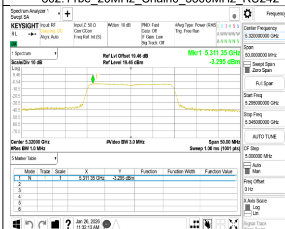
802.11be 20MHz Chain0 5320MHz RU242
