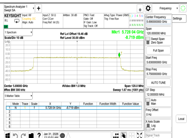
802.11be_80MHz_Chain1_5690MHz_UNII 3
