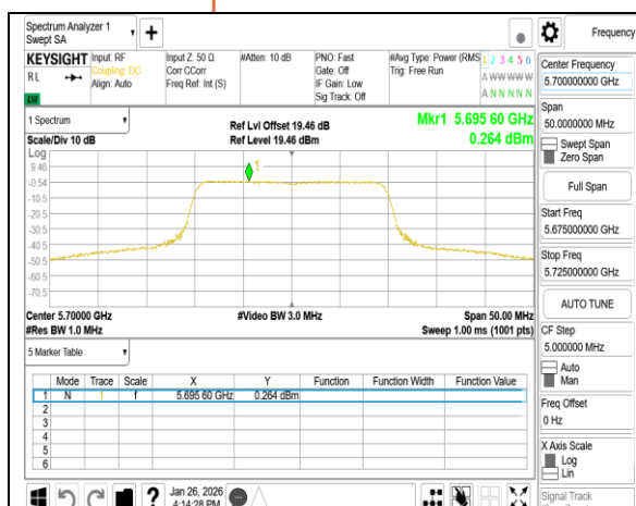
802.11be 20MHz Chain0 5700MHz RU242
