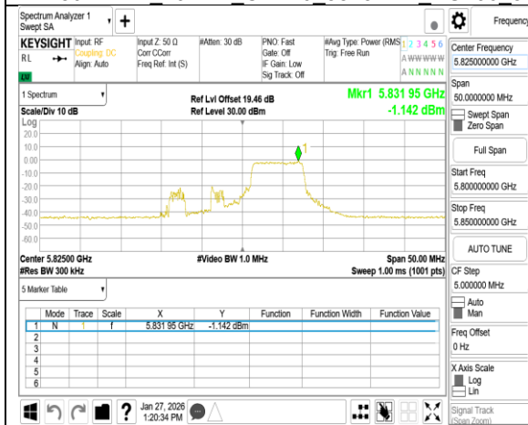
802.11be 20MHz Chain0 5825MHz 52+26 MRU3
