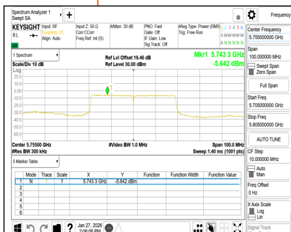
802.11be 40MHz Chain0 5755MHz RU484
