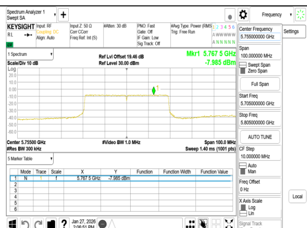
802.11be 40MHz Chain1 5755MHz RU484
