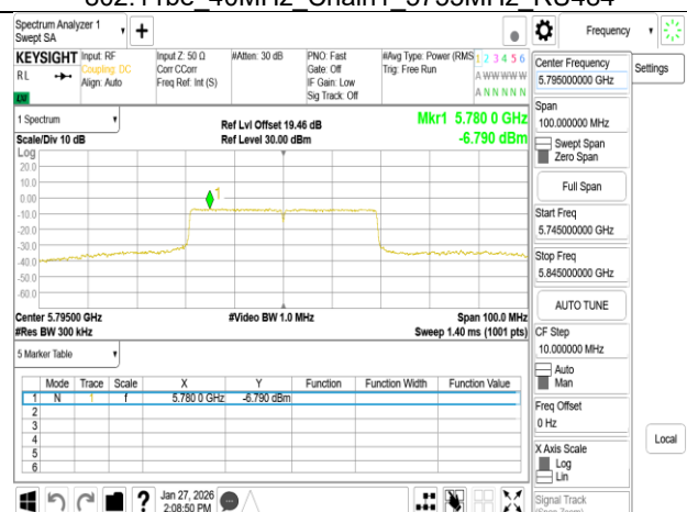
802.11be 40MHz Chain1 5795MHz RU484
