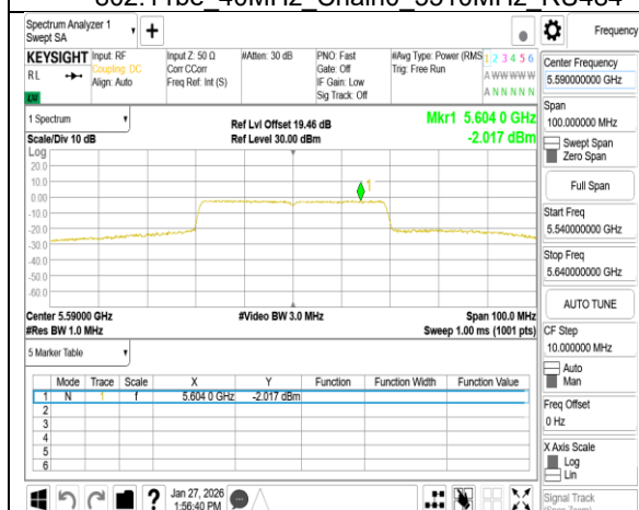
802.11be_40MHz_Chain0_5590MHz_RU484
