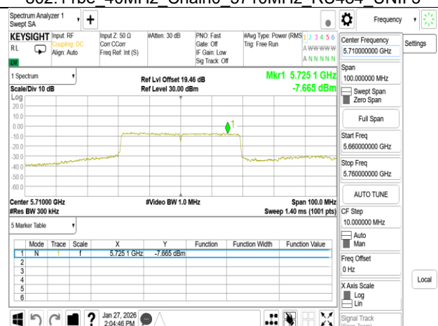
802.11be 40MHz Chain1 5710MHz RU484 UNII 3
