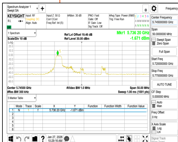
802.11be 20MHz Chain0 5745MHz RU26 0
