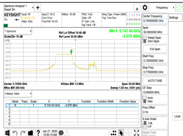
802.11be 20MHz Chain1 5745MHz 52+26 MRU1
