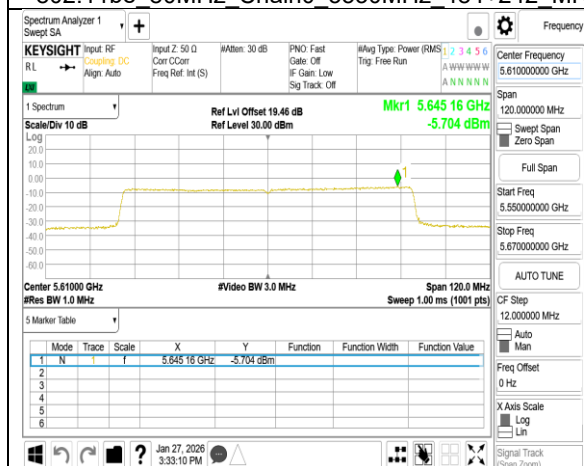
802.11be 80MHz Chain0 5610MHz RU996
