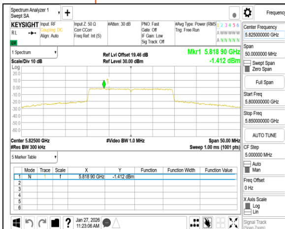
802.11be 20MHz Chain0 5825MHz RU242
