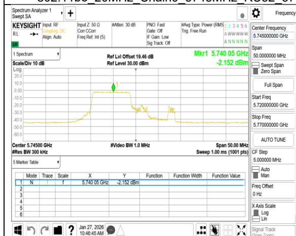
802.11be 20MHz Chain0 5745MHz RU106 53
