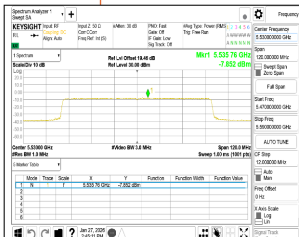
802.11be 80MHz Chain0 5530MHz RU996
