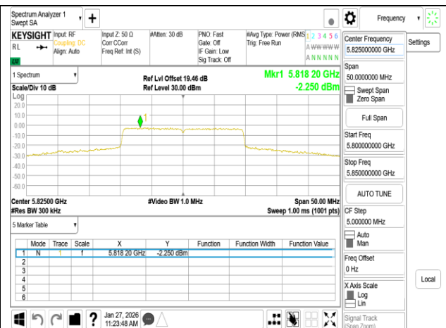
802.11be 20MHz Chain1 5825MHz RU242
