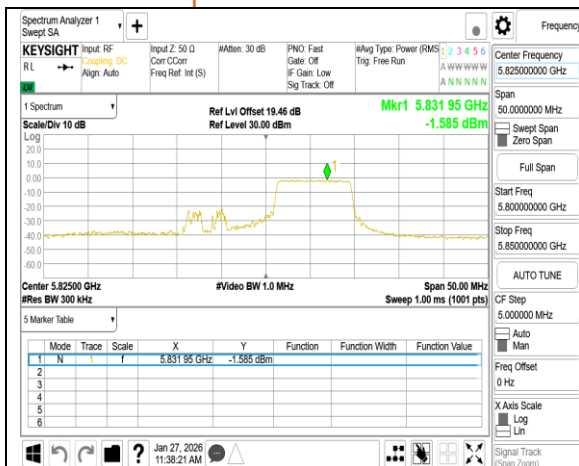
802.11be 20MHz Chain0 5825MHz RU106 54
