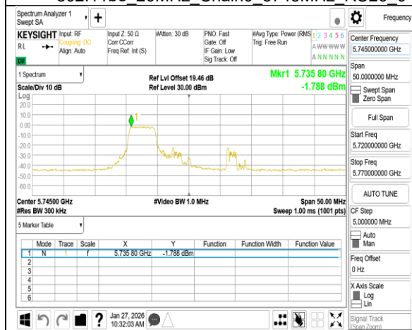
802.11be 20MHz Chain0 5745MHz RU52 37
