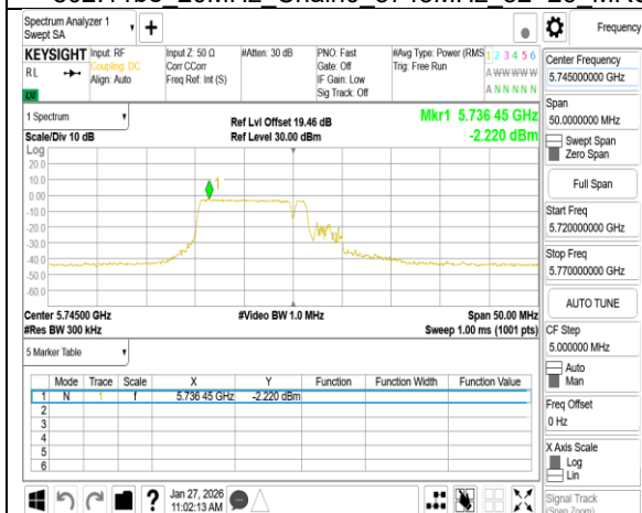
802.11be 20MHz Chain0 5745MHz 106+26 MRU1
