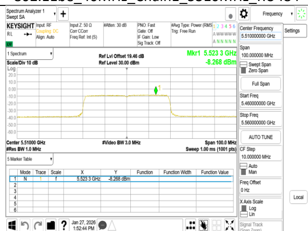
802.11be_40MHz_Chain1_5510MHz_RU484
