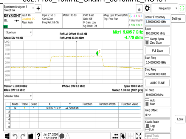
802.11be_40MHz_Chain1_5590MHz_RU484
