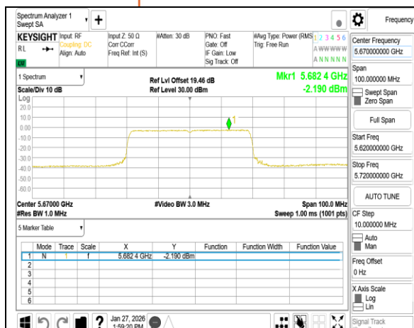
802.11be 40MHz Chain0 5670MHz RU484
