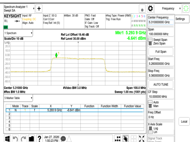
802.11be_40MHz_Chain1_5310MHz_RU484
