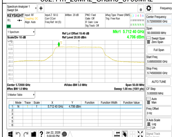
802.11n 20MHz Chain0_5720MHz UNII 2C
