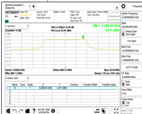
802.11be 20MHz Chain0 5260MHz
