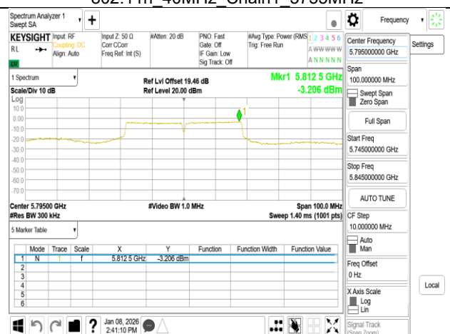
802.11n 40MHz Chain1 5795MHz
