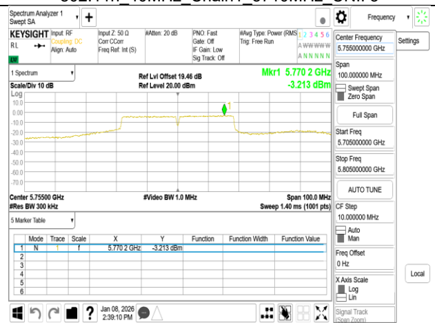
802.11n 40MHz Chain1 5755MHz
