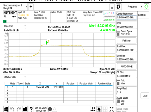
802.11be 20MHz Chain1 5240MHz
