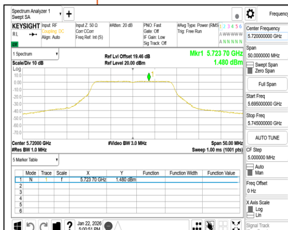
802.11n_20MHz_Chain1_5720MHz_UNII 2C
