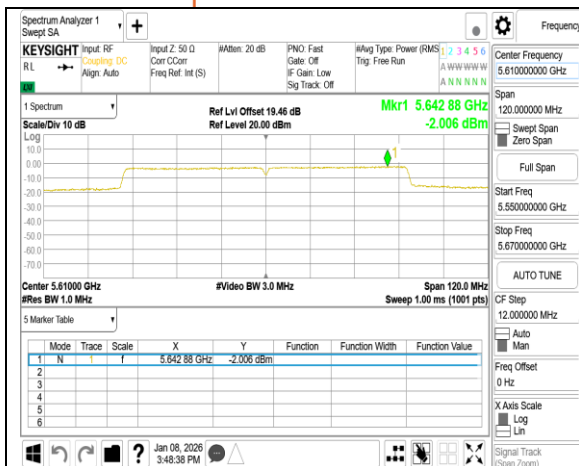
802.11ac 80MHz Chain0 5610MHz
