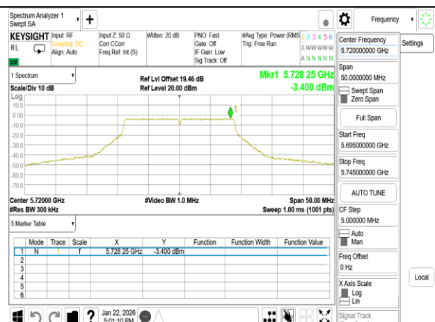
802.11n_20MHz_Chain1_5720MHz_UNII 3
