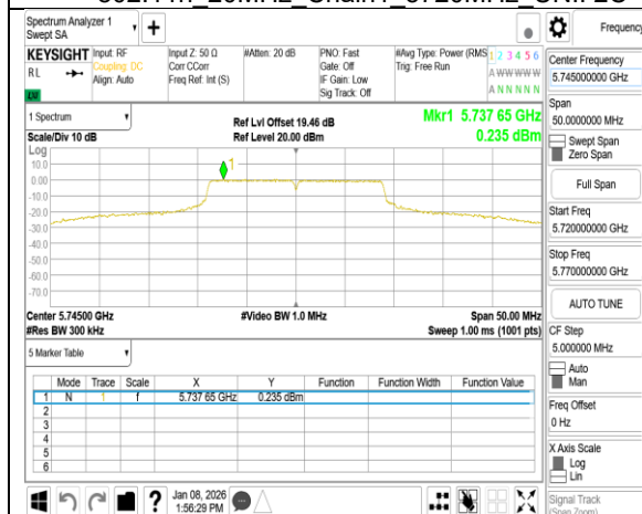
802.11n_20MHz_Chain0_5745MHz
