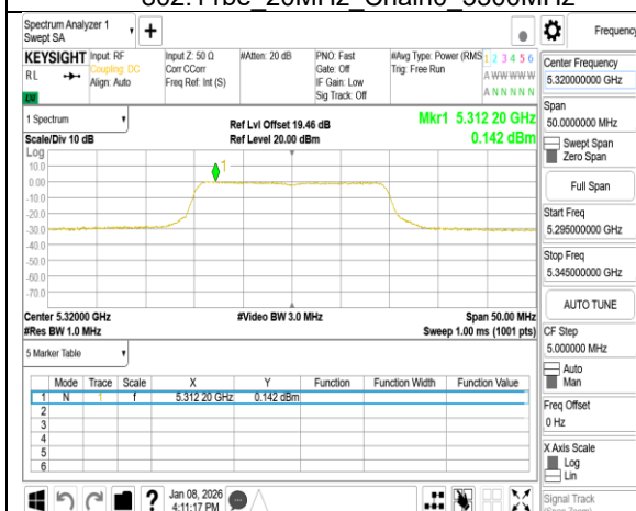
802.11be 20MHz Chain0 5320MHz
