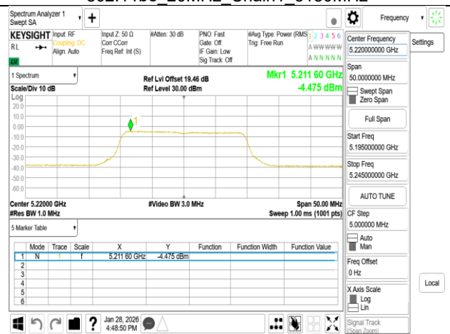
802.11be 20MHz Chain1 5220MHz
