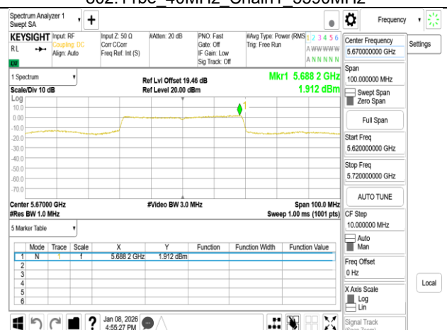
802.11be 40MHz Chain1 5670MHz
