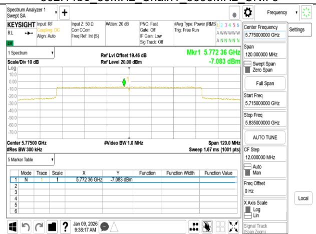
802.11be_80MHz_Chain1_5775MHz
