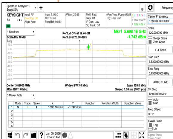
802.11be_80MHz_Chain1_5690MHz_UNII 2C
