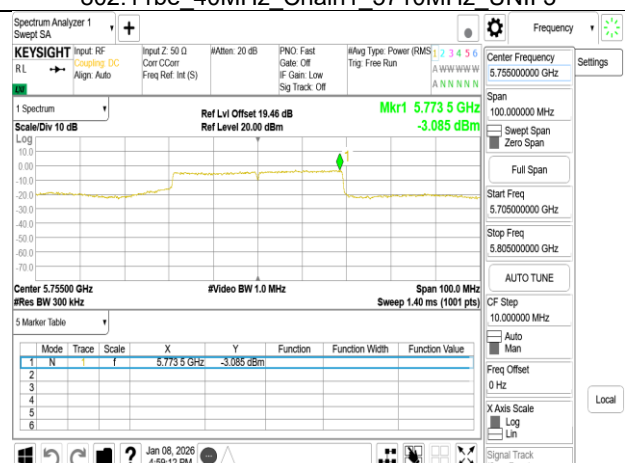
802.11be 40MHz Chain1 5755MHz
