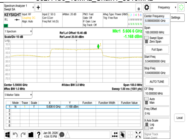
802.11be 40MHz Chain1 5590MHz
