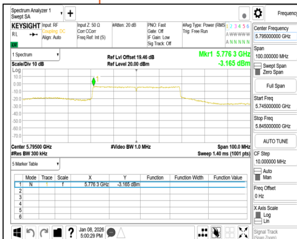
802.11be 40MHz Chain0 5795MHz
