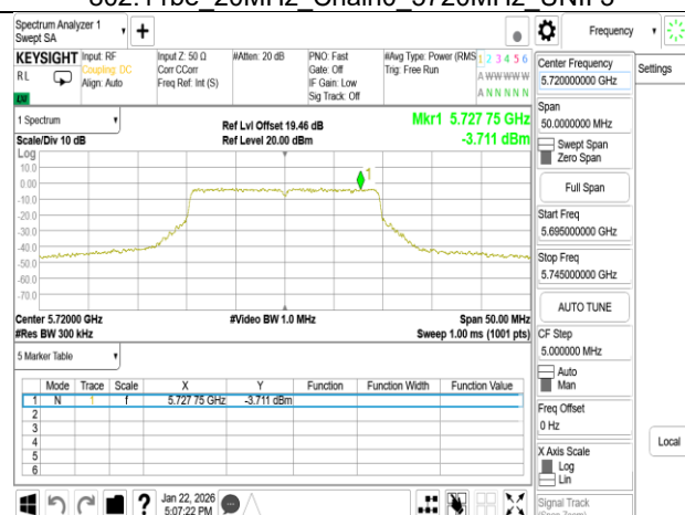
802.11be_20MHz_Chain1_5720MHz_UNII 3
