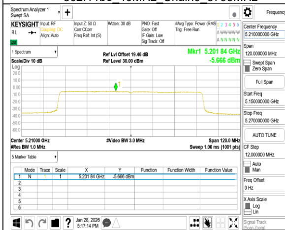
802.11be 80MHz Chain0 5210MHz
