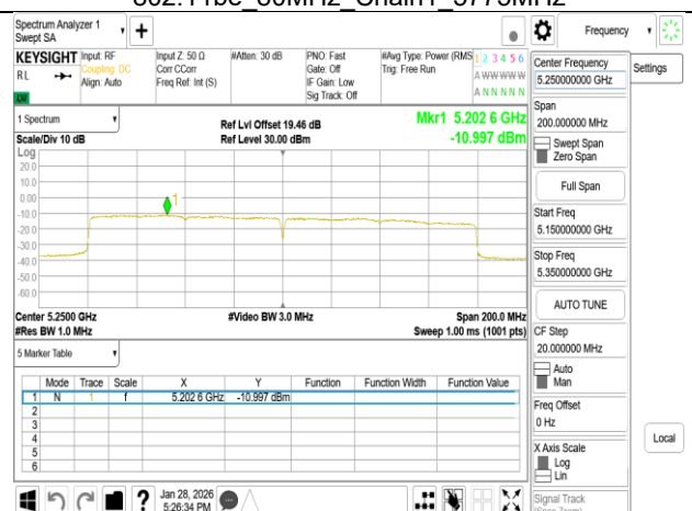
802.11be_160MHz_Chain1_5250MHz
