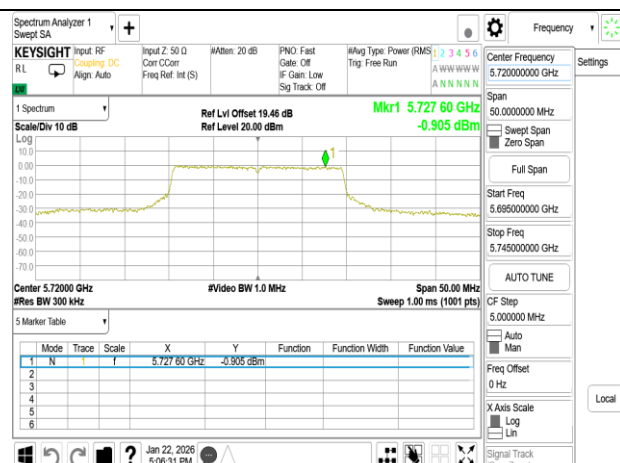
802.11be_20MHz_Chain0_5720MHz_UNII 3
