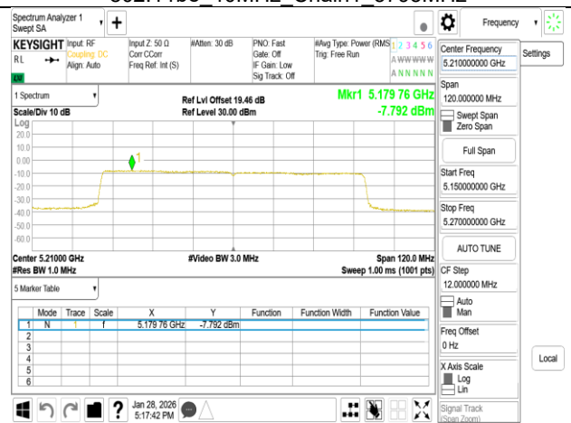
802.11be 80MHz Chain1 5210MHz
