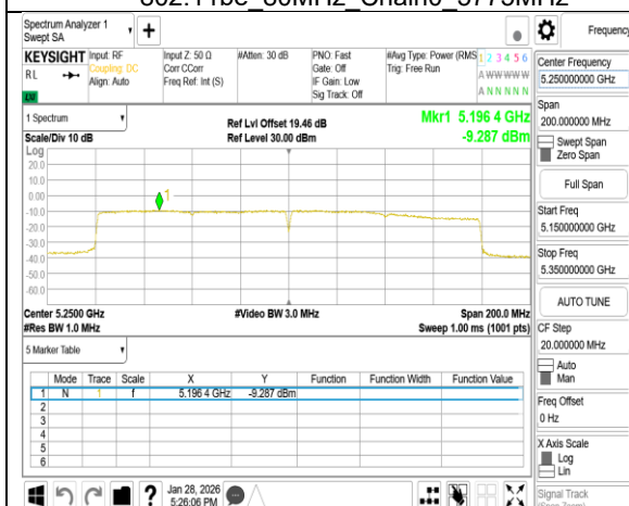
802.11be_160MHz_Chain0_5250MHz
