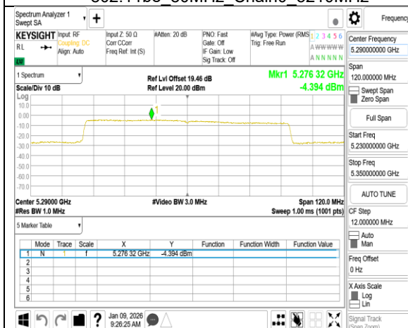
802.11be 80MHz Chain0 5290MHz
