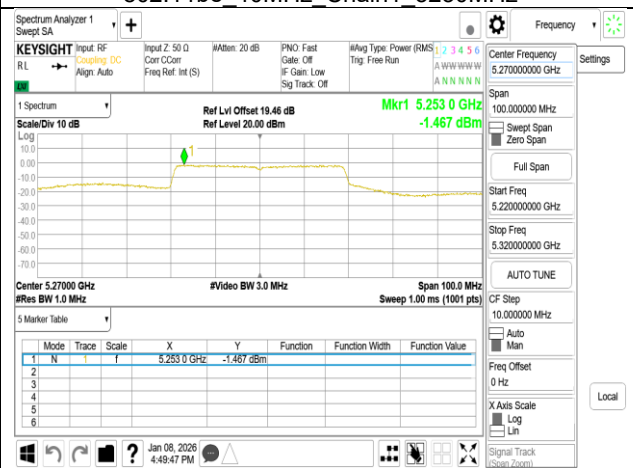
802.11be 40MHz Chain1 5270MHz
