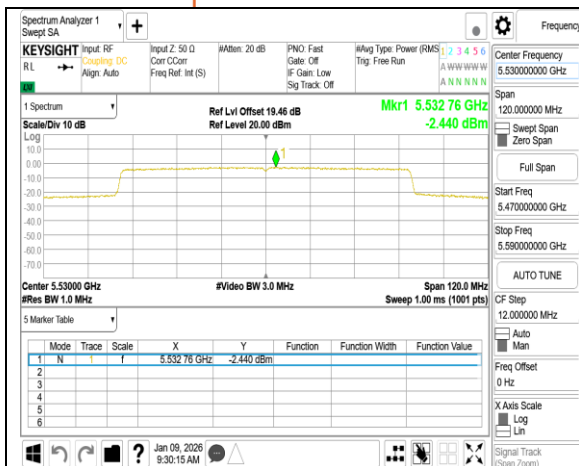
802.11be 80MHz Chain0 5530MHz
