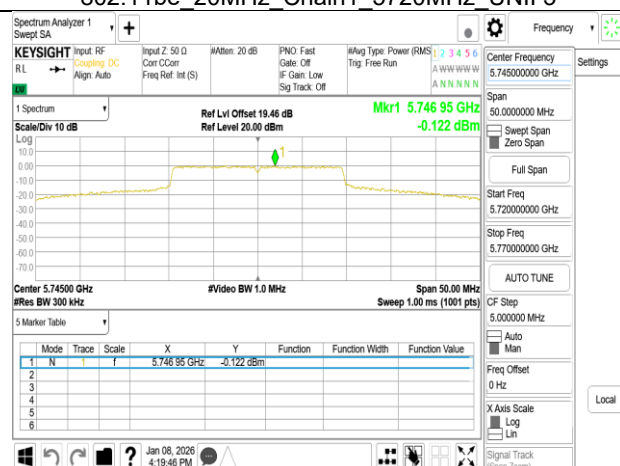
802.11be_20MHz_Chain1_5745MHz
