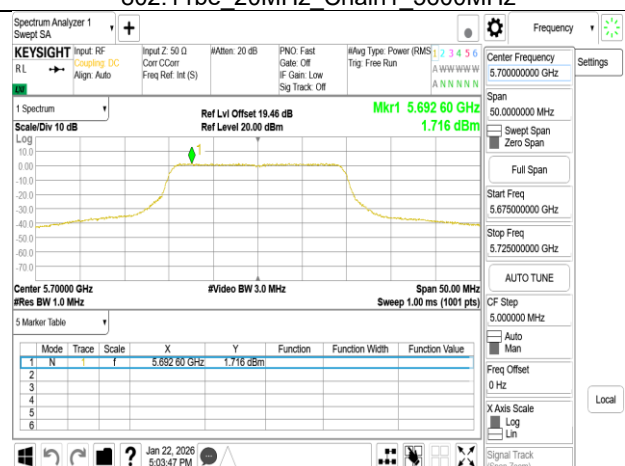
802.11be 20MHz Chain1 5700MHz
