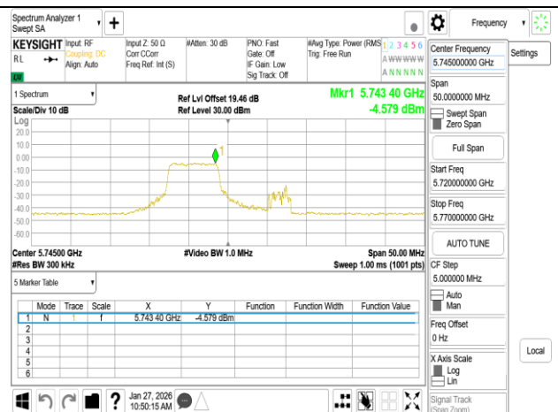
802.11be 20MHz Chain1 5745MHz 52+26 MRU1
