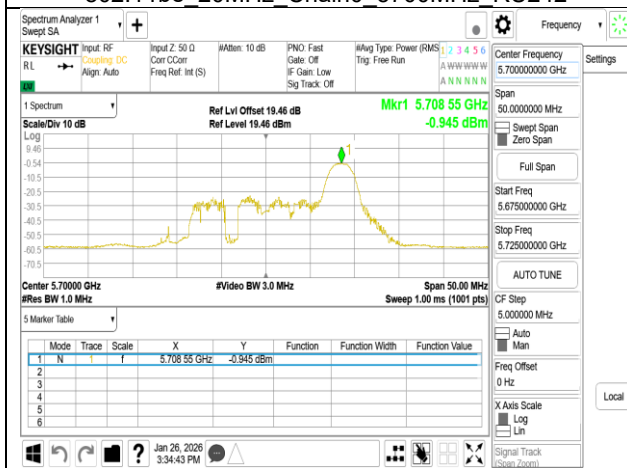
802.11be 20MHz Chain0 5700MHz RU26 8
