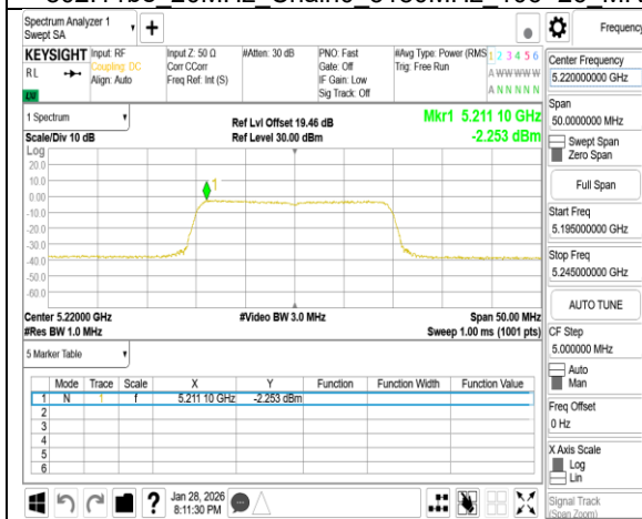
802.11be 20MHz Chain0 5220MHz RU242
