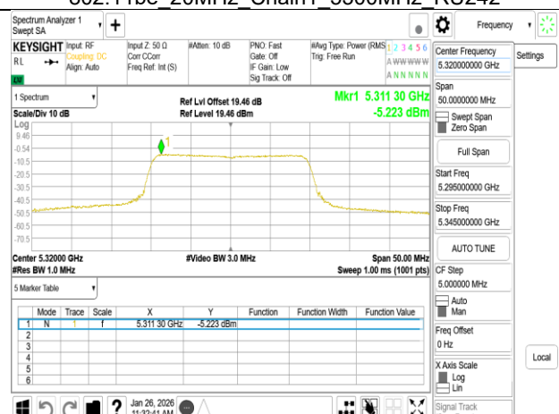
802.11be 20MHz Chain1 5320MHz RU242
