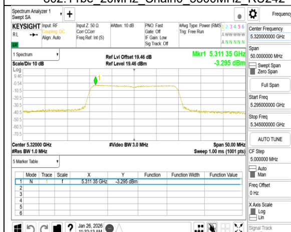
802.11be 20MHz Chain0 5320MHz RU242
