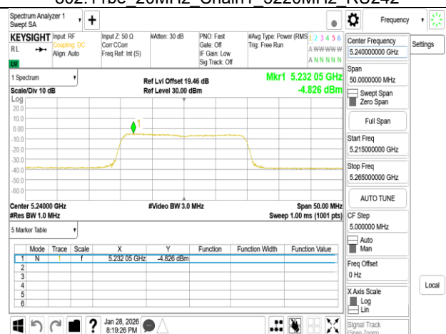
802.11be 20MHz Chain1 5240MHz RU242
