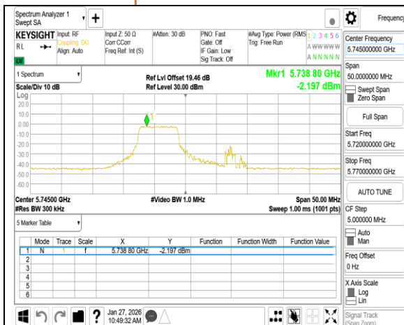
802.11be 20MHz Chain0 5745MHz 52+26 MRU1
