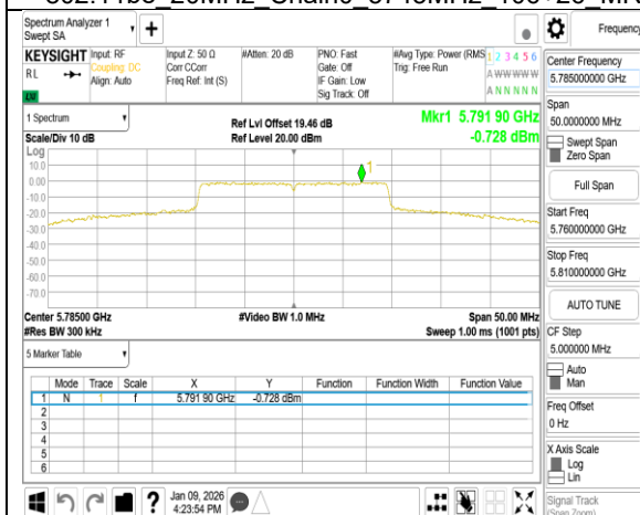
802.11be 20MHz Chain0 5785MHz RU242
