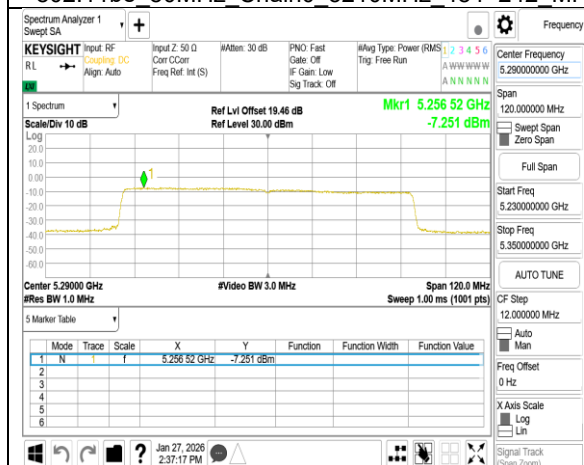
802.11be 80MHz Chain0 5290MHz RU996
