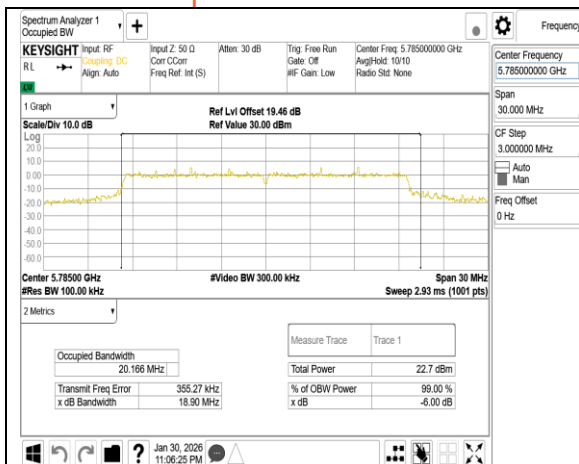
802.11be 20MHz Chain0 5785MHz
