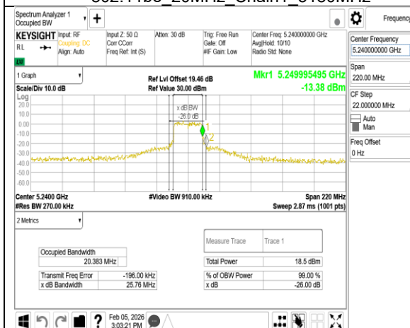
802.11be 20MHz Chain1 5240MHz
