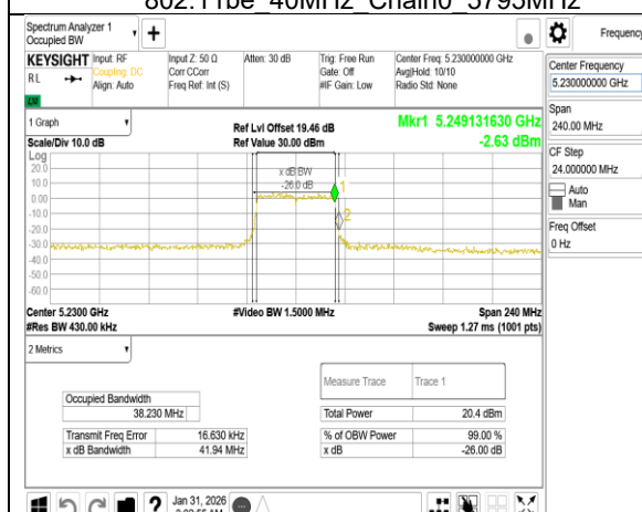
802.11be 40MHz Chain1 5230MHz
