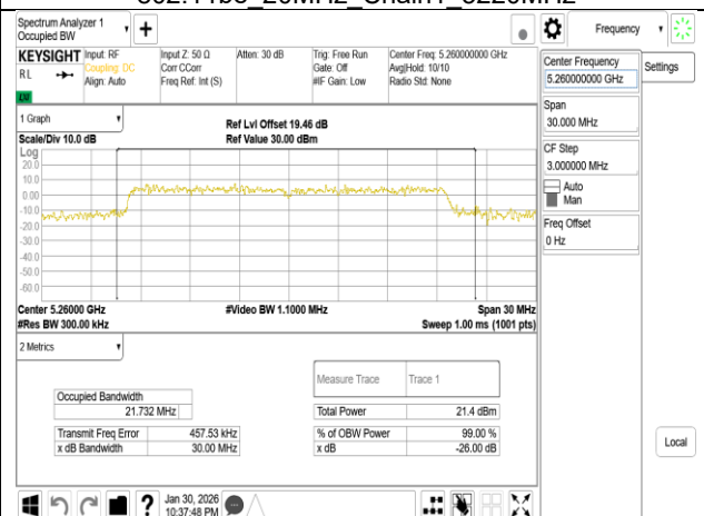
802.11be 20MHz Chain1 5260MHz
