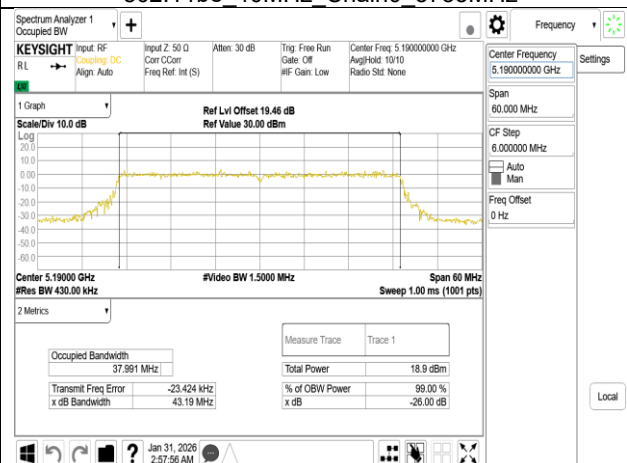
802.11be 40MHz Chain1 5190MHz
