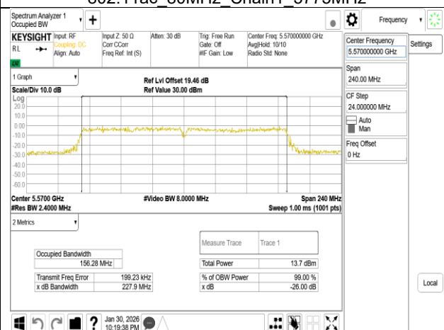
802.11ac 160MHz Chain0 5570MHz
