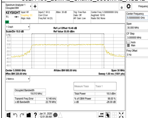
802.11be 20MHz Chain0 5500MHz RU242
