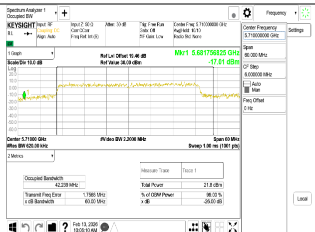
802.11be 40MHz Chain0 5710MHz UNII-2CRU484
