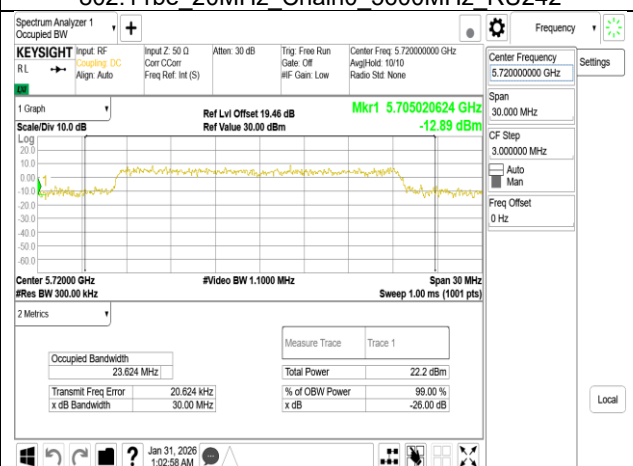
802.11be 20MHz Chain0 5720MHz UNII-2CRU242
