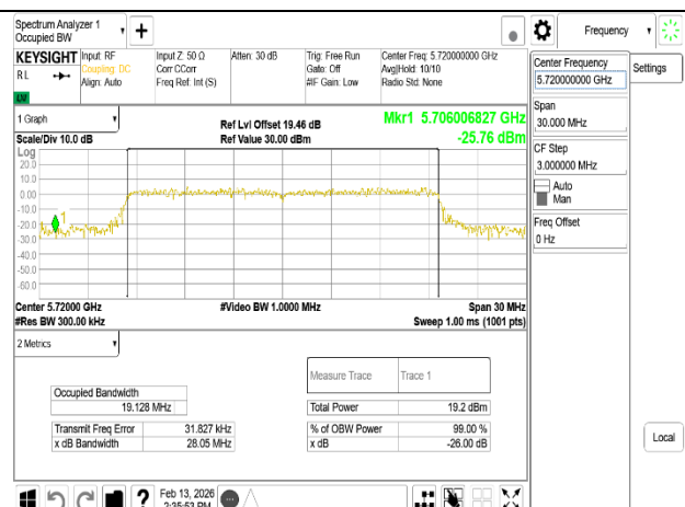
802.11be 20MHz Chain1 5720MHz UNII-2CRU242
