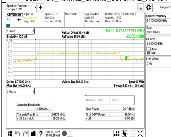
802.11be 40MHz Chain0 5710MHz UNII-3RU484
