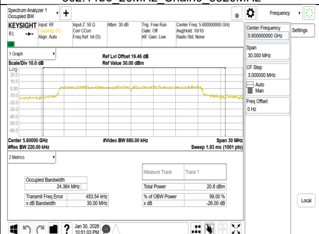
802.11be 20MHz Chain0 5600MHz
