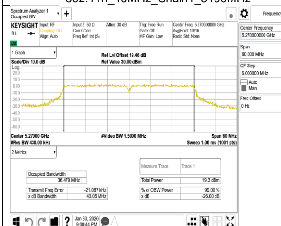
802.11n 40MHz Chain1_5270MHz
