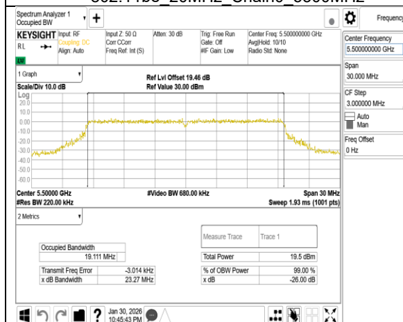
802.11be 20MHz Chain0 5500MHz
