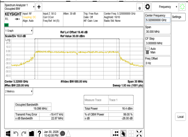
802.11be 20MHz Chain0 5320MHz
