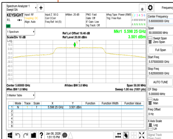
802.11n 20MHz Chain0_5600MHz
