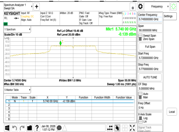
802.11n_20MHz_Chain1_5745MHz
