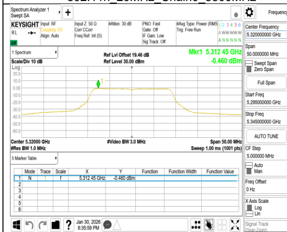
802.11n 20MHz Chain0 5320MHz
