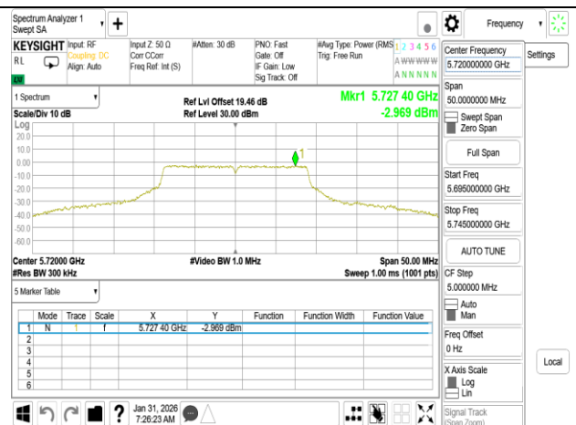
802.11n_20MHz_Chain1_5720MHz_UNII 3
