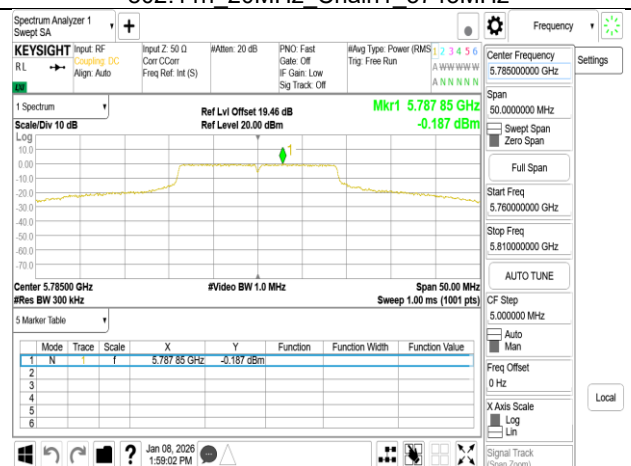
802.11n_20MHz_Chain1_5785MHz
