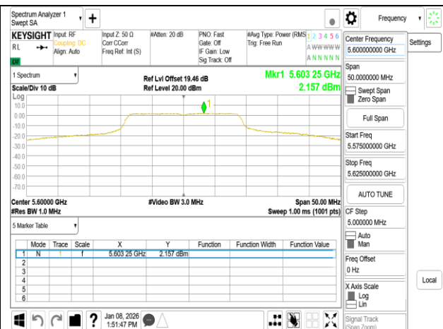
802.11n 20MHz Chain1_5600MHz
