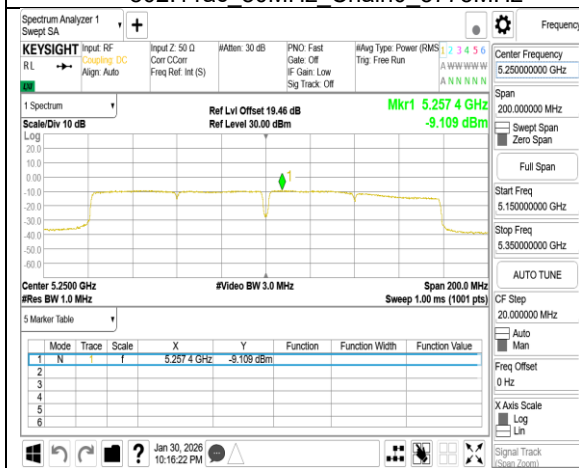
802.11ac 160MHz Chain0 5250MHz
