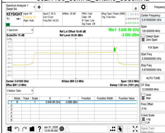
802.11be 80MHz Chain0 5610MHz
