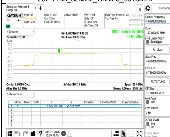
802.11be 80MHz Chain0 5690MHz UNII 2C
