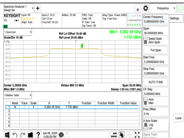
802.11be_20MHz_Chain1_5260MHz
