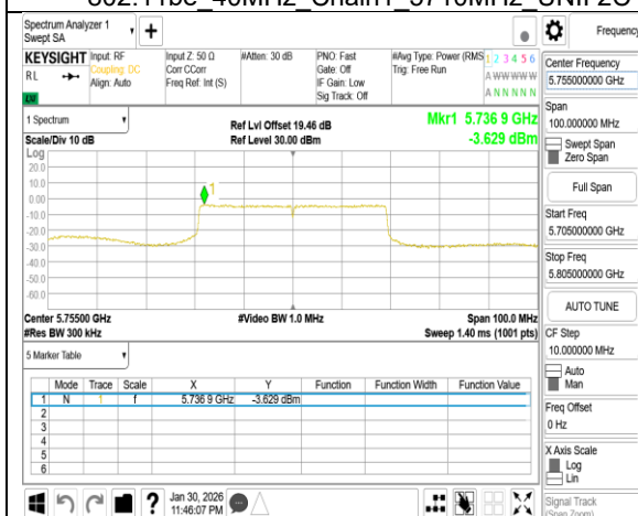
802.11be 40MHz Chain0 5755MHz
