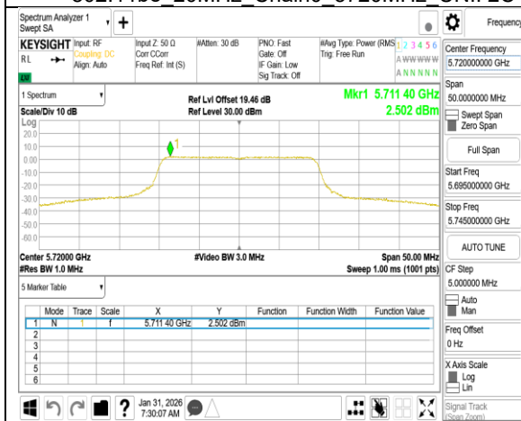
802.11be_20MHz_Chain1_5720MHz_UNII 2C
