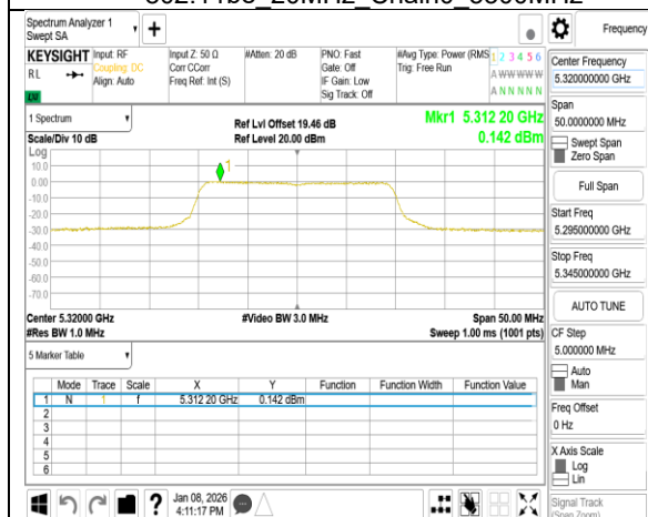
802.11be_20MHz_Chain0_5320MHz
