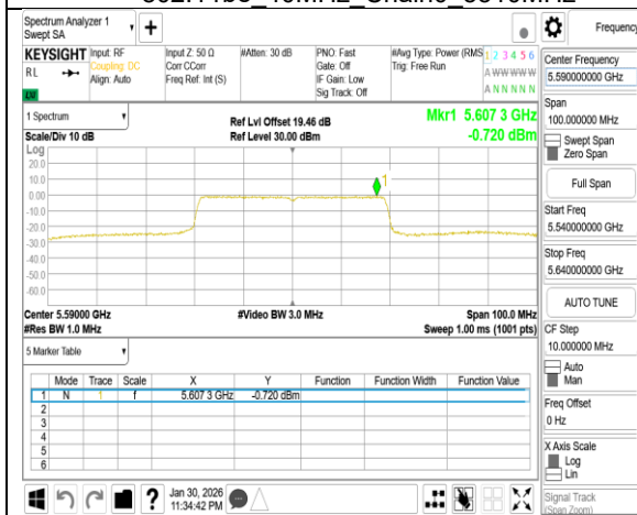
802.11be 40MHz Chain0 5590MHz
