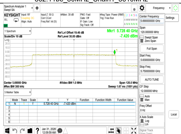
802.11be 80MHz Chain0 5690MHz UNII 3
