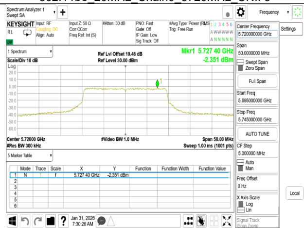
802.11be_20MHz_Chain1_5720MHz_UNII 3
