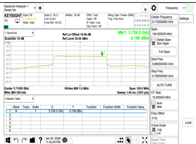
802.11be 40MHz Chain0 5710MHz UNII 3
