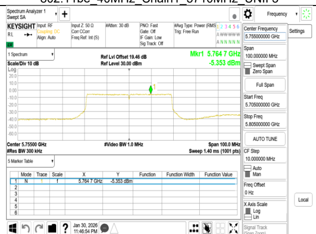
802.11be 40MHz Chain1 5755MHz
