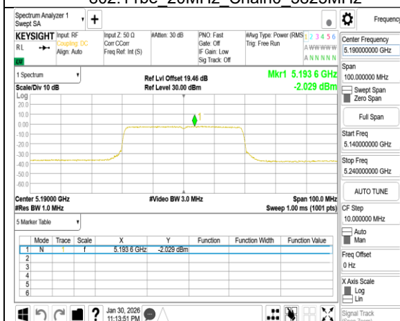
802.11be 40MHz Chain0 5190MHz
