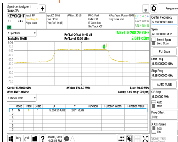
802.11be_20MHz_Chain0_5260MHz
