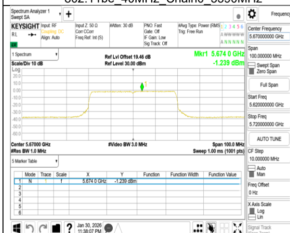
802.11be 40MHz Chain0 5670MHz
