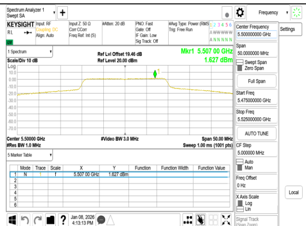
802.11be 20MHz Chain1 5500MHz
