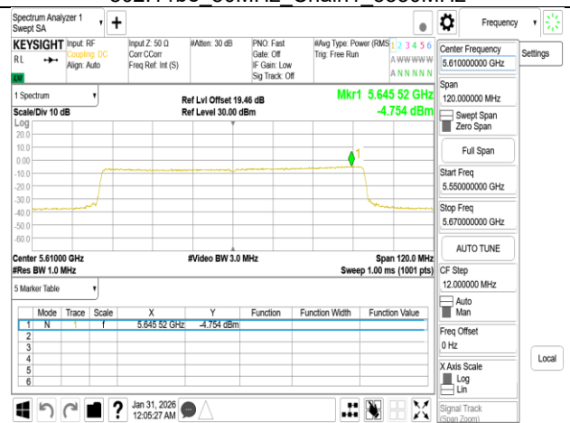
802.11be 80MHz Chain1 5610MHz
