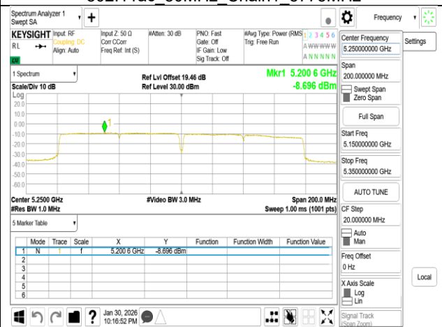
802.11ac 160MHz Chain1 5250MHz
