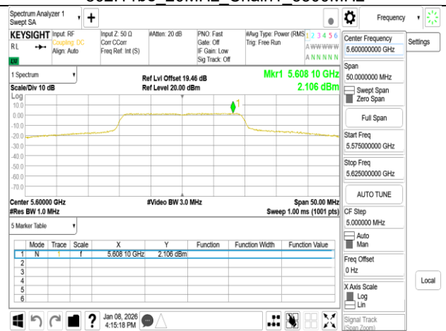
802.11be 20MHz Chain1 5600MHz
