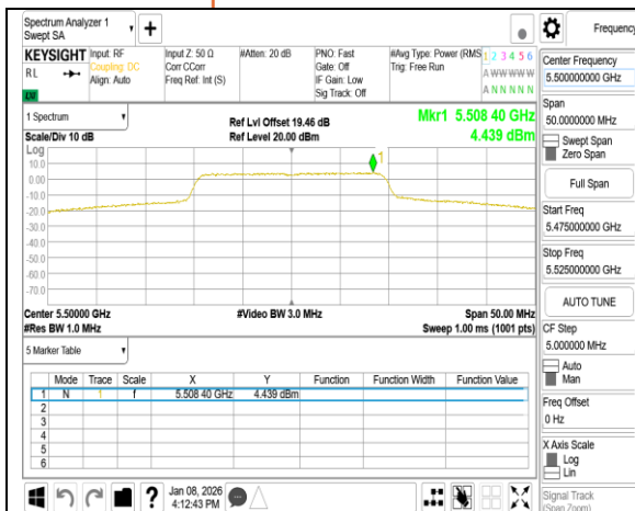
802.11be 20MHz Chain0 5500MHz
