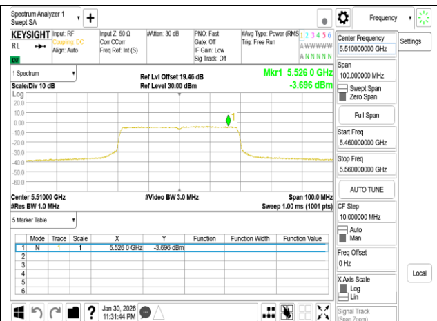
802.11be 40MHz Chain1 5510MHz
