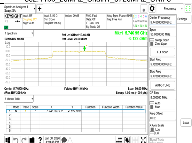
802.11be_20MHz_Chain1_5745MHz
