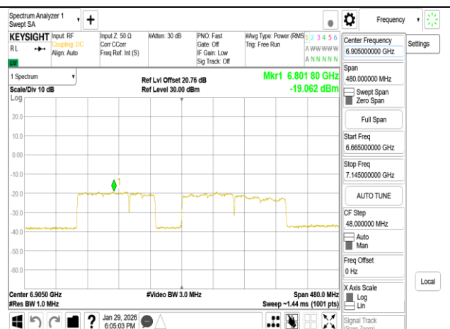
802.11be_320MHz_Chain1_6905MHz_3x996+484_MR4
