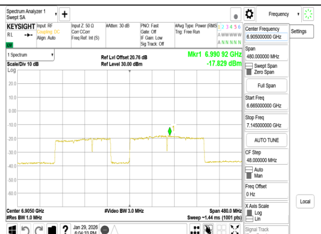
802.11be 320MHz Chain0 6905MHz 3x996+484 MRU4
