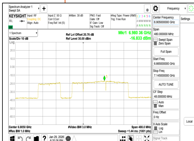
802.11be 320MHz Chain0 6905MHz 3x996+484 MRU3
