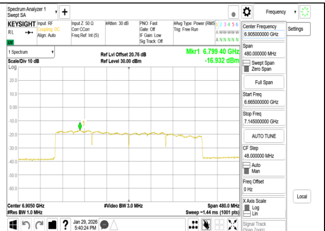
802.11be 320MHz Chain1 6905MHz RU996x4
