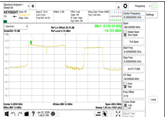
802.11be 320MHz Chain1 6265MHz 3x996 MRU3
