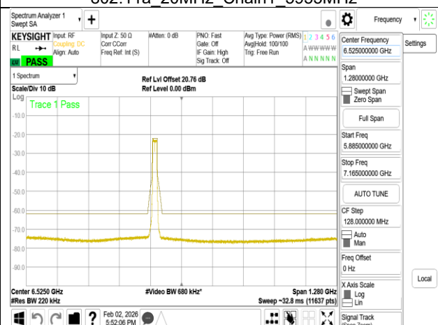
802.11a 20MHz Chain1 6415MHz
