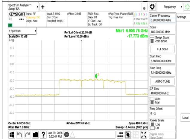
802.11be 320MHz Chain1 6905MHz 3x996 MRU1
