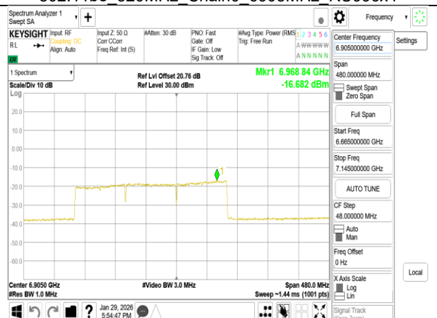
802.11be 320MHz Chain0 6905MHz 3x996 MRU4
