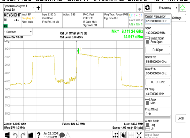
802.11be 320MHz Chain1 6105MHz 3x996 MRU2
