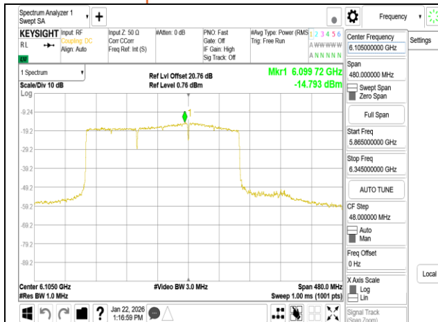
802.11be 320MHz Chain1 6105MHz 3x996 MRU4
