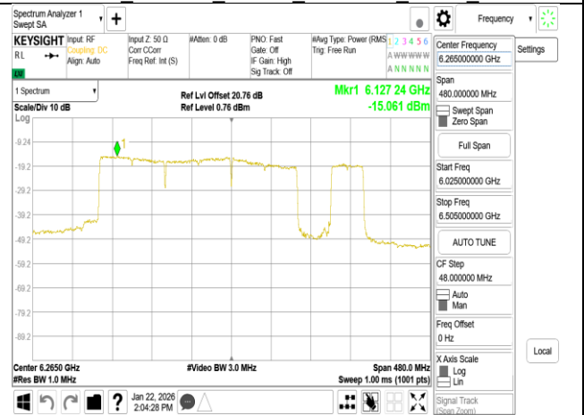
802.11be 320MHz Chain1 6265MHz 3x996+484 MRU7
