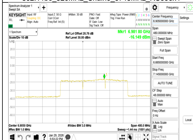
802.11be 320MHz Chain0 6905MHz 3x996 MRU1
