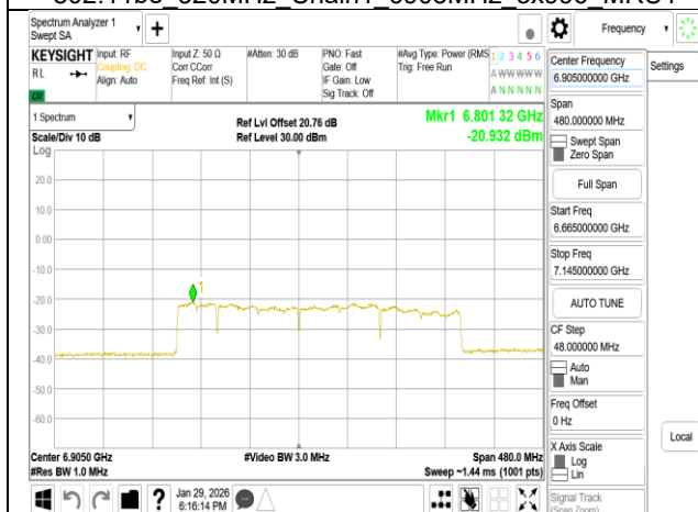
802.11be 320MHz Chain1 6905MHz 3x996+484 MRU1
