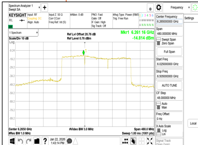
802.11be 320MHz Chain1 6265MHz 3x996 MRU1
