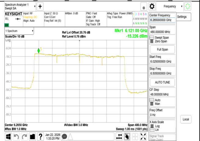
802.11be 320MHz Chain1 6265MHz RU996x4
