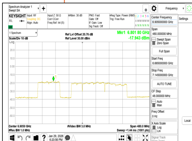
802.11be_320MHz_Chain1_6905MHz_3x996+484_MR3
