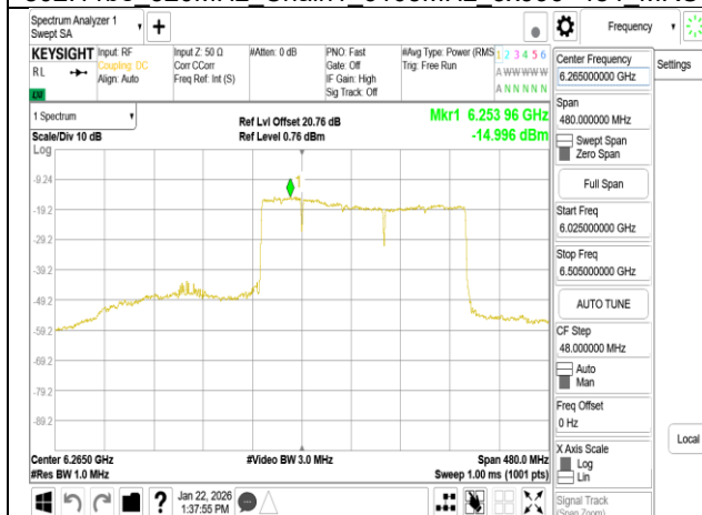
802.11be 320MHz Chain1 6265MHz 2x996+484 MRU7
