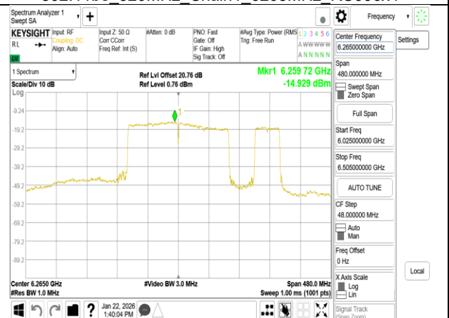
802.11be 320MHz Chain1 6265MHz 2x996+484 MRU11
