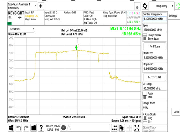
802.11be 320MHz Chain1 6105MHz 3x996+484 MRU8
