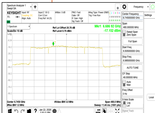
802.11be 320MHz Chain0 6745MHz RU996x4
