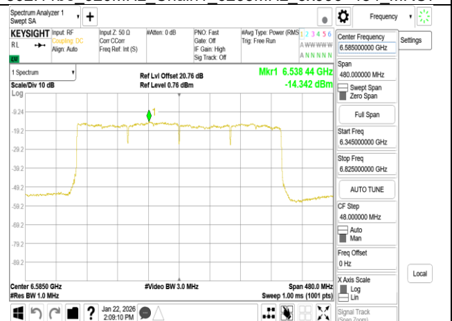
802.11be 320MHz Chain1 6585MHz RU996x4
