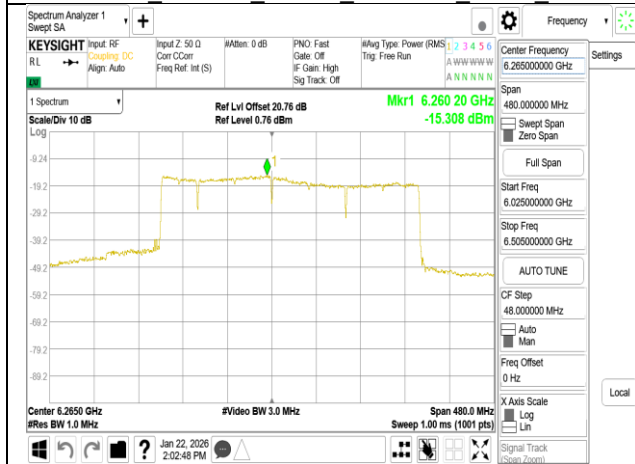
802.11be 320MHz Chain1 6265MHz 3x996+484 MRU1
