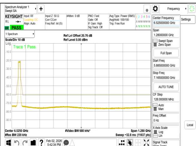
802.11a 20MHz Chain1 5955MHz
