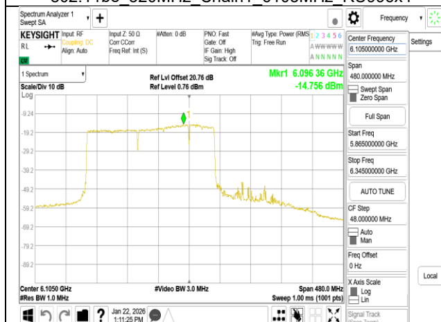
802.11be 320MHz Chain1 6105MHz 2x996+484 MRU6
