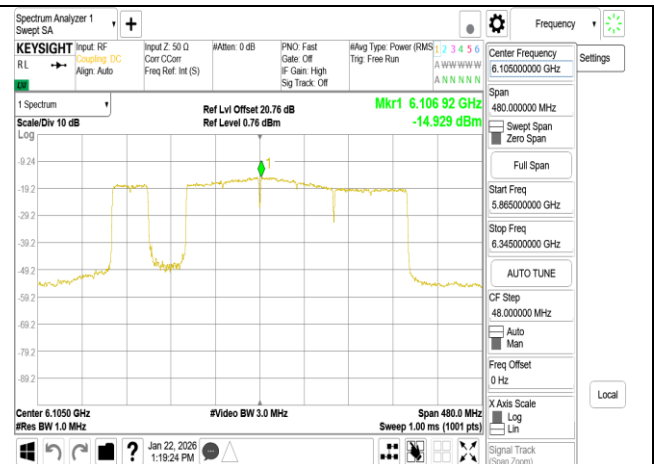
802.11be 320MHz Chain1 6105MHz 3x996+484 MRU2
