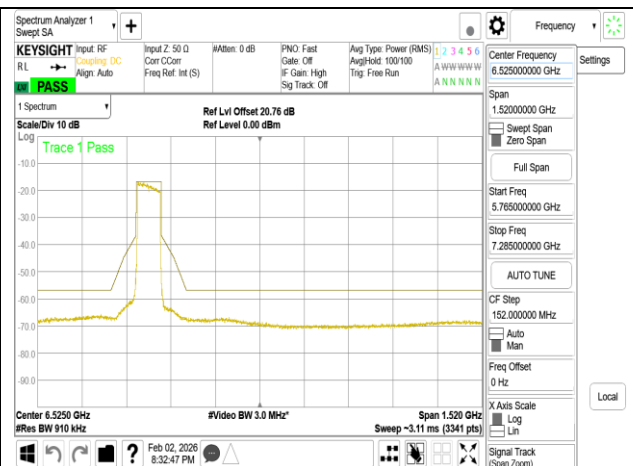
802.11be_80MHz_Chain0_6145MHz
