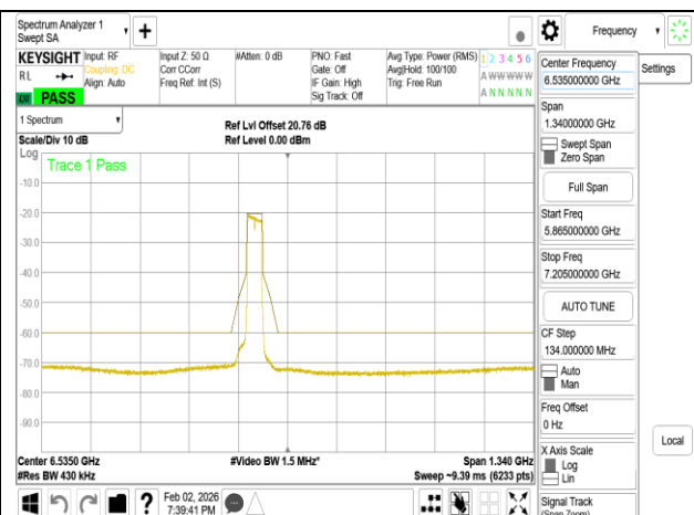
802.11be 40MHz Chain0 6445MHz
