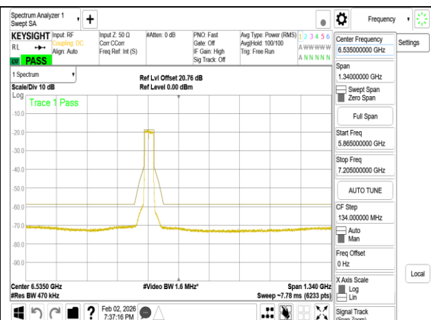
802.11be 40MHz Chain1 6405MHz
