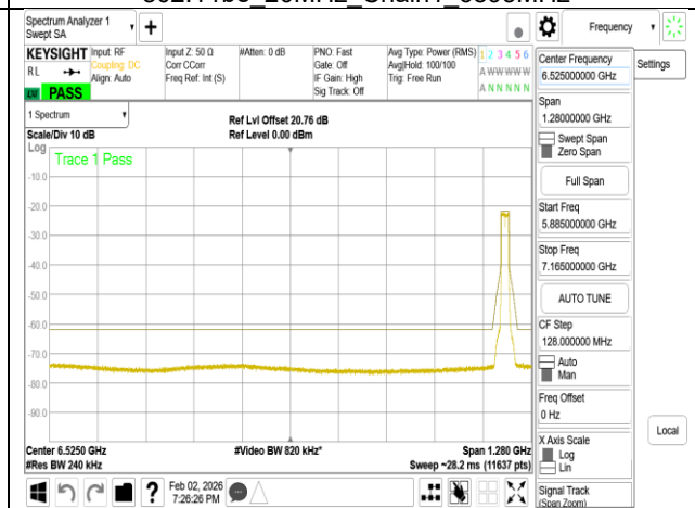
802.11be_20MHz_Chain1_7095MHz
