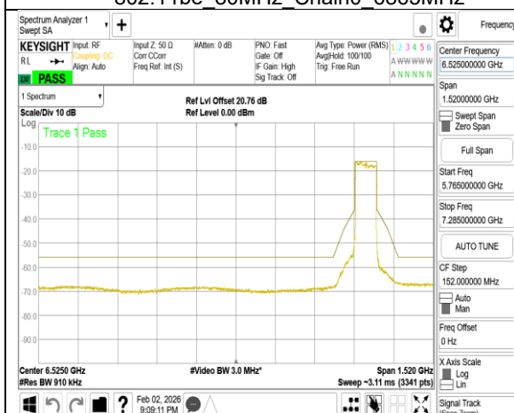
802.11be_80MHz_Chain0_7025MHz
