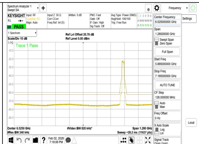
802.11be_20MHz_Chain1_6895MHz
