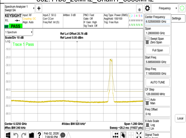
802.11be_20MHz_Chain1_6855MHz
