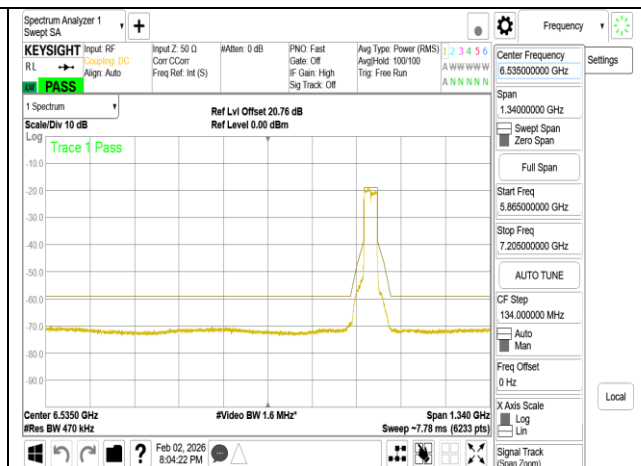
802.11be 40MHz Chain1 685MHz
