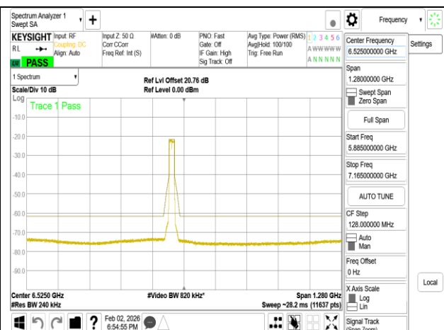
802.11be_20MHz_Chain1_6475MHz
