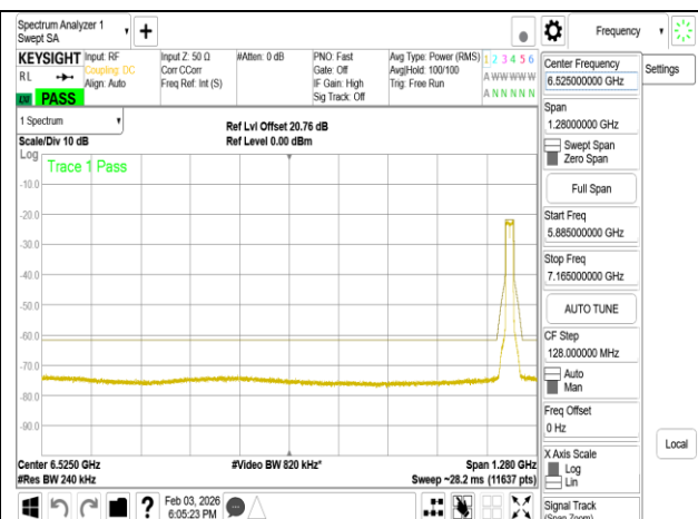
802.11be 20MHz Chain1 7095MHz RU242
