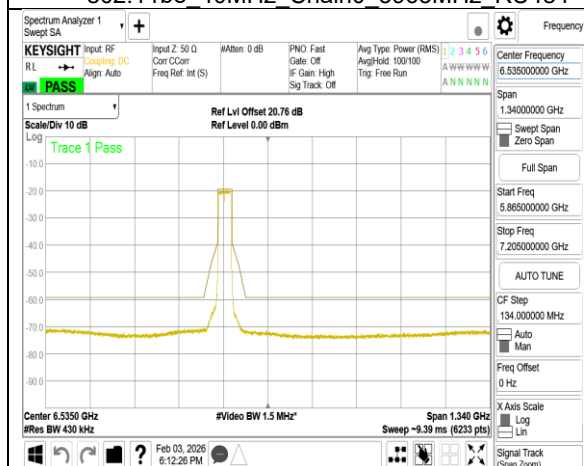
802.11be 40MHz Chain0 6405MHz RU484
