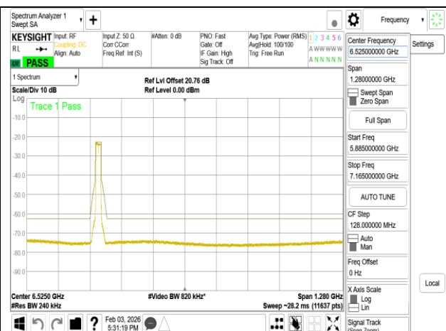
802.11be 20MHz Chain0 6175MHz RU242
