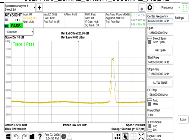
802.11be 20MHz Chain1 6855MHz RU242
