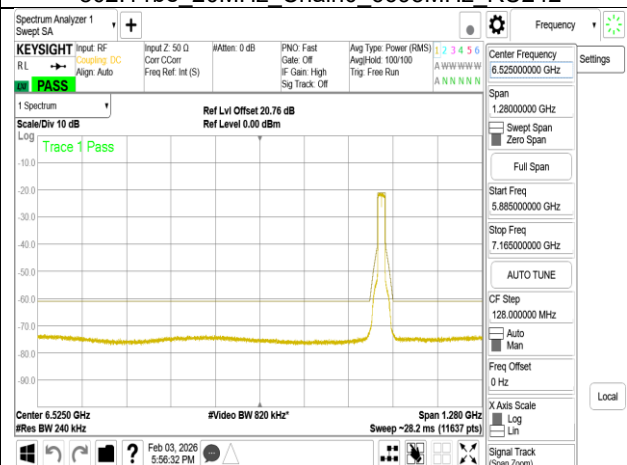
802.11be 20MHz Chain0 6875MHz RU242
