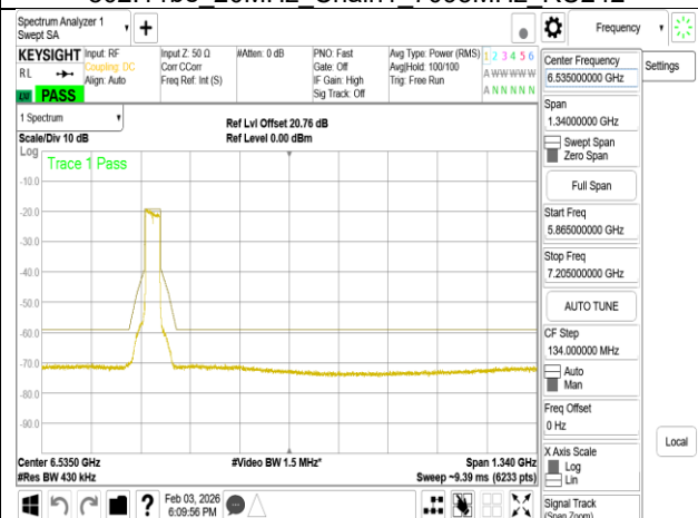
802.11be 40MHz Chain0 6165MHz RU484
