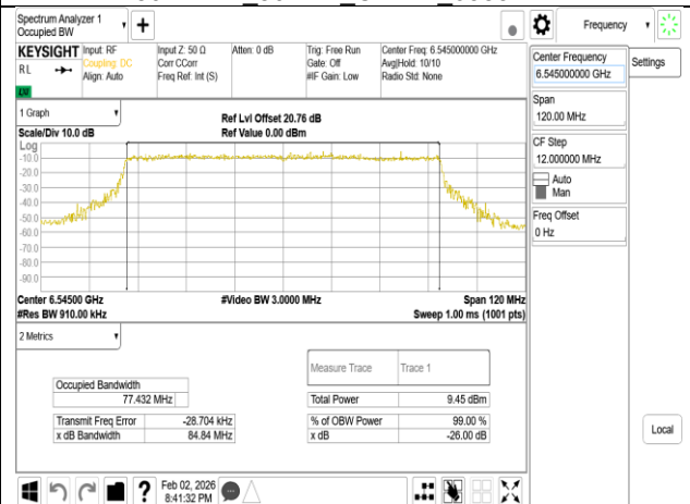
802.11be_80MHz_Chain1_6545MHz
