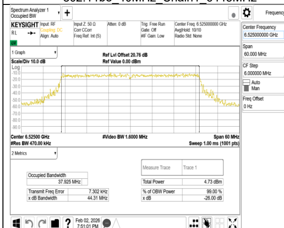
802.11be 40MHz Chain1 6525MHz
