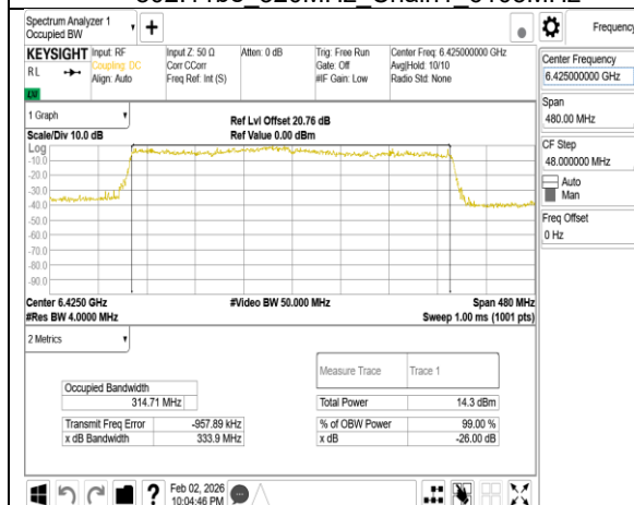
802.11be 320MHz Chain1 6425MHz
