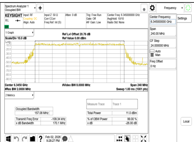
802.11be_160MHz_Chain1_6345MHz
