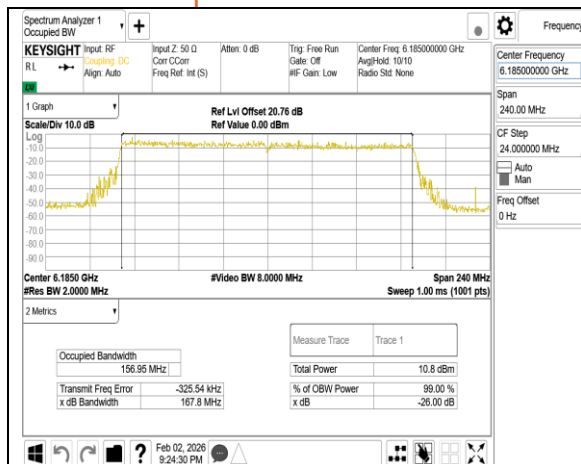
802.11be_160MHz_Chain1_6185MHz
