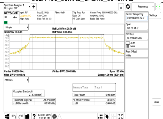
802.11be_80MHz_Chain1_5985MHz
