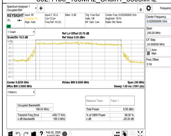
802.11be_160MHz_Chain1_6825MHz
