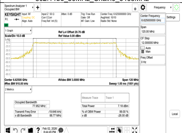
802.11be_80MHz_Chain0_6625MHz
