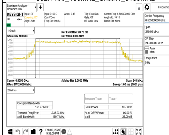
802.11be_160MHz_Chain1_6505MHz
