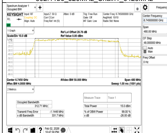
802.11be 320MHz Chain1 6745MHz
