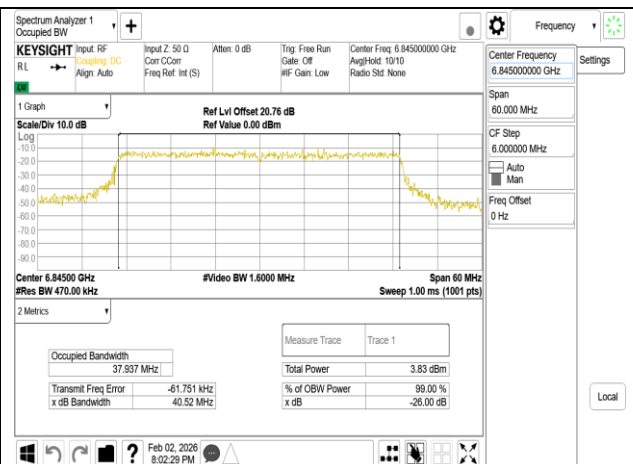
802.11be 40MHz Chain1 6845MHz
