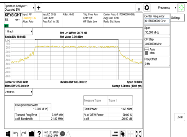
802.11be 20MHz Chain0 6175MHz RU242
