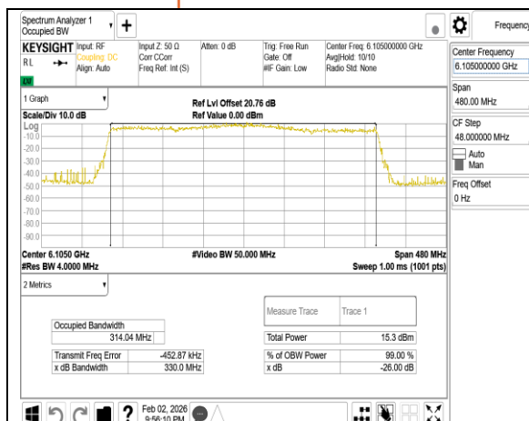
802.11be 320MHz Chain1 6105MHz
