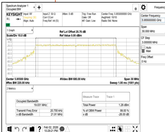
802.11be 20MHz Chain0 5955MHz RU242
