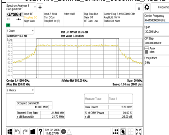
802.11be 20MHz Chain0 6415MHz RU242
