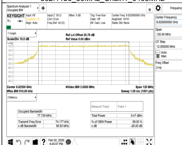
802.11be_80MHz_Chain1_6625MHz
