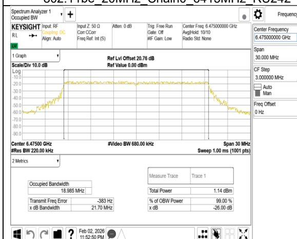
802.11be 20MHz Chain0 6475MHz RU242
