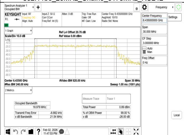
802.11be 20MHz Chain0 6435MHz RU242
