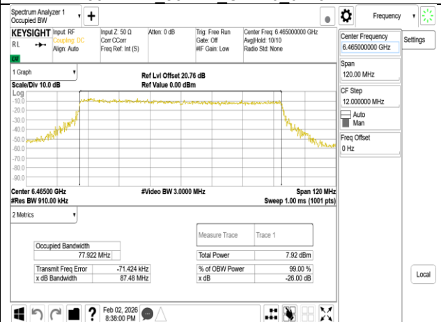
802.11be_80MHz_Chain0_6465MHz
