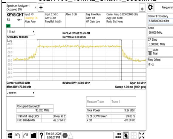
802.11be 40MHz Chain1 6885MHz
