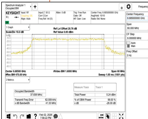
802.11be 40MHz Chain1 6685MHz
