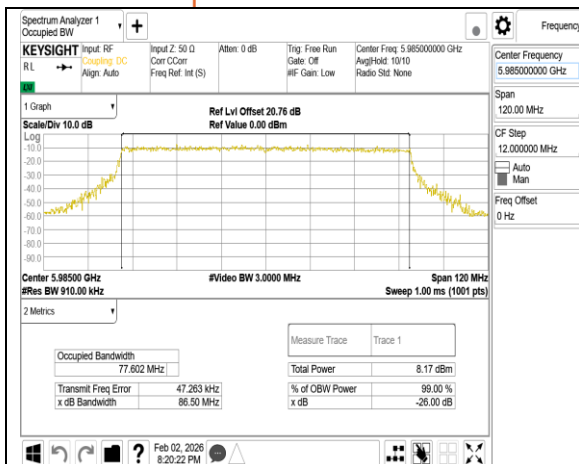
802.11be_80MHz_Chain0_5985MHz
