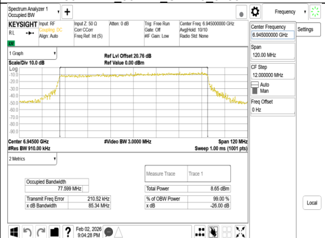
802.11be_80MHz_Chain0_6945MHz
