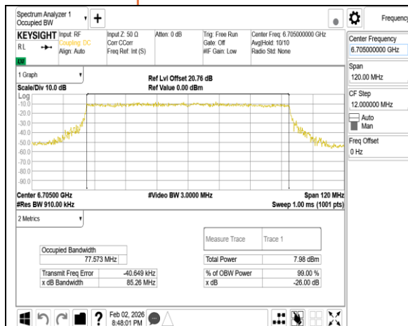
802.11be_80MHz_Chain0_6705MHz
