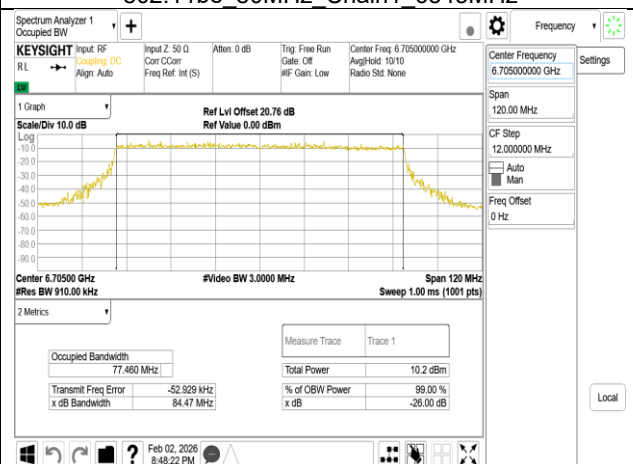
802.11be_80MHz_Chain1_6705MHz
