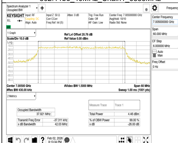
802.11be 40MHz Chain1 7005MHz
