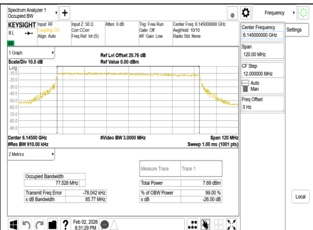
802.11be_80MHz_Chain0_6145MHz
