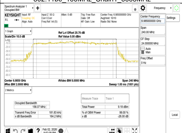
802.11be_160MHz_Chain1_6985MHz
