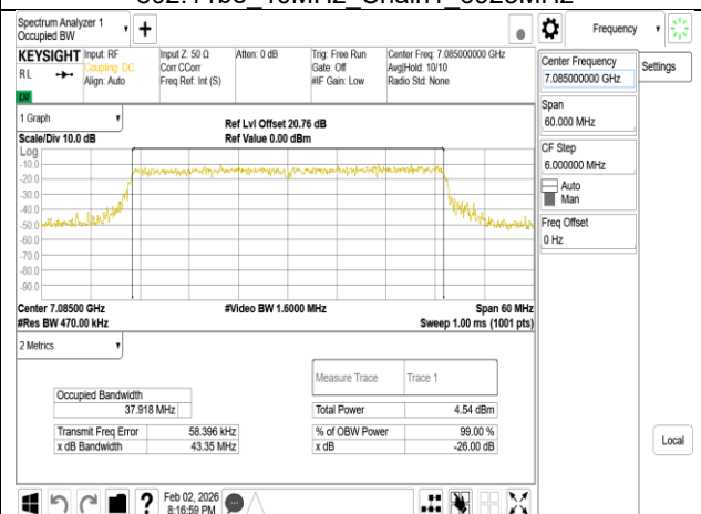
802.11be 40MHz Chain1 7085MHz
