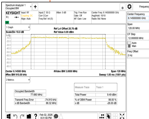
802.11be_80MHz_Chain1_6145MHz
