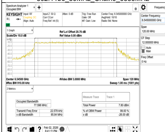
802.11be_80MHz_Chain0_6545MHz
