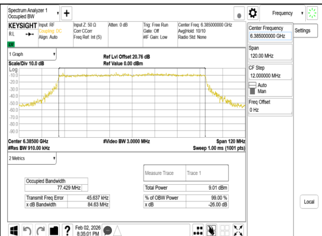
802.11be_80MHz_Chain1_6385MHz
