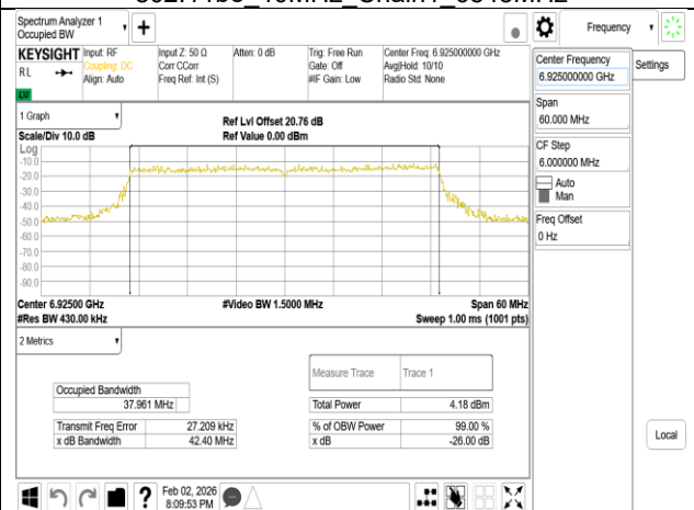
802.11be 40MHz Chain1 6925MHz
