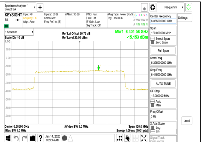
802.11be 80MHz Chain1 6385MHz
