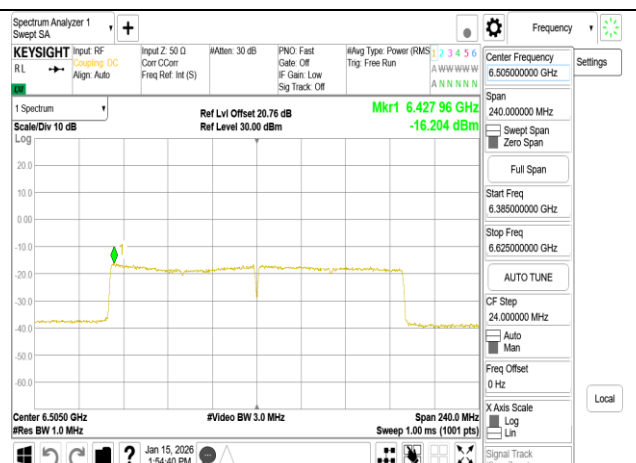
802.11be_160MHz_Chain0_6505MHz
