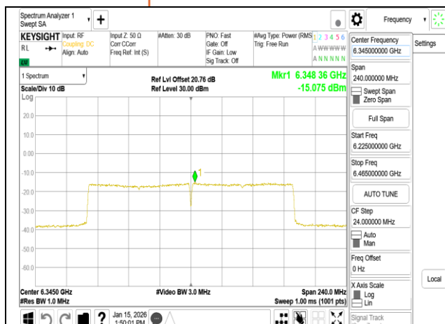
802.11be_160MHz_Chain0_6345MHz
