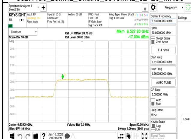
802.11be 20MHz Chain0 6535MHz RU242
