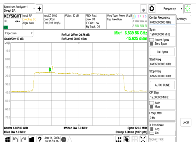
802.11be 80MHz Chain1 6865MHz
