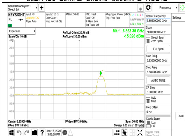
802.11be 20MHz Chain0 6855MHz RU26 8
