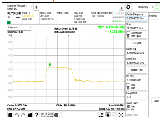
802.11be 20MHz Chain0 6435MHz 106+26 MRU1
