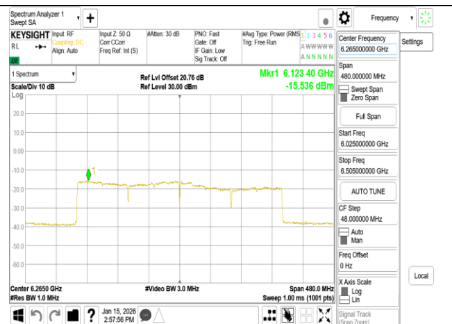
802.11be 320MHz Chain1_6265MHz
