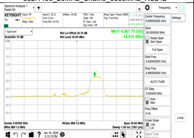
802.11be 20MHz Chain0 6855MHz RU52 40
