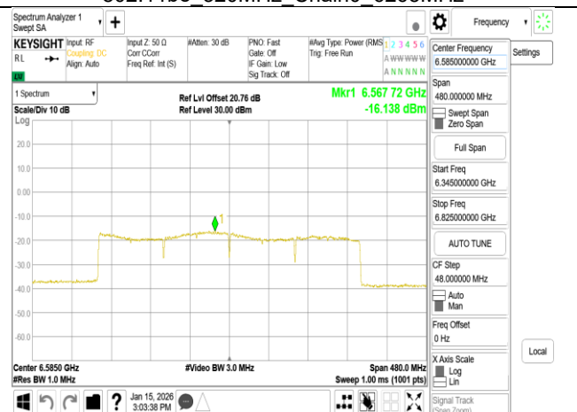
802.11be_320MHz_Chain0_6585MHz
