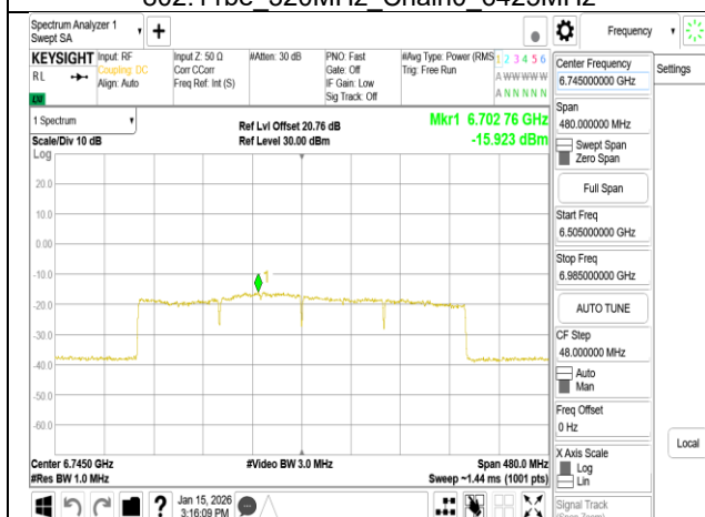
802.11be_320MHz_Chain0_6745MHz
