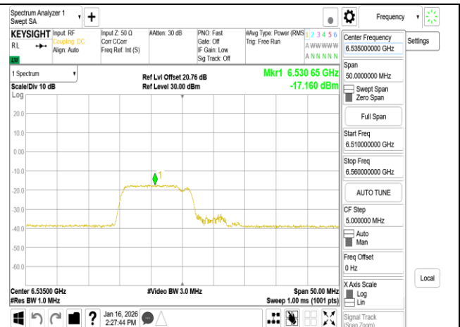
802.11be 20MHz Chain0 6535MHz 106+26 MRU1
