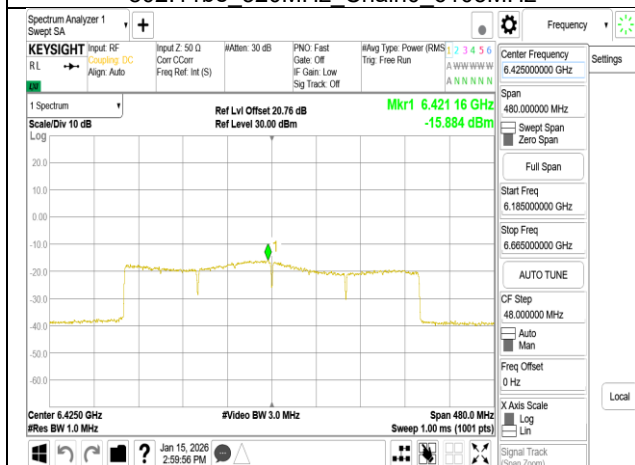
802.11be_320MHz_Chain0_6425MHz
