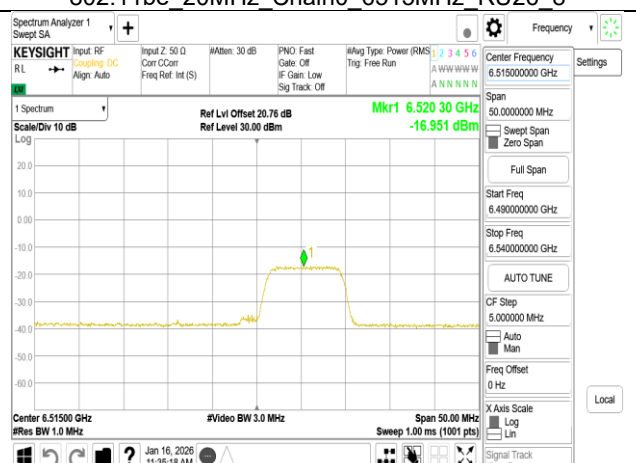
802.11be 20MHz Chain0 6515MHz RU106_54
