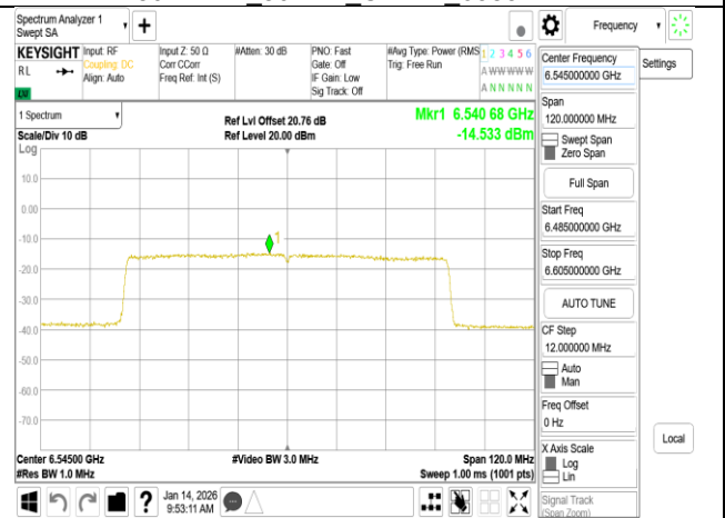
802.11be 80MHz Chain1 6545MHz
