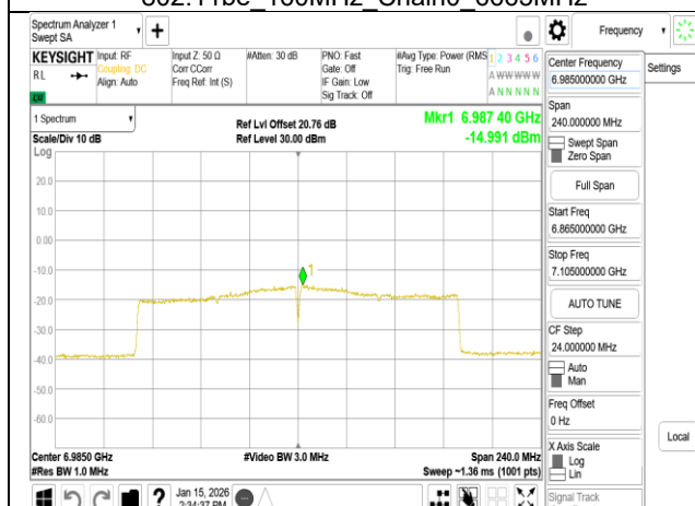
802.11be_160MHz_Chain0_6985MHz
