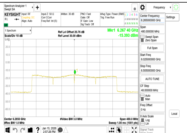
802.11be_320MHz_Chain0_6265MHz
