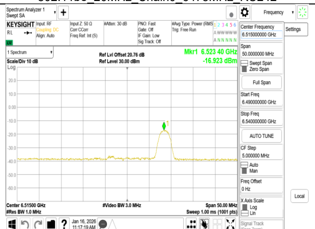
802.11be 20MHz Chain0 6515MHz RU26_8
