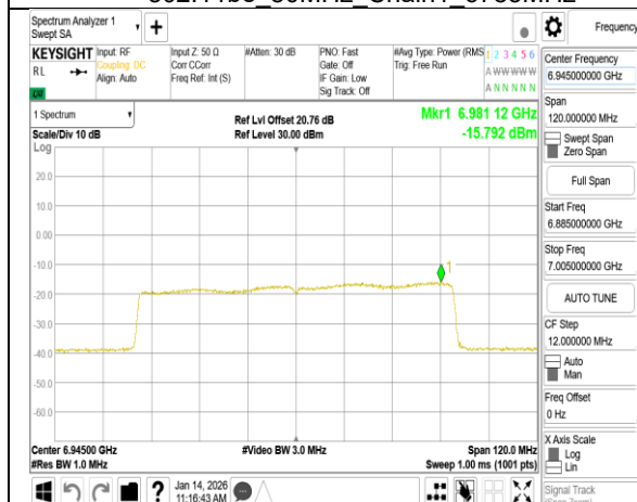
802.11be 80MHz Chain1 6945MHz
