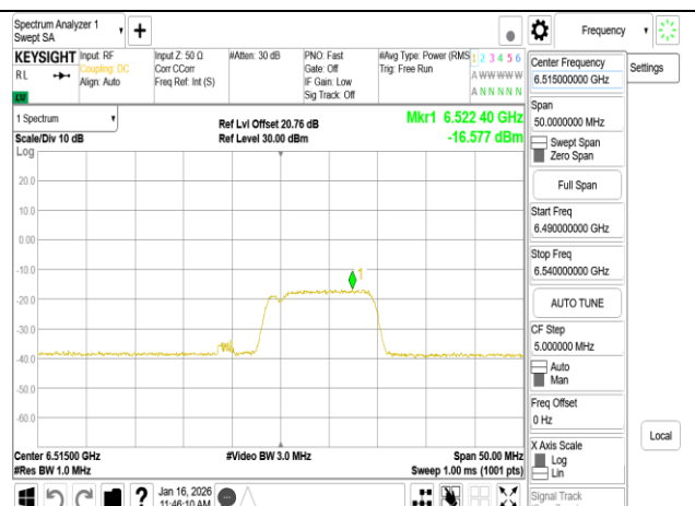
802.11be 20MHz Chain0 6515MHz 106+26 MRU2
