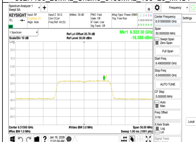
802.11be 20MHz Chain0 6515MHz RU242
