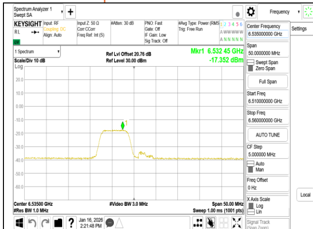
802.11be 20MHz Chain0 6535MHz 52+26 MRU1
