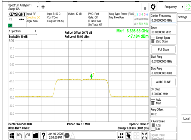
802.11be 20MHz Chain0 6695MHz RU242
