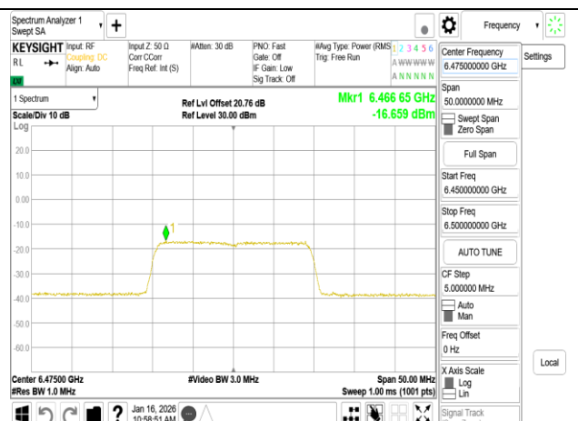
802.11be 20MHz Chain0 6475MHz RU242
