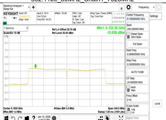
802.11be 160MHz Chain0 6185MHz
