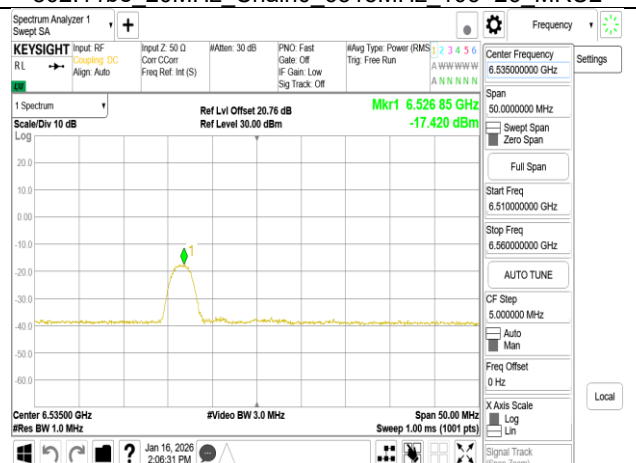
802.11be 20MHz Chain0 6535MHz RU26_0
