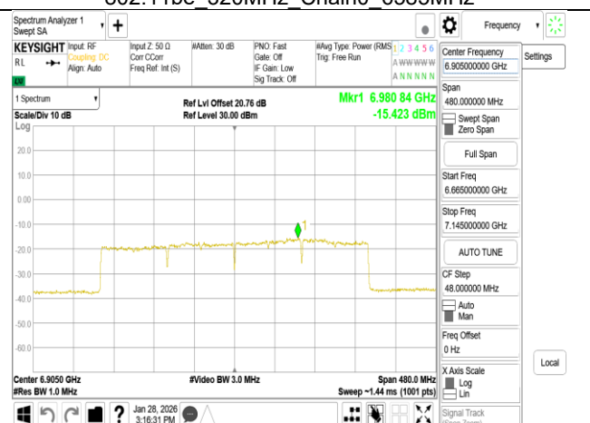
802.11be_320MHz_Chain0_6905MHz
