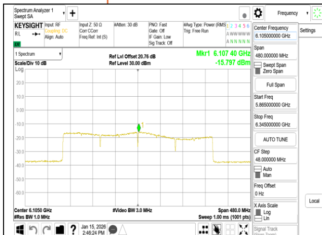
802.11be_320MHz_Chain0_6105MHz
