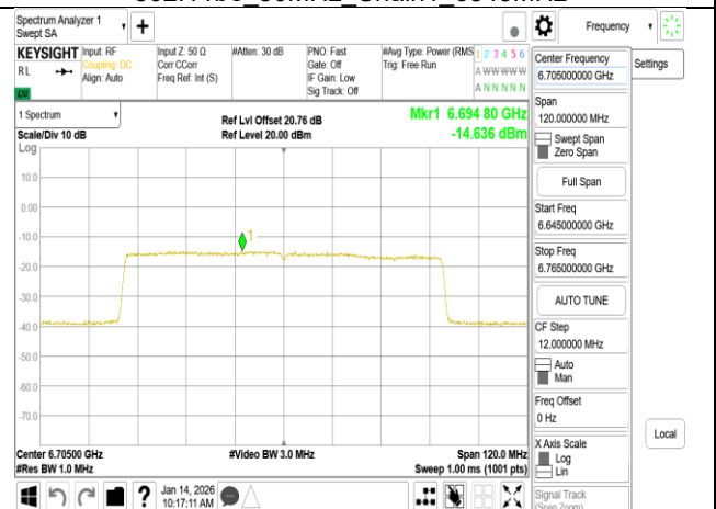
802.11be 80MHz Chain1 6705MHz
