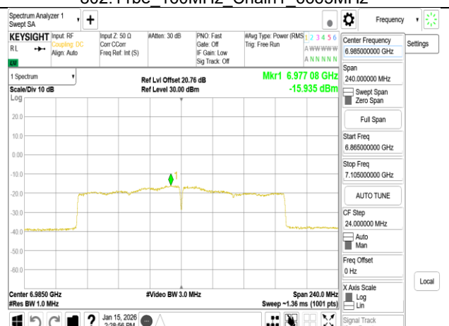
802.11be 160MHz Chain1_6985MHz
