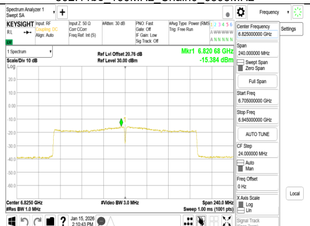
802.11be_160MHz_Chain0_6825MHz
