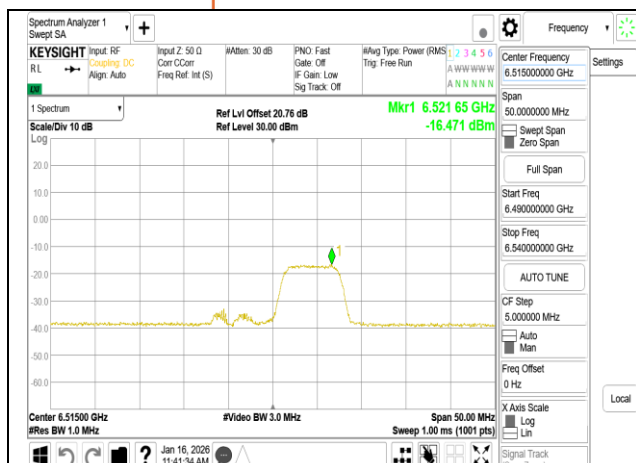
802.11be 20MHz Chain0 6515MHz 52+26 MRU3
