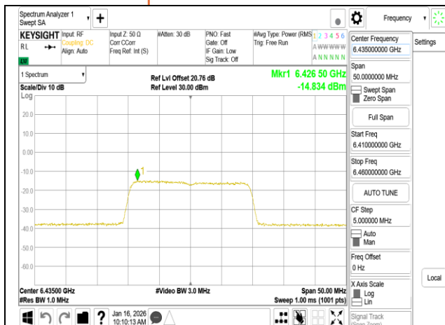
802.11be 20MHz Chain1 6435MHz RU242
