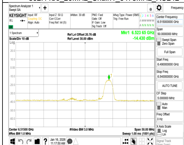
802.11be_20MHz_Chain1_6515MHz_RU26_8
