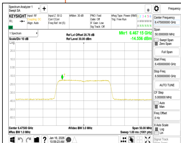
802.11be_20MHz_Chain1_6475MHz_RU242
