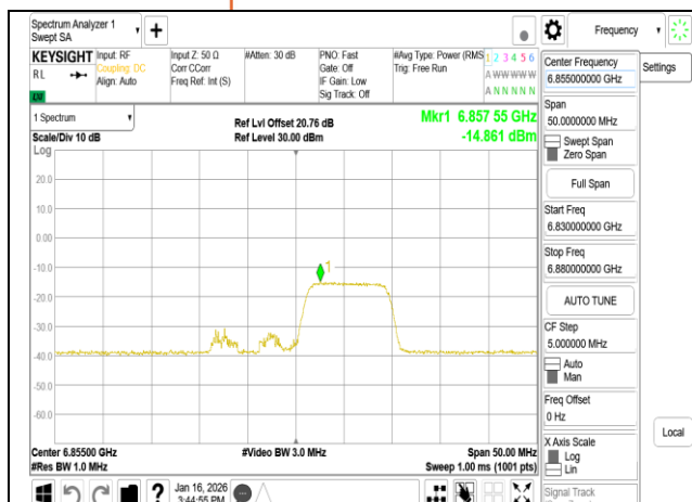
802.11be 20MHz Chain0 6855MHz RU106 54
