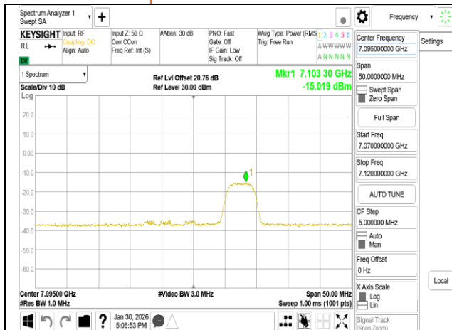
802.11be 20MHz Chain1 7095MHz RU52_40
