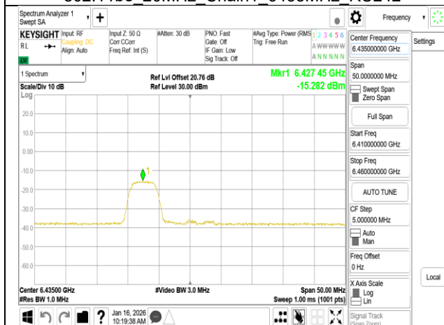
802.11be 20MHz Chain1 6435MHz RU52_37
