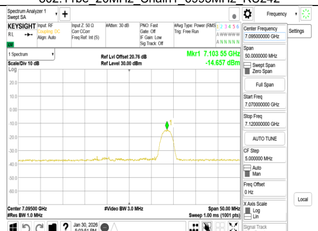
802.11be 20MHz Chain1 7095MHz RU26_8
