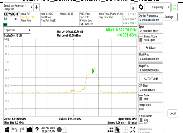
802.11be_20MHz_Chain1_6515MHz_RU52_40
