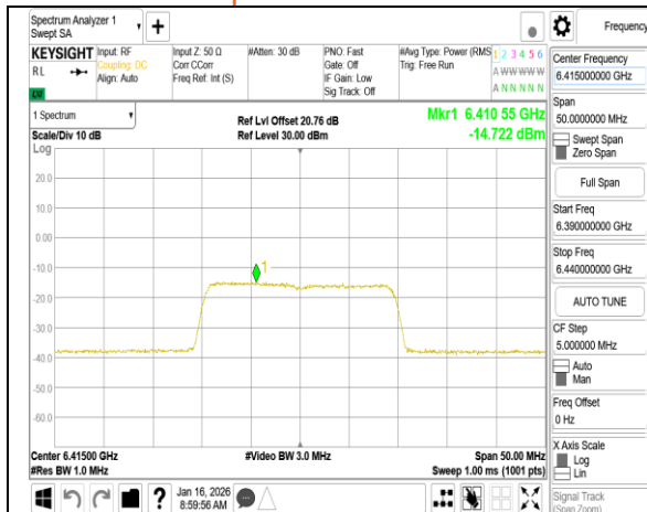
802.11be 20MHz Chain1 6415MHz RU242
