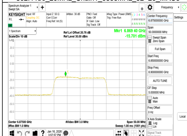
802.11be 20MHz Chain1 6875MHz RU242
