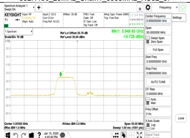
802.11be 20MHz Chain1 5955MHz 52+26 MRU1
