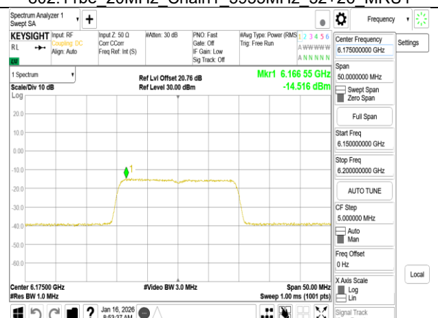
802.11be 20MHz Chain1 6175MHz RU242
