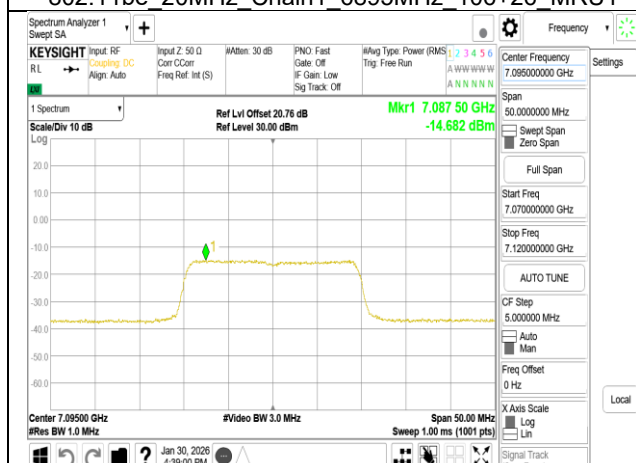
802.11be 20MHz Chain1 7095MHz RU242
