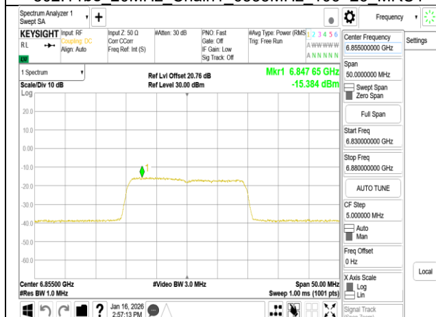
802.11be 20MHz Chain1 6855MHz RU242
