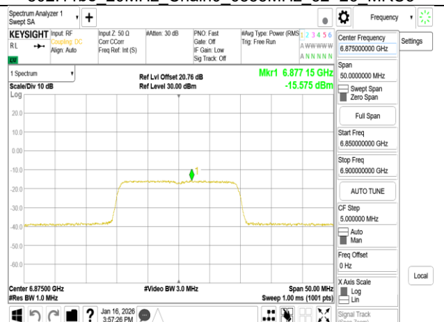
802.11be 20MHz Chain0 6875MHz RU242
