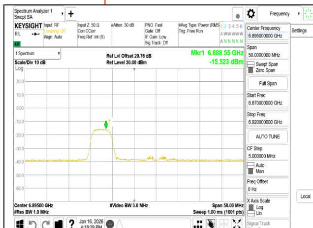
802.11be 20MHz Chain0 6895MHz RU52_37
