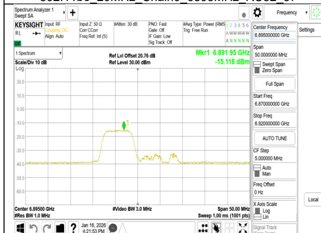
802.11be 20MHz Chain0 6895MHz 52+26 MRU1
