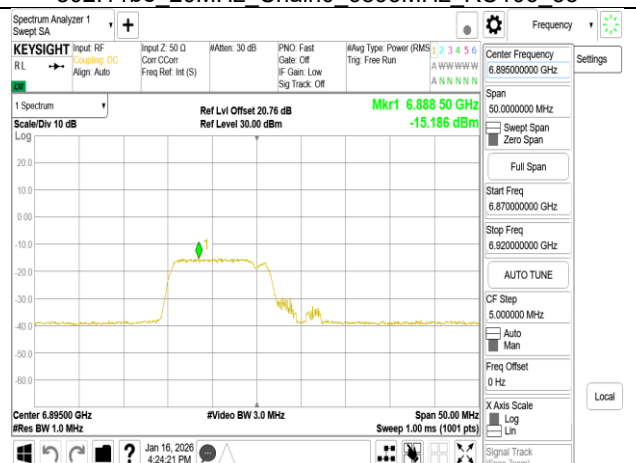
802.11be 20MHz Chain0 6895MHz 106+26 MRU1
