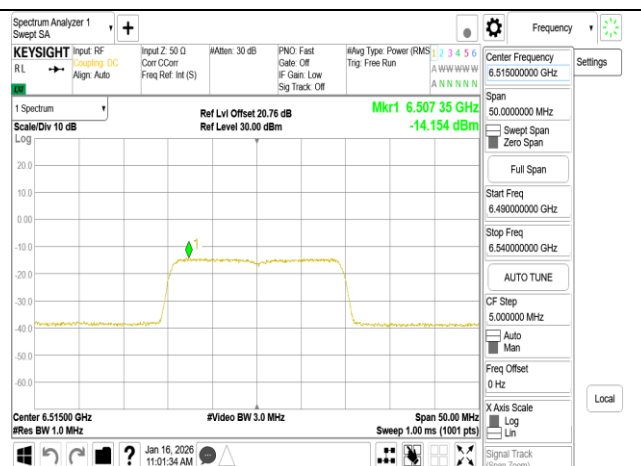
802.11be_20MHz_Chain1_6515MHz_RU242
