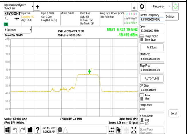
802.11be 20MHz Chain1 6415MHz RU106_54
