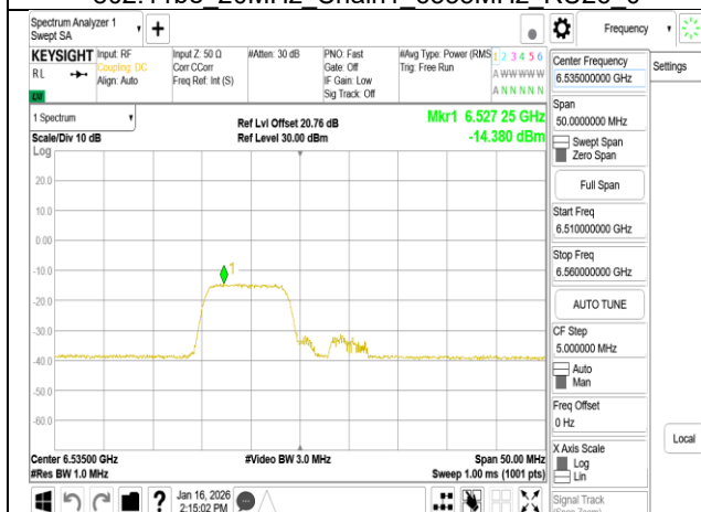
802.11be 20MHz Chain1 6535MHz RU106 53
