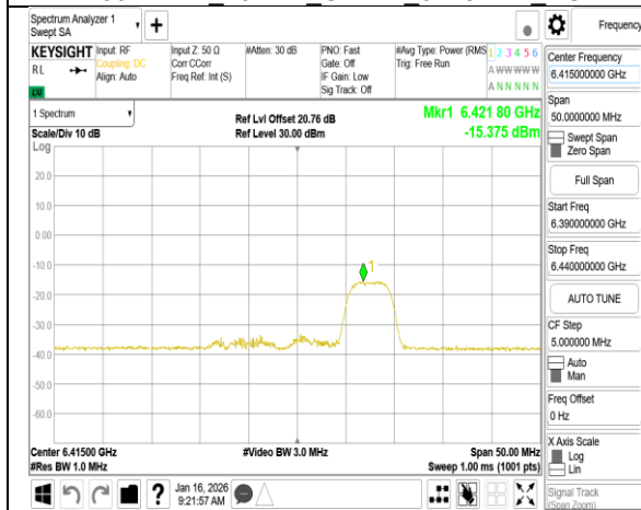
802.11be 20MHz Chain1 6415MHz RU52_40
