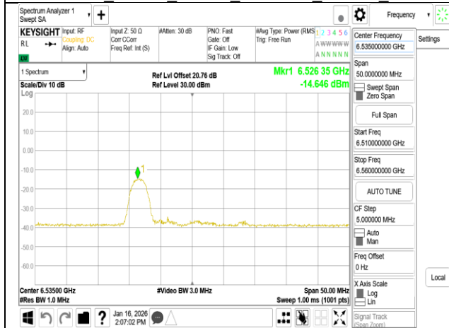
802.11be 20MHz Chain1 6535MHz RU26 0
