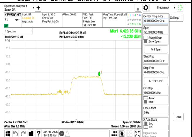
802.11be 20MHz Chain1 6415MHz 106+26_MRU2
