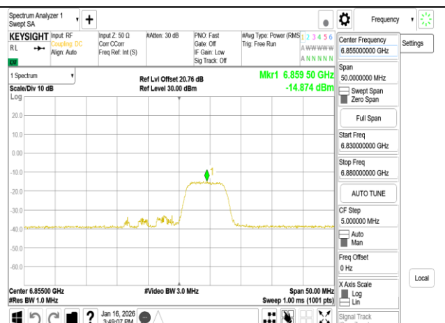
802.11be 20MHz Chain0 6855MHz 52+26 MRU3
