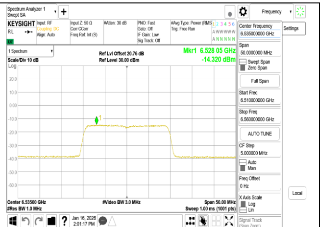
802.11be 20MHz Chain1 6535MHz RU242
