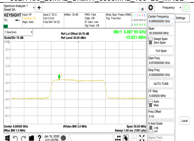
802.11be 20MHz Chain1 6895MHz RU242
