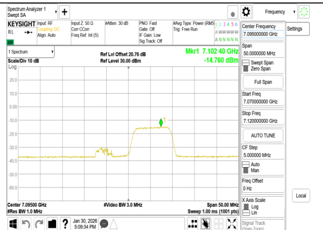
802.11be 20MHz Chain1 7095MHz RU106_54
