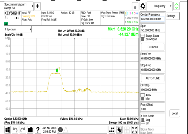
802.11be 20MHz Chain1 6535MHz RU52 37
