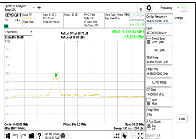
802.11be 20MHz Chain1 6435MHz RU26_0
