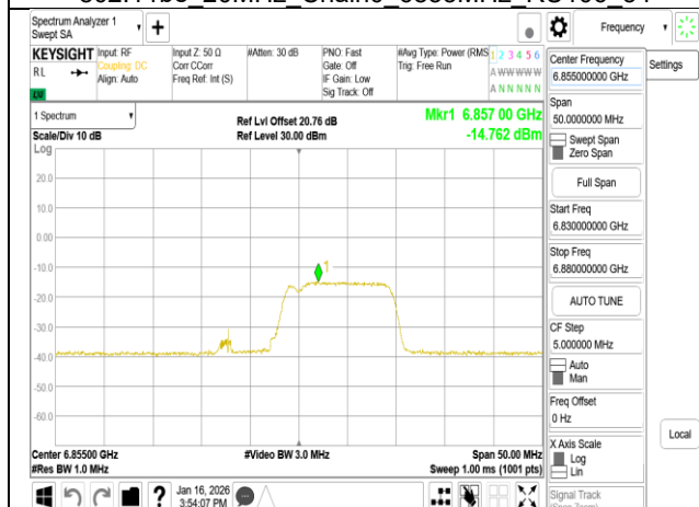
802.11be 20MHz Chain0 6855MHz 106+26 MRU2
