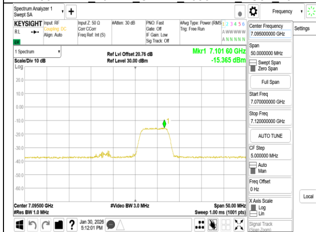
802.11be 20MHz Chain1 7095MHz 52+26_MRUI3
