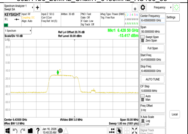
802.11be 20MHz Chain1 6435MHz 106+26_MRU1
