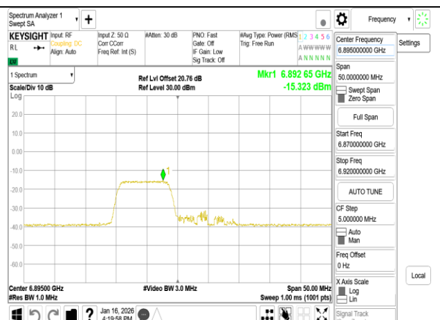
802.11be 20MHz Chain0 6895MHz RU106_53
