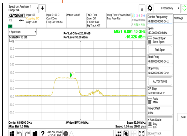
802.11be 20MHz Chain1 6895MHz RU106 53
