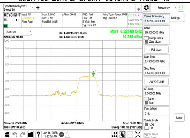
802.11be_20MHz_Chain1_6515MHz_52+26_MRU3
