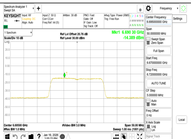
802.11be 20MHz Chain1 6695MHz RU242
