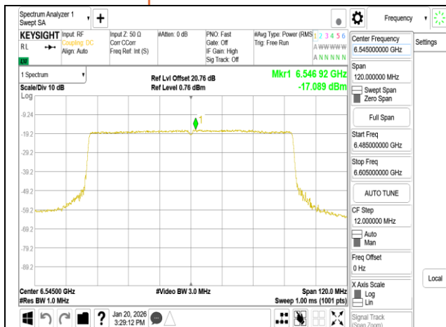
802.11be 80MHz Chain0 6545MHz RU996
