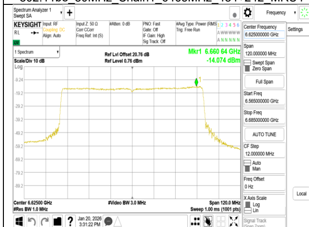
802.11be 80MHz Chain1 6625MHz RU996
