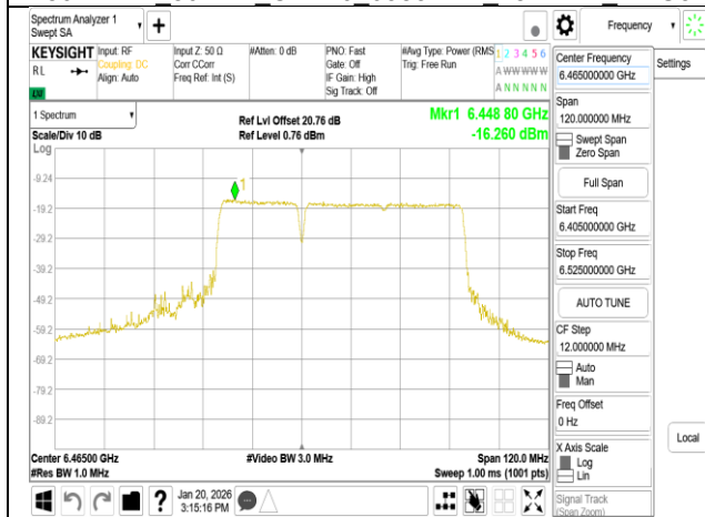
802.11be_80MHz_Chain0_6465MHz_484+242_MRU1
