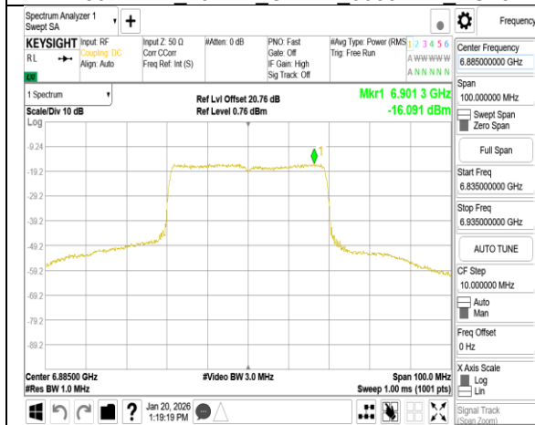
802.11be 40MHz Chain1 6885MHz RU484
