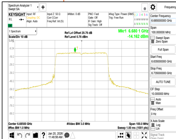
802.11be 40MHz Chain1 6685MHz RU484
