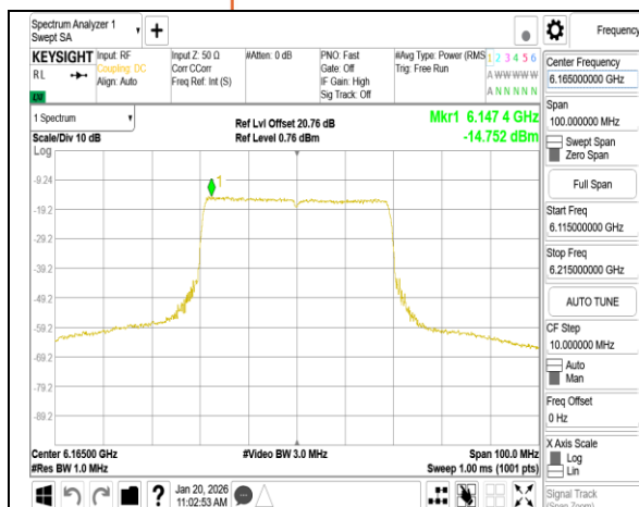
802.11be 40MHz Chain1 6165MHz RU484
