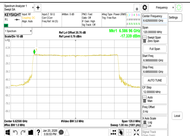
802.11be 80MHz Chain0 6625MHz RU996
