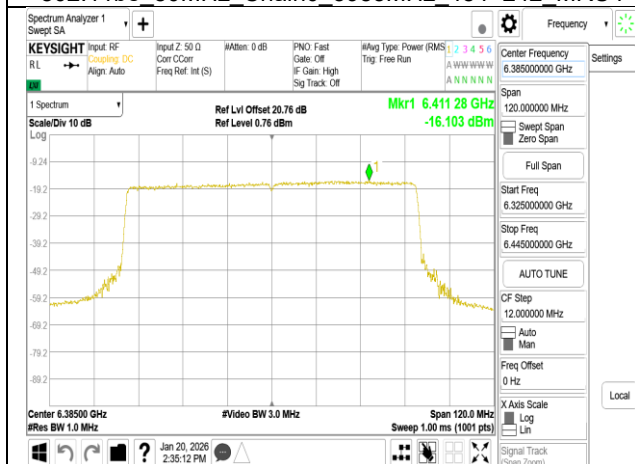
802.11be 80MHz Chain0 6385MHz RU996
