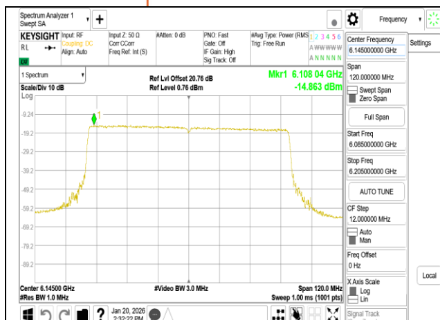
802.11be 80MHz Chain1 6145MHz RU996
