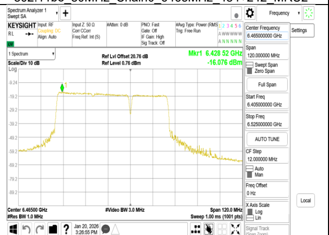
802.11be_80MHz_Chain0_6465MHz_484+242_MRU4
