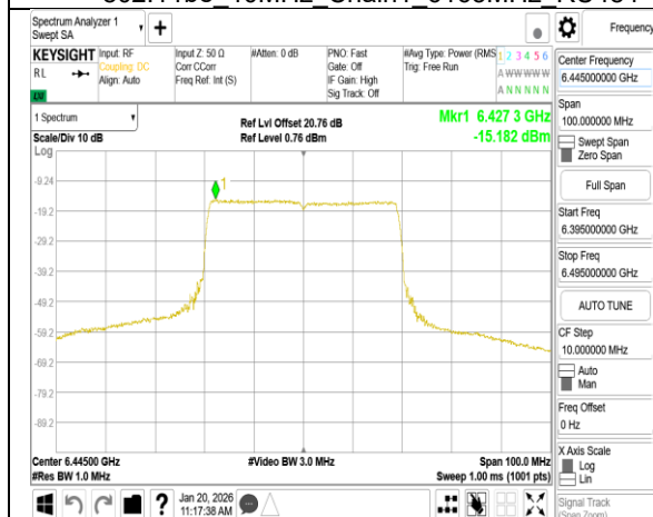
802.11be 40MHz Chain1 6445MHz RU484
