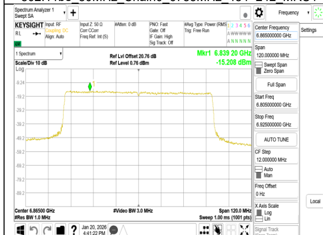
802.11be 80MHz Chain0 6865MHz RU996
