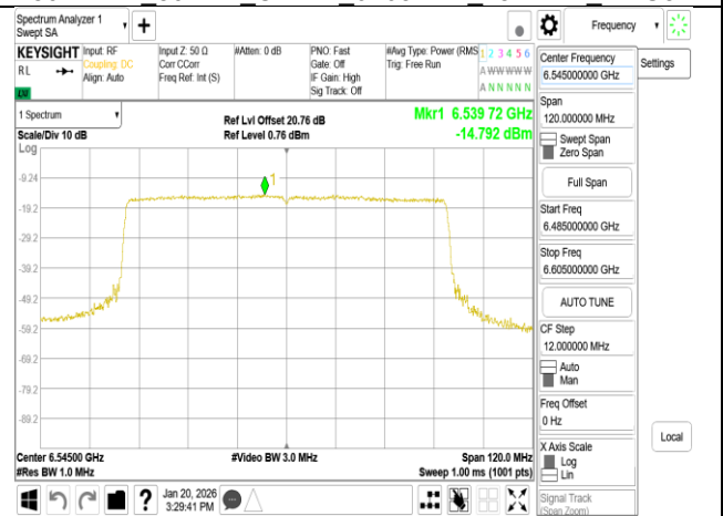
802.11be 80MHz Chain1 6545MHz RU996
