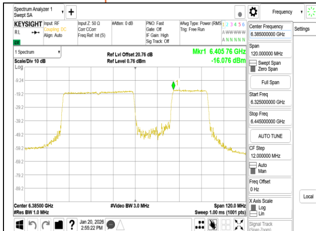
802.11be_80MHz_Chain0_6385MHz_484+242_MRU3
