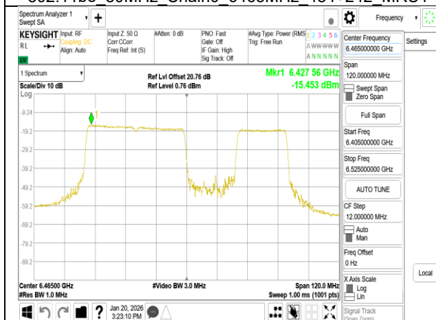
802.11be_80MHz_Chain0_6465MHz_484+242_MRU3
