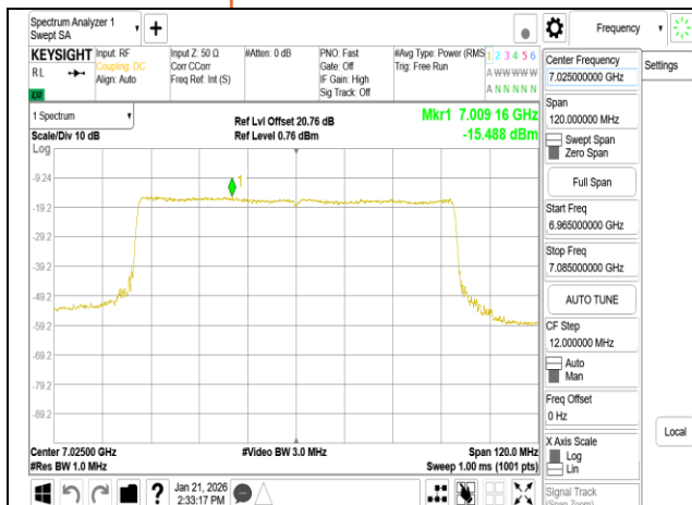
802.11be 80MHz Chain0 7025MHz RU996
