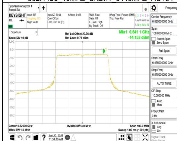
802.11be 40MHz Chain1 6525MHz RU484
