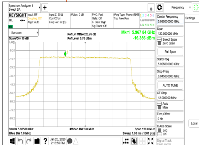
802.11be 80MHz Chain0 5985MHz RU996
