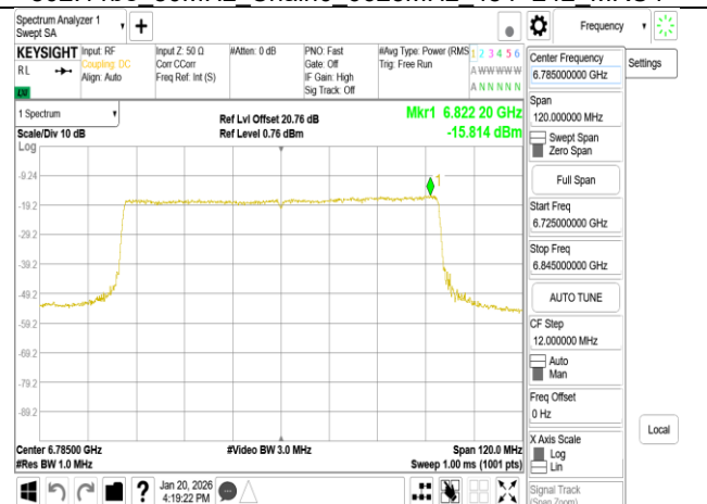
802.11be 80MHz Chain0 6785MHz RU996
