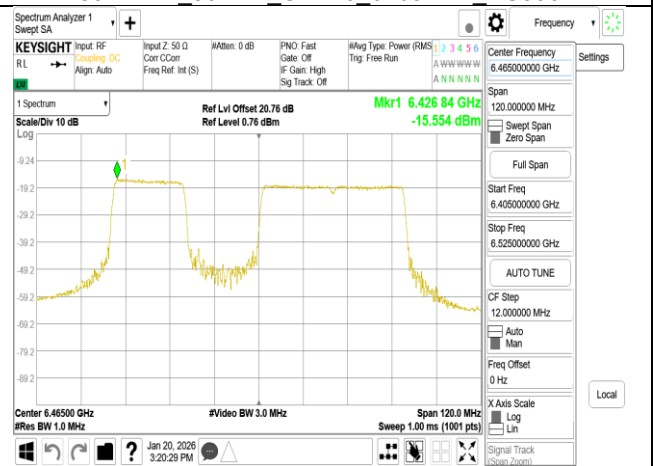
802.11be_80MHz_Chain0_6465MHz_484+242_MRU2
