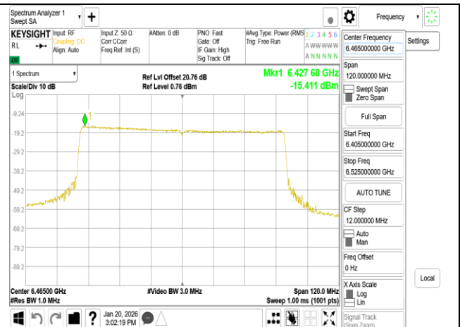
802.11be_80MHz_Chain0_6465MHz_RU996
