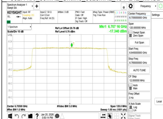
802.11be 80MHz Chain0 6705MHz RU996
