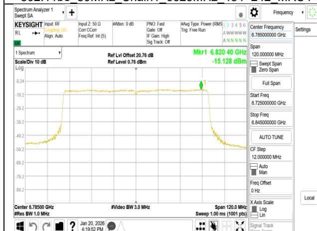
802.11be 80MHz Chain1 6785MHz RU996
