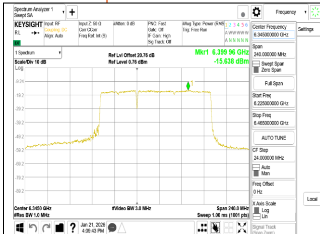
802.11be 160MHz Chain1 6345MHz 996+484 MRU1
