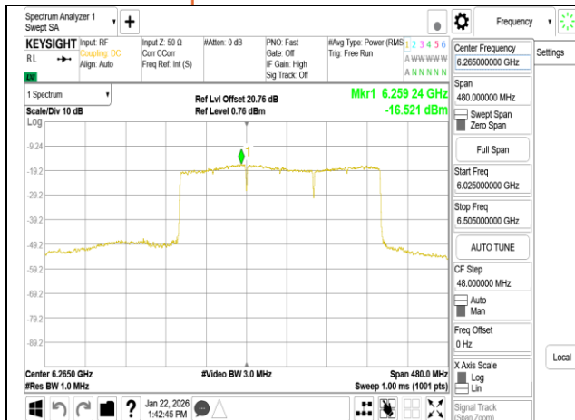
802.11be 320MHz Chain0 6265MHz 3x996 MRU1
