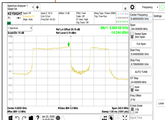
802.11be 160MHz Chain1 6665MHz 996+484 MRU3
