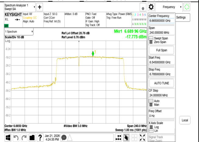
802.11be 160MHz Chain0 6665MHz 996+484 MRU1
