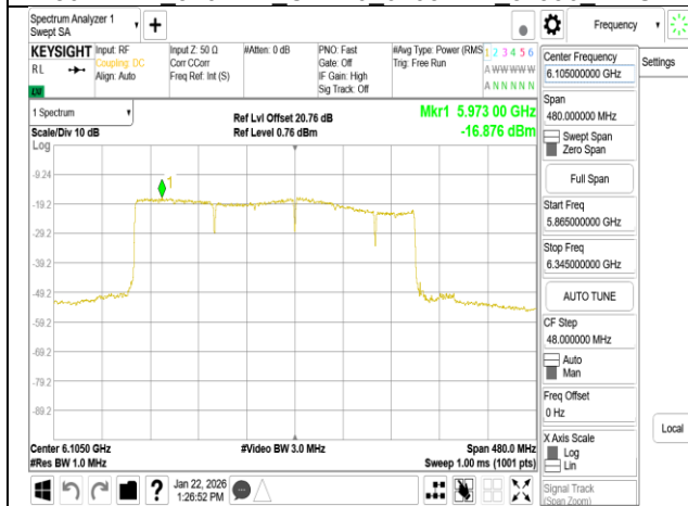
802.11be 320MHz Chain0 6105MHz 3x996+484 MRU8
