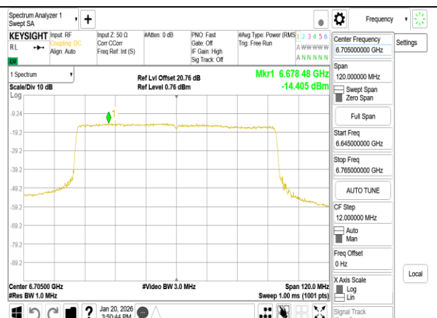
802.11be 80MHz Chain1 6705MHz RU996
