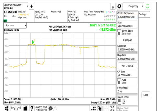
802.11be 320MHz Chain0 6105MHz 3x996+484 MRU2
