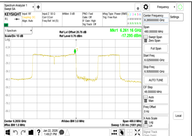
802.11be 320MHz Chain0 6265MHz 3x996 MRU3
