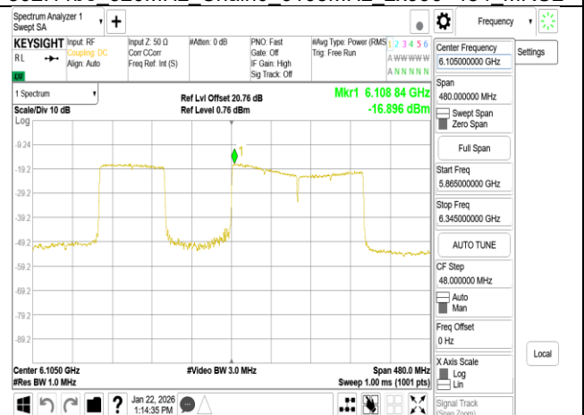
802.11be 320MHz Chain0 6105MHz 3x996 MRU2
