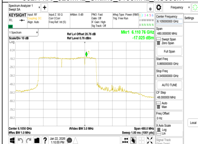
802.11be 320MHz Chain0 6105MHz 2x996+484 MRU6
