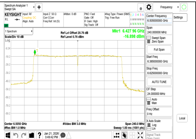
802.11be 160MHz Chain0 6505MHz RU996x2
