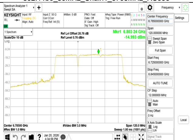
802.11be 80MHz Chain1 6785MHz 484+242 MRU1
