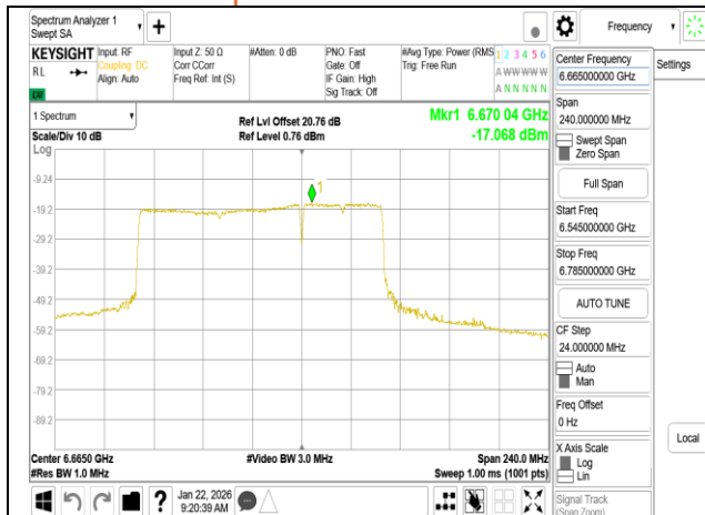
802.11be 160MHz Chain0 6665MHz 996+484 MRU4
