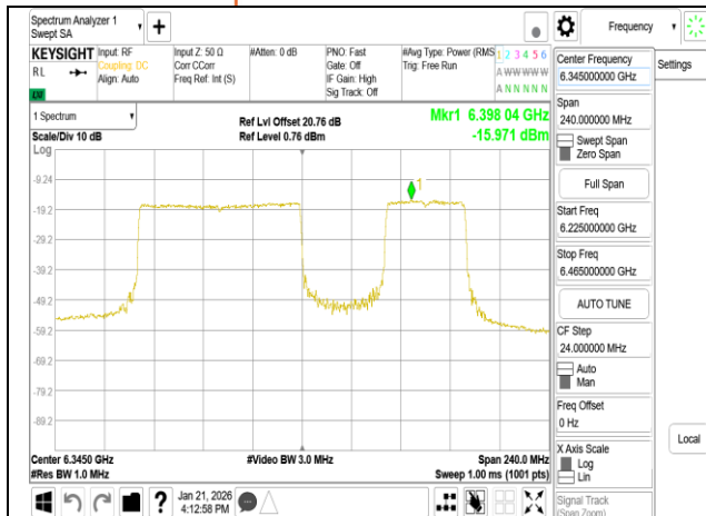
802.11be 160MHz Chain0 6345MHz 996+484 MRU3
