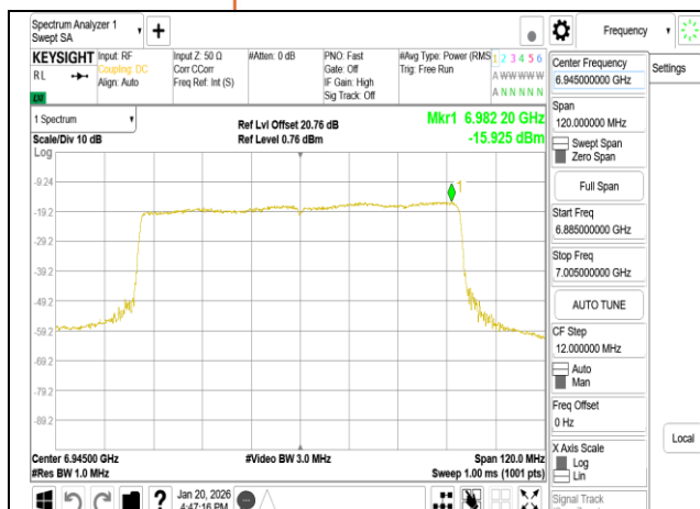
802.11be 80MHz Chain1 6945MHz RU996
