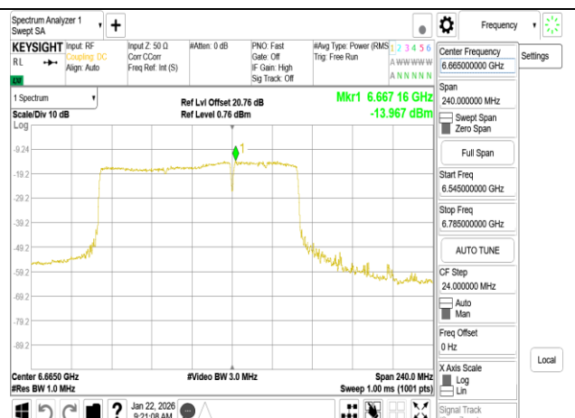
802.11be 160MHz Chain1 6665MHz 996+484 MRU4
