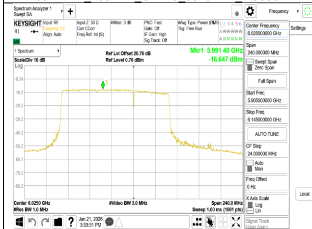
802.11be 160MHz Chain0 6025MHz 996+484 MRU4
