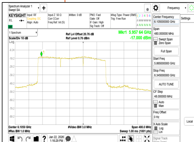
802.11be 320MHz Chain0 6105MHz 3x996 MRU4
