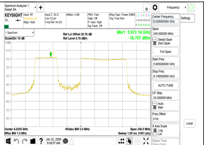
802.11be 160MHz Chain0 6025MHz 996+484 MRU2
