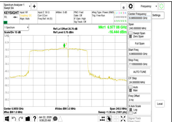
802.11be 160MHz Chain1 6985MHz 996+484 MRU4
