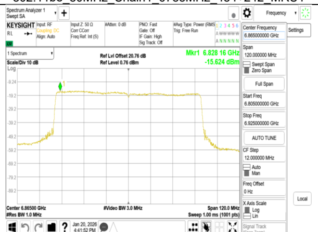
802.11be 80MHz Chain1 6865MHz RU996
