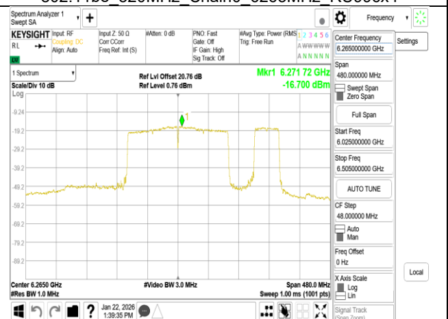
802.11be 320MHz Chain0 6265MHz 2x996+484 MRU11
