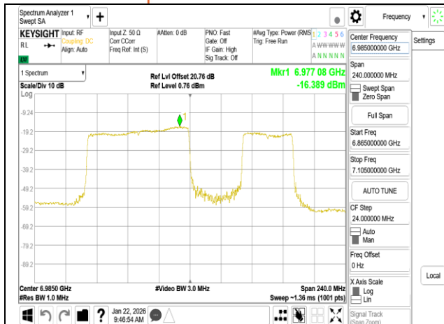
802.11be 160MHz Chain1 6985MHz 996+484 MRU3
