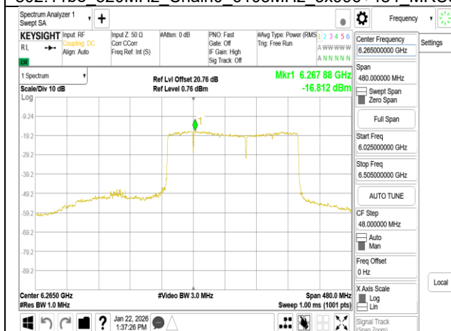
802.11be 320MHz Chain0 6265MHz 2x996+484 MRU7
