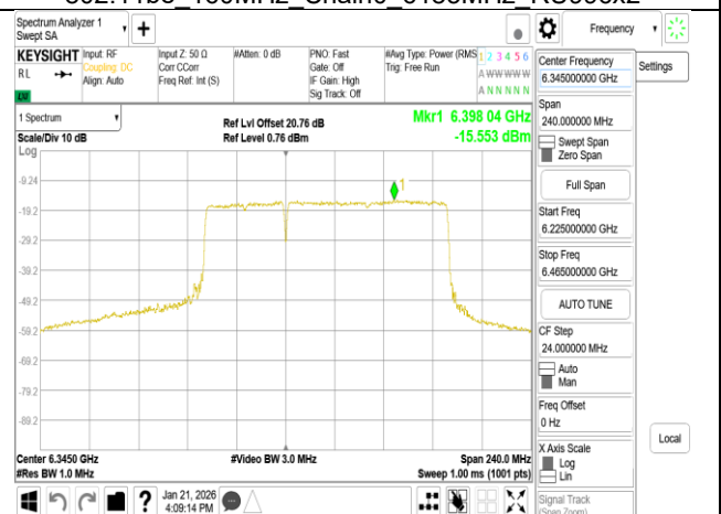
802.11be 160MHz Chain0 6345MHz 996+484 MRU1
