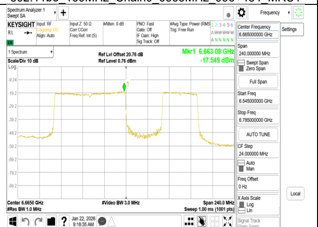
802.11be 160MHz Chain0 6665MHz 996+484 MRU3
