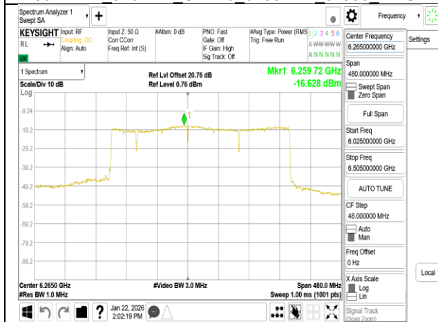
802.11be 320MHz Chain0 6265MHz 3x996+484 MRU1
