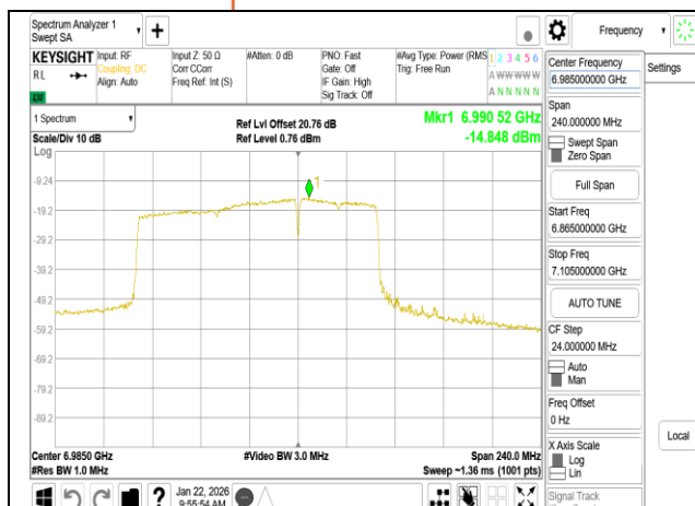
802.11be 160MHz Chain0 6985MHz 996+484 MRU4
