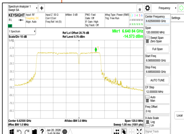
802.11be 80MHz Chain1 6625MHz 484+242 MRU4
