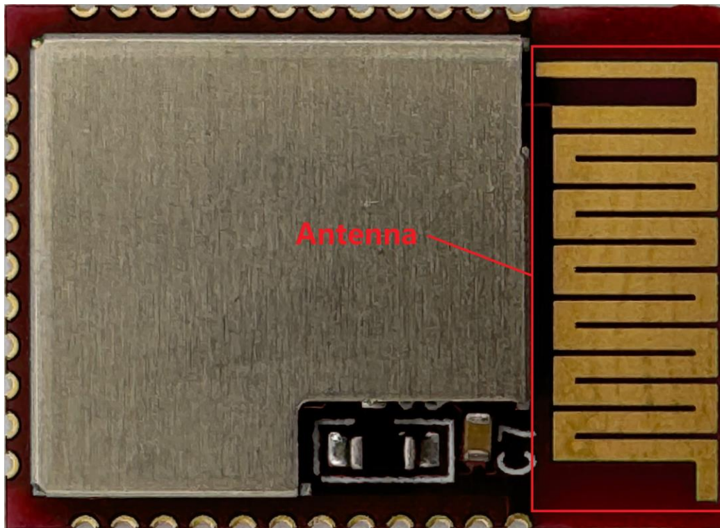
(3) EUT Photo
