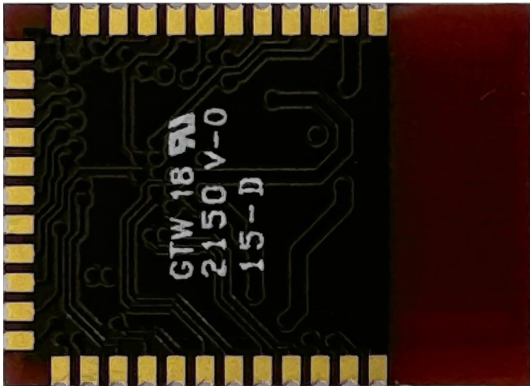
(2) EUT Photo
