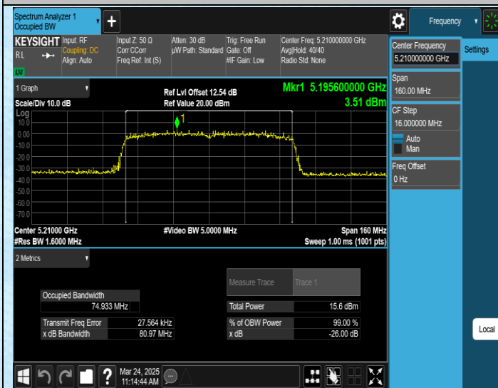
11AC80SISO-Ant1-5210
