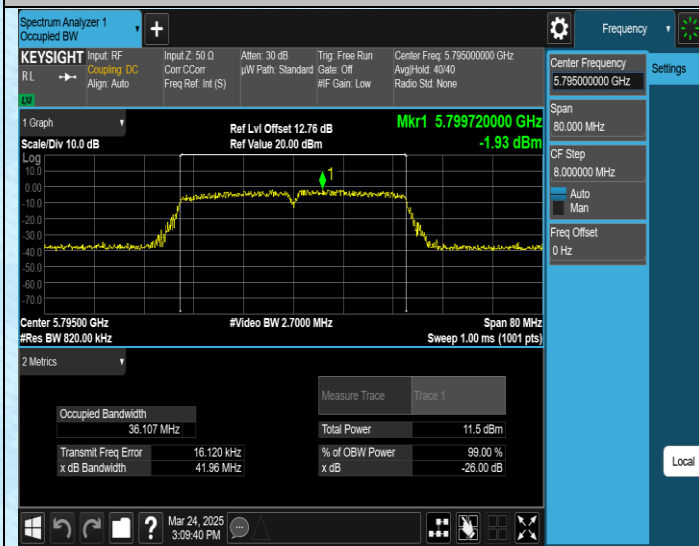
11AC40MIMO-Ant1-5795
