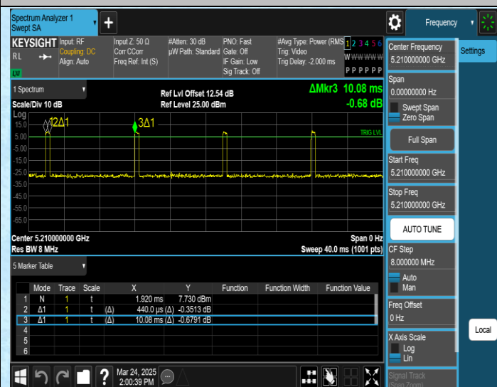
NTNV-11AC80SISO-Ant2-5210
