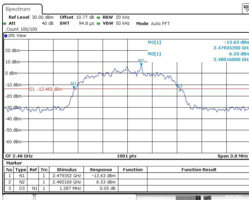
Fig. 63 20dB Bandwidth ( \pi/4 DQPSK, CH78)
