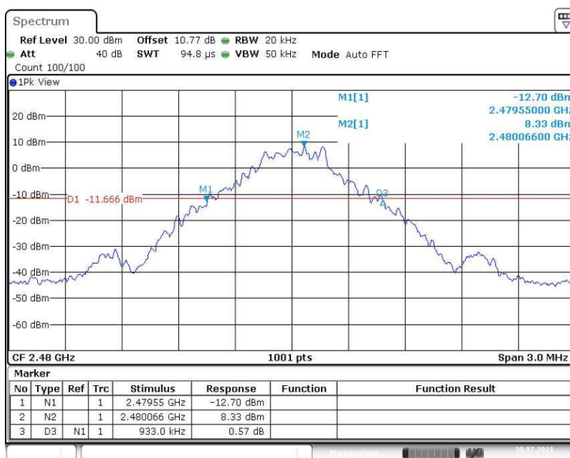
Fig. 60 20dB Bandwidth (GFSK, CH78)
