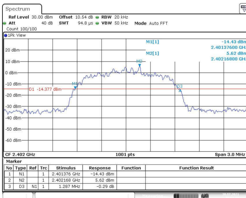
Fig. 61 20dB Bandwidth ( \pi/4 DQPSK, CH0)
