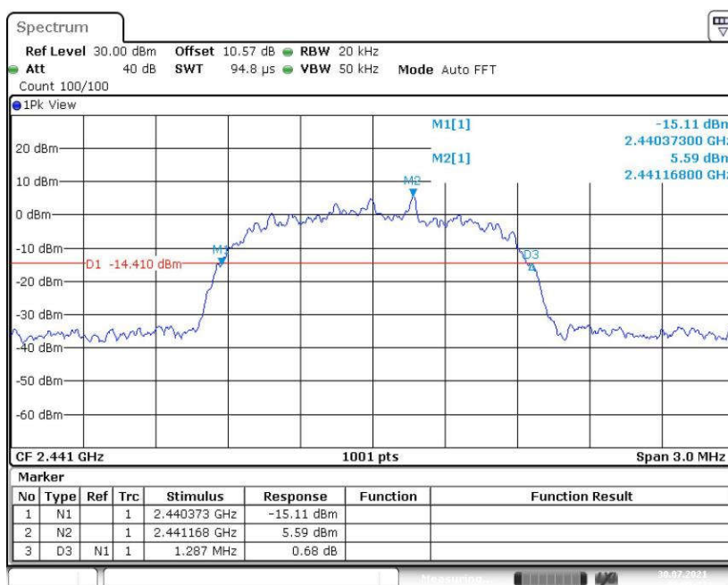
Fig. 62 20dB Bandwidth ( \pi/4 DQPSK, CH39)
