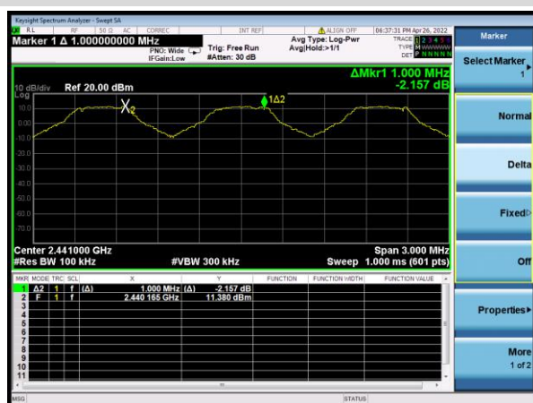
GFSK
