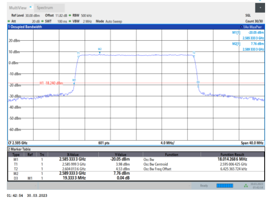
Band41-20MHz-QPSK-40640-100RB#0
