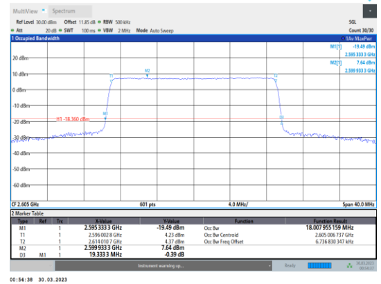
Band41-20MHz-QPSK-40740-100RB#0
