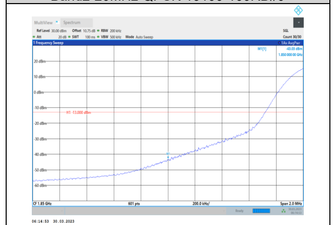
Band2-20MHz-16QAM-18700-1RB#0
