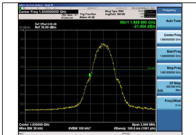
GSM1900-512-0
