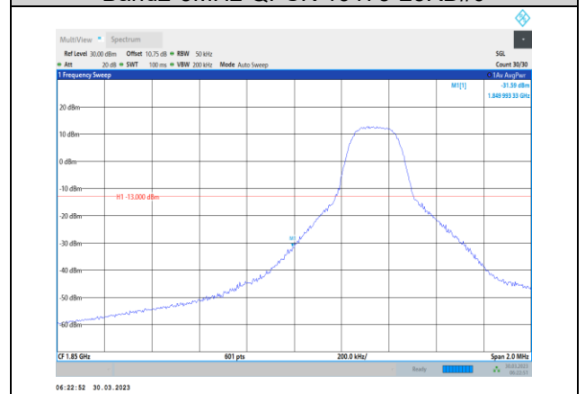
Band2-5MHz-16QAM-18625-1RB#0
