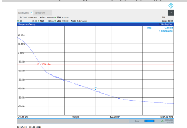
Band2-20MHz-QPSK-19100-1RB#99
