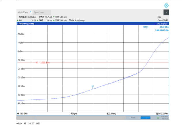
Band2-20MHz-QPSK-18700-1RB#0
