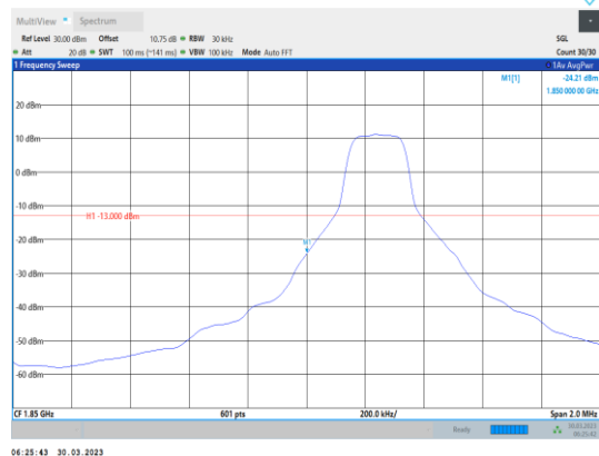
Band2-3MHz-QPSK-18615-1RB#0
