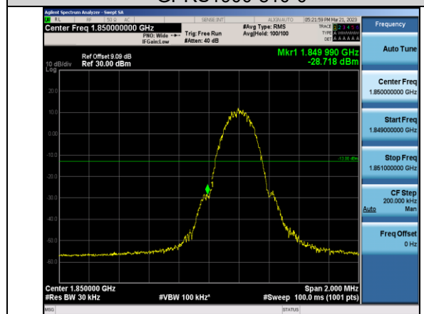
EGPRS1900-512-2
