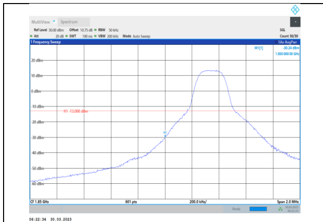
Band2-5MHz-QPSK-18625-1RB#0
