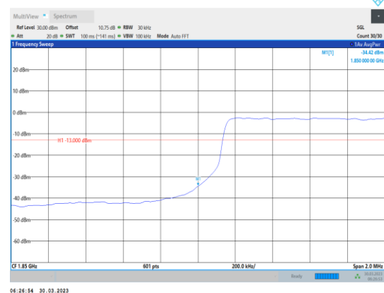
Band2-3MHz-16QAM-18615-15RB#0
