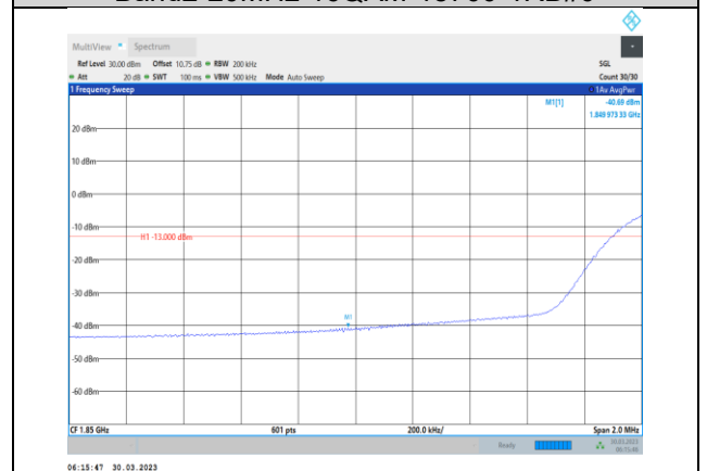
Band2-20MHz-16QAM-18700-100RB#0
