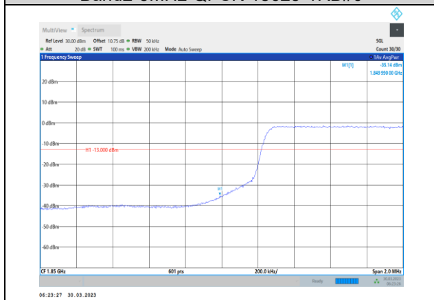
Band2-5MHz-QPSK-18625-25RB#0
