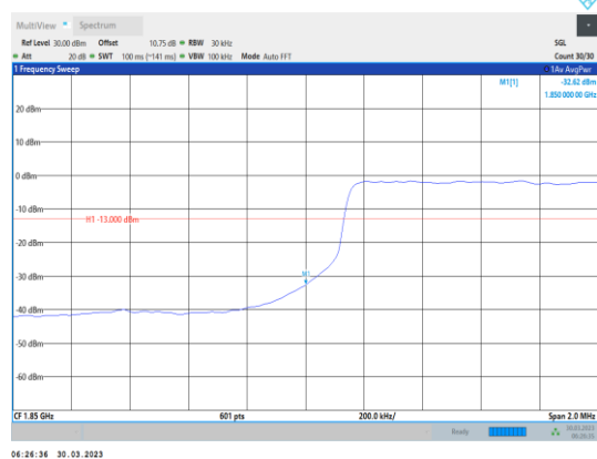
Band2-3MHz-QPSK-18615-15RB#0
