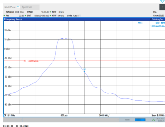
Band2-3MHz-QPSK-19185-1RB#14
