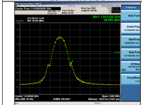
EGPRS1900-810-2
