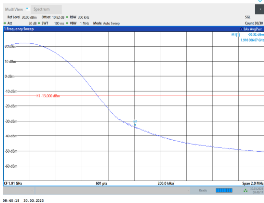
Band2-15MHz-16QAM-19125-1RB#74
