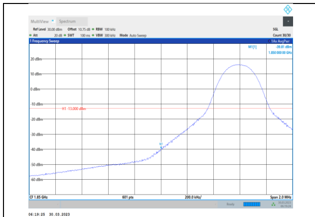
Band2-10MHz-QPSK-18650-1RB#0
