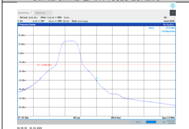
Band2-5MHz-QPSK-19175-1RB#24
