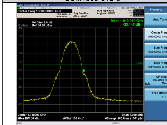
GSM1900-810-0
