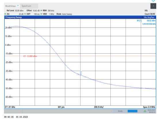
Band2-15MHz-64QAM-19125-1RB#74
