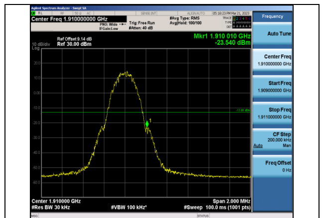
GPRS1900-810-0
