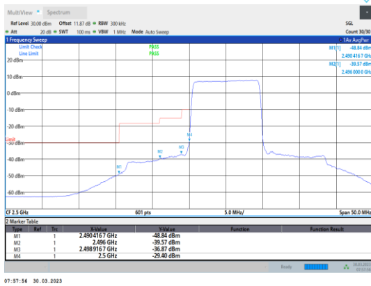
Band7-10MHz-QPSK-20800-50RB#0
