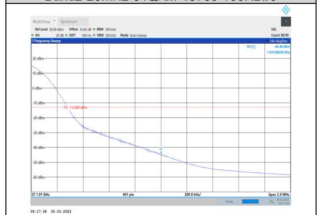
Band2-20MHz-64QAM-18700-1RB#99
