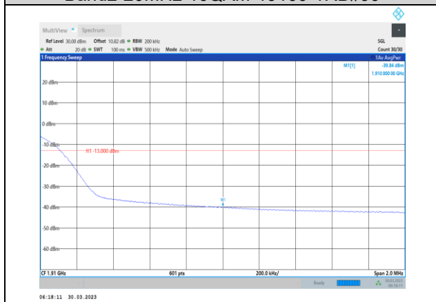
Band2-20MHz-16QAM-19100-100RB#0
