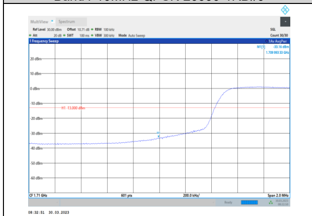
Band4-10MHz-QPSK-20000-50RB#0
