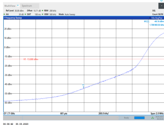
Band4-20MHz-QPSK-20050-1RB#0
