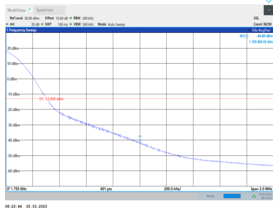
Band4-20MHz-QPSK-20300-1RB#99
