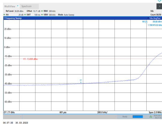
Band4-20MHz-QPSK-20050-100RB#0
