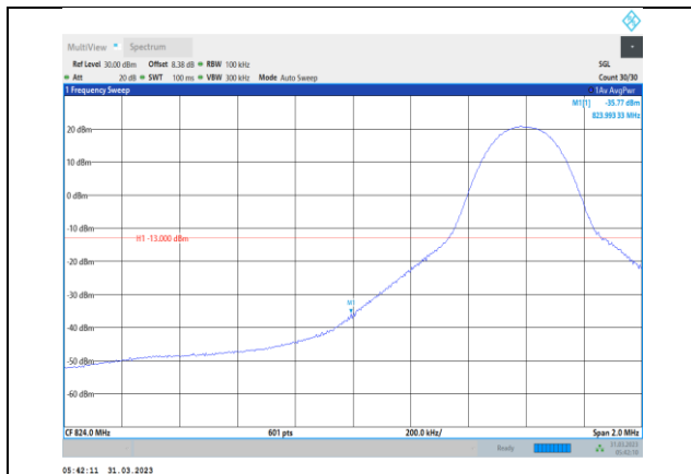
Band5-10MHz-QPSK-20450-1RB#0
