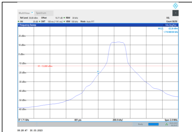
Band4-3MHz-QPSK-19965-1RB#0
