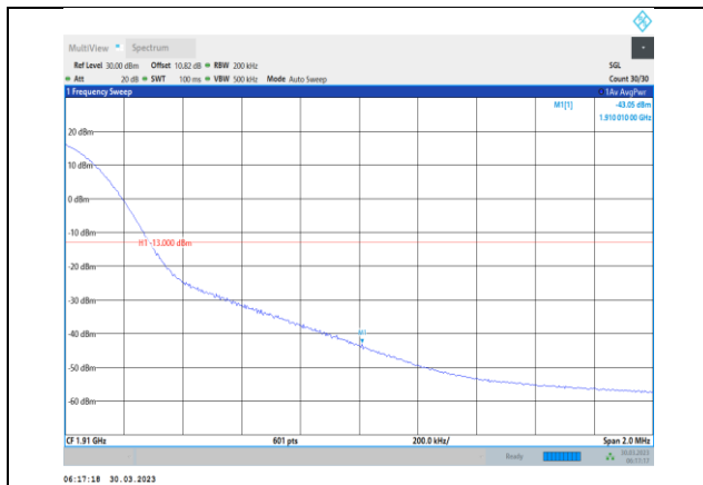
Band2-20MHz-16QAM-19100-1RB#99
