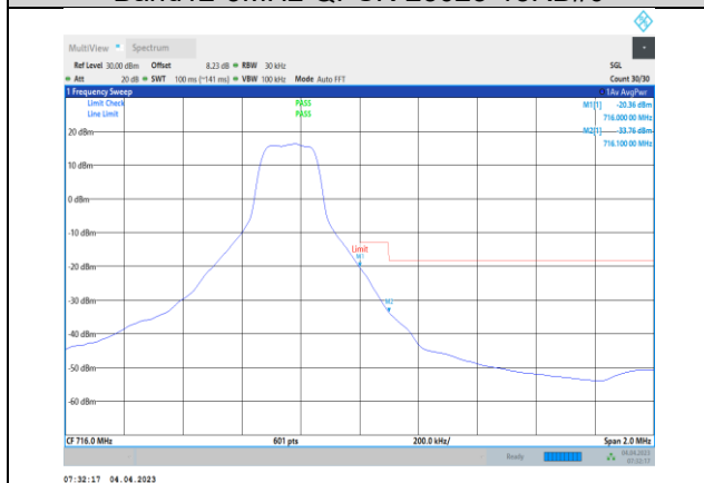
Band12-3MHz-QPSK-23165-1RB#14
