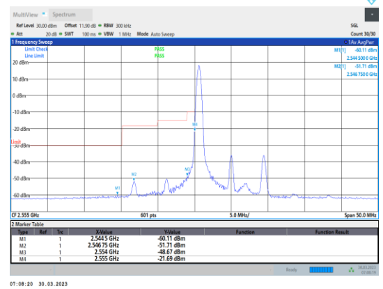
Band41-10MHz-QPSK-40290-1RB#0
