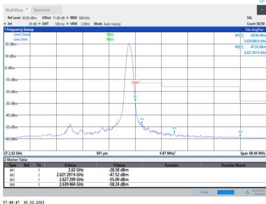
Band38-20MHz-QPSK-38150-1RB#99
