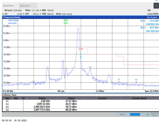
Band41-5MHz-16QAM-41565-1RB#24
