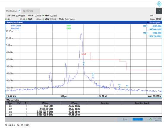
Band41-5MHz-64QAM-41565-1RB#24
