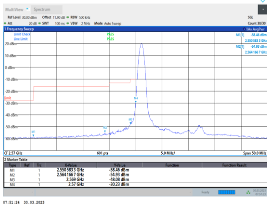
Band38-20MHz-QPSK-37850-1RB#0
