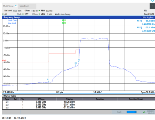
Band41-10MHz-QPSK-39700-50RB#0
