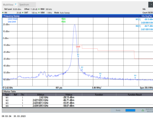
Band38-15MHz-QPSK-38175-1RB#74
