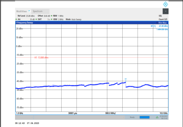
GSM850-128-1000~10000MHz
