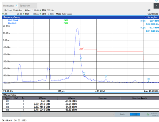
Band41-20MHz-16QAM-41490-1RB#99
