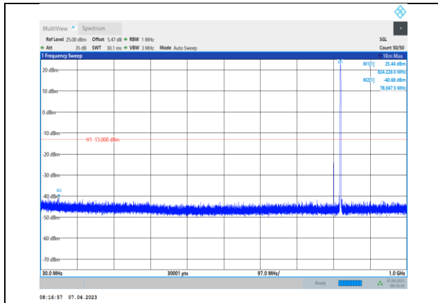
EGPRS850-128-30~1000MHz
