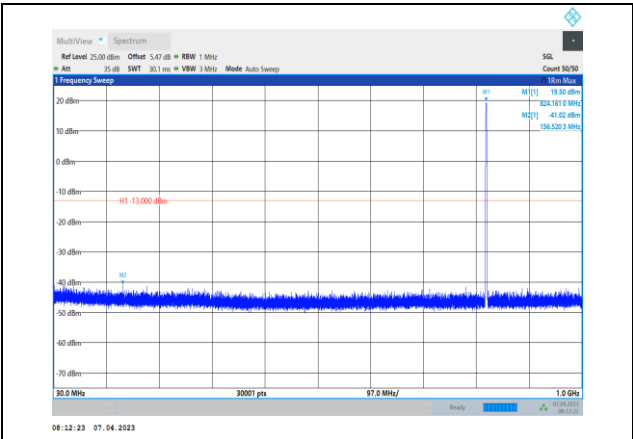
GSM850-128-30~1000MHz
