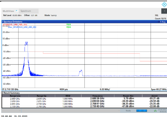
41-41-20MHz-20MHz-16QAM-16QAM-41292-41490-1RB#99-1RB#99
