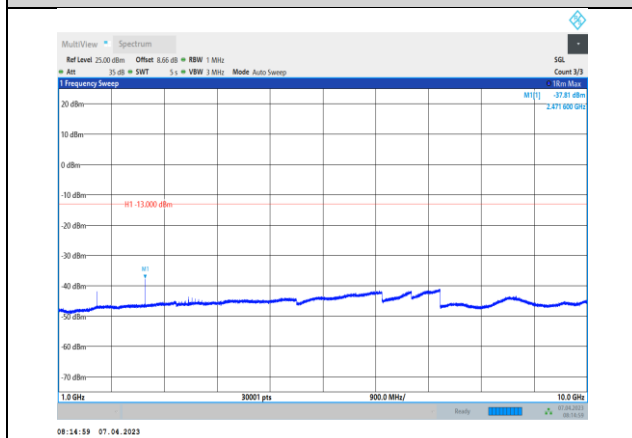
GPRS850-128-1000~10000MHz
