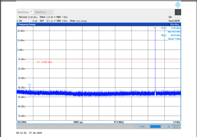
GSM850-251-30~1000MHz
