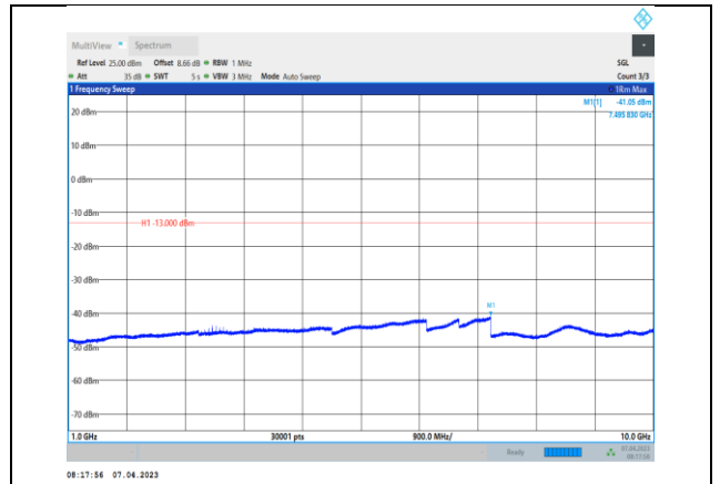
EGPRS850-190-1000~10000MHz
