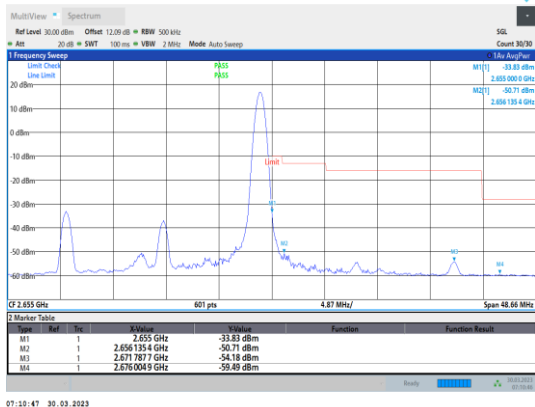
Band41-20MHz-QPSK-41140-1RB#99
