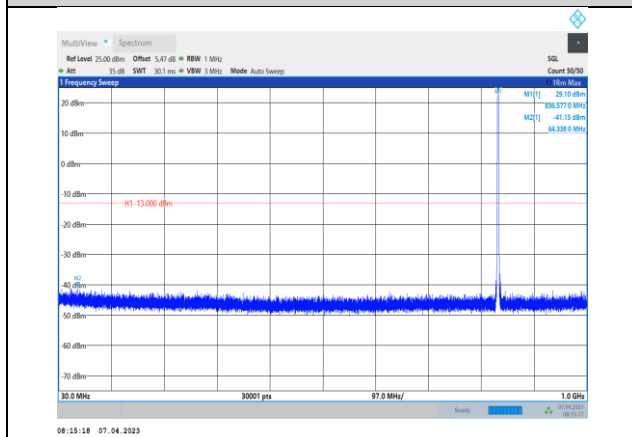
GPRS850-190-30~1000MHz
