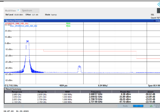
41-41-20MHz-20MHz-64QAM-64QAM-41292-41490-1RB#99-1RB#99
