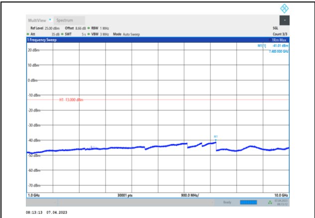
GSM850-190-1000~10000MHz
