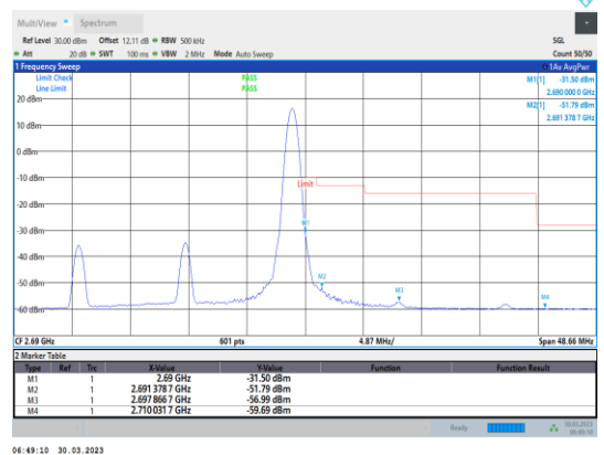
Band41-20MHz-64QAM-41490-1RB#99
