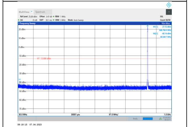
EGPRS850-251-30~1000MHz
