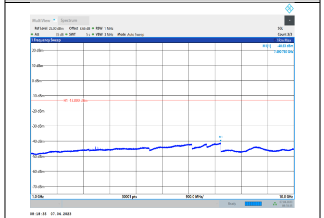
EGPRS850-251-1000~10000MHz
