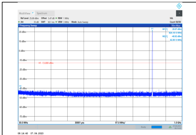
GPRS850-128-30~1000MHz
