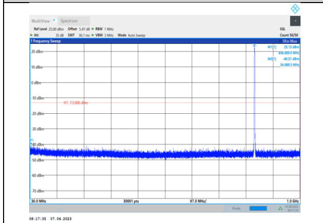
EGPRS850-190-30~1000MHz
