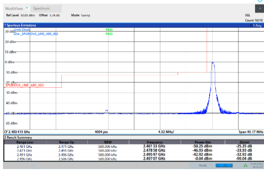
41-41-20MHz-5MHz-QPSK-QPSK-39750-39867-1RB#0-1RB#0
