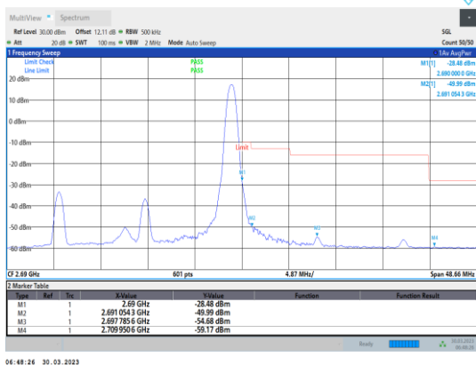
Band41-20MHz-QPSK-41490-1RB#99
