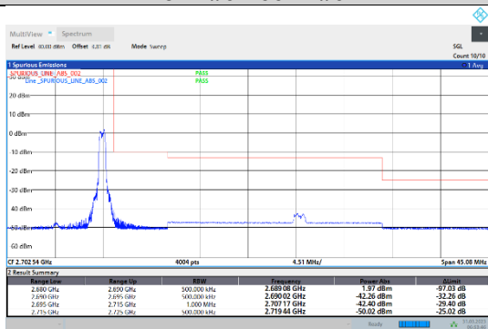
41-41-5MHz-20MHz-QPSK-QPSK-41373-41490-1RB#24-1RB#99
