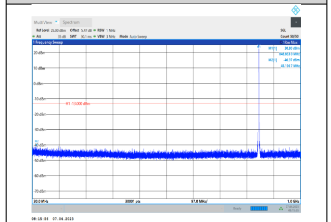
GPRS850-251-30~1000MHz
