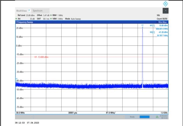
GSM850-190-30~1000MHz
