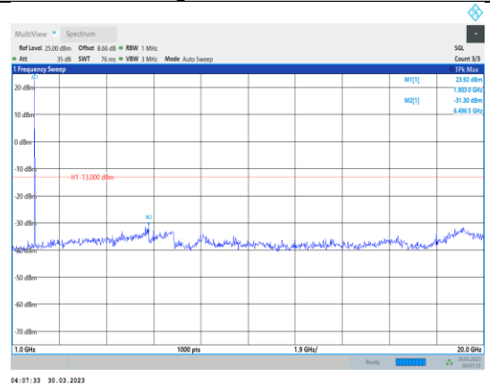
Band2-15MHz-QPSK-19125-1RB#0- Range2:1000~20000MHz
