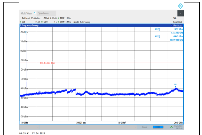
Band4-1413-1000~20000MHz
