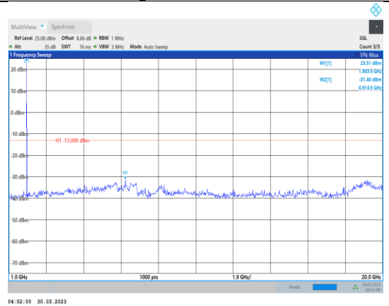
Band2-5MHz-16QAM-19175-1RB#0- Range2:1000~20000MHz
