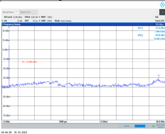
Band2-20MHz-QPSK-18700-1RB#0- Range2:1000~20000MHz
