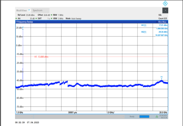
Band2-9538-1000~20000MHz
