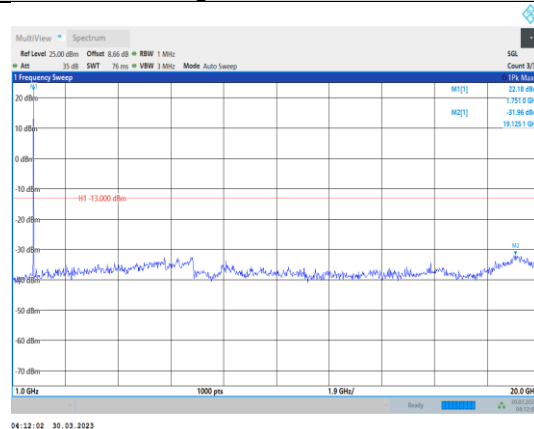
Band4-10MHz-QPSK-20350-1RB#0- Range2:1000~20000MHz
