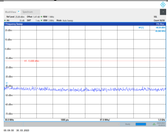
Band4-1.4MHz-QPSK-20393-1RB#0- Range1:30~1000MHz
