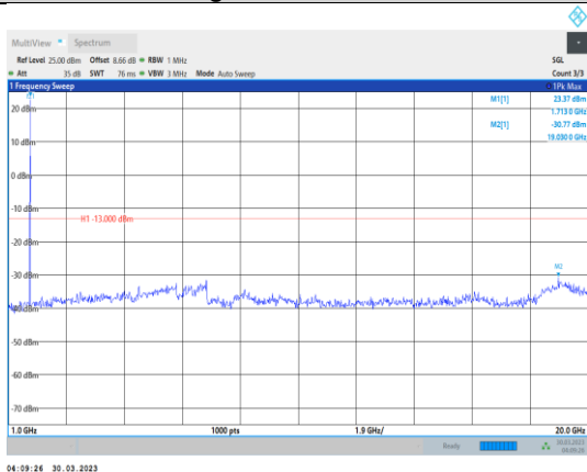
Band4-10MHz-QPSK-20000-1RB#0- Range2:1000~20000MHz
