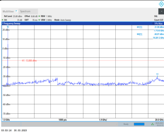
Band4-3MHz-QPSK-19965-1RB#0- Range2:1000~20000MHz
