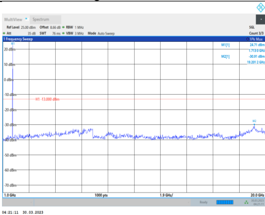
Band4-5MHz-QPSK-19975-1RB#0- Range2:1000~20000MHz
