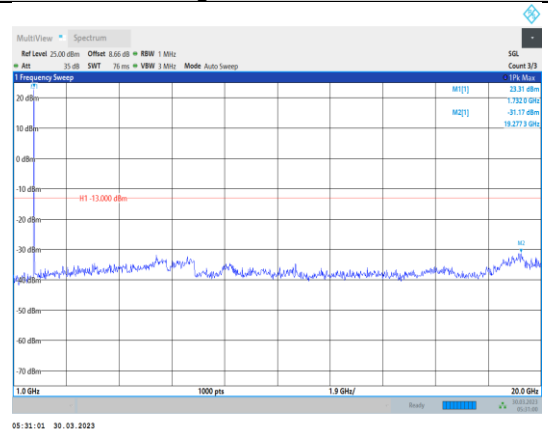
Band4-20MHz-QPSK-20300-1RB#0-Range2:1000~20000MHz
