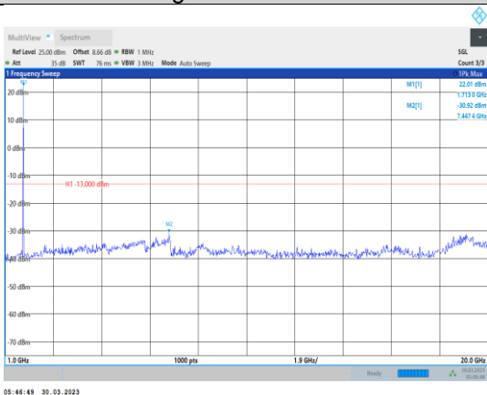
Band4-15MHz-QPSK-20025-1RB#0- Range2:1000~20000MHz
