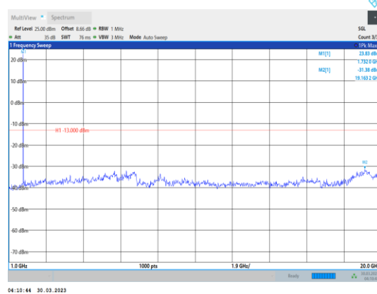
Band4-10MHz-QPSK-20175-1RB#0- Range2:1000~20000MHz
