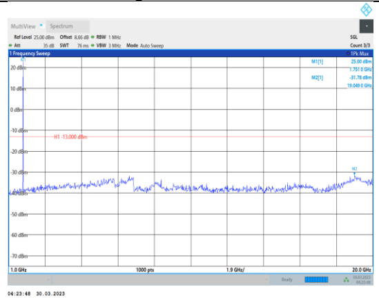
Band4-5MHz-QPSK-20375-1RB#0- Range2:1000~20000MHz
