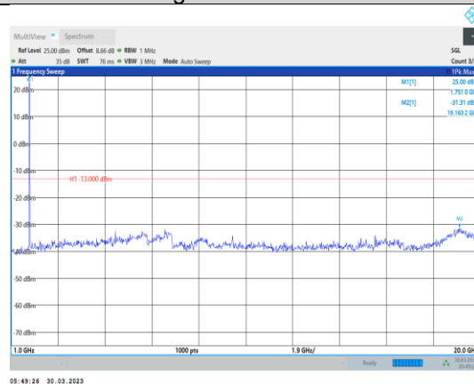
Band4-15MHz-QPSK-20325-1RB#0- Range2:1000~20000MHz
