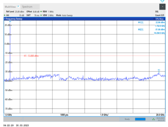
Band4-5MHz-QPSK-20175-1RB#0- Range2:1000~20000MHz
