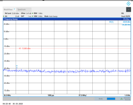
Band4-5MHz-QPSK-20375-1RB#0- Range1:30~1000MHz
