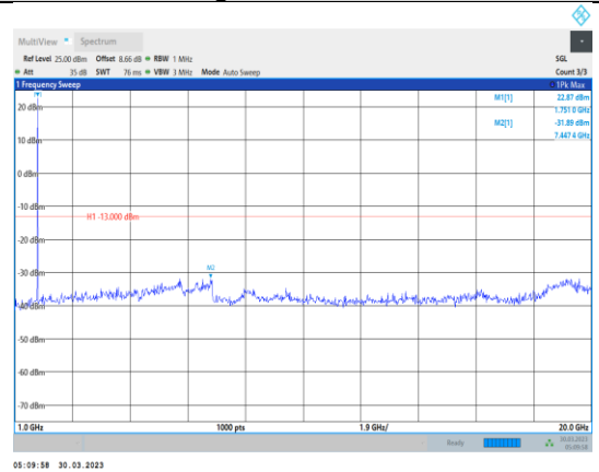
Band4-1.4MHz-QPSK-20393-1RB#0- Range2:1000~20000MHz
