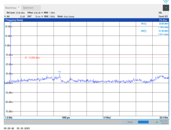
Band4-20MHz-QPSK-20175-1RB#0-Range2:1000~20000MHz
