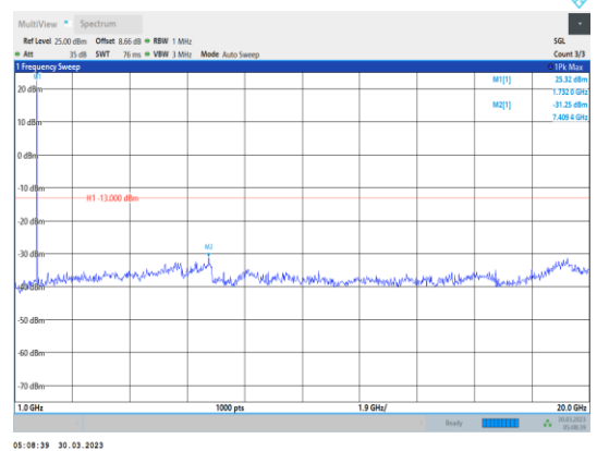
Band4-1.4MHz-QPSK-20175-1RB#0- Range2:1000~20000MHz
