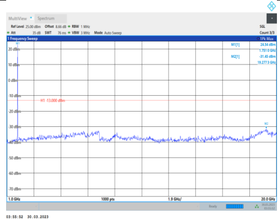
Band4-3MHz-QPSK-20385-1RB#0- Range2:1000~20000MHz
