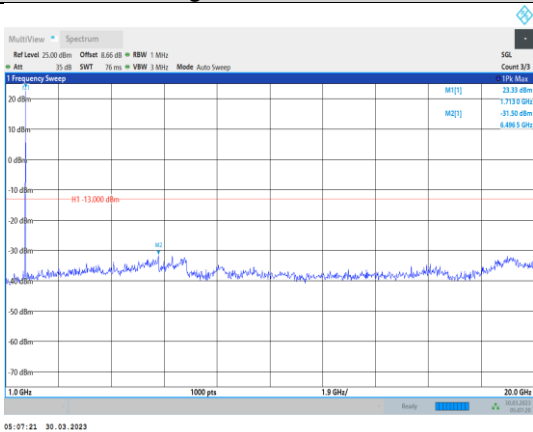
Band4-1.4MHz-QPSK-19957-1RB#0- Range2:1000~20000MHz
