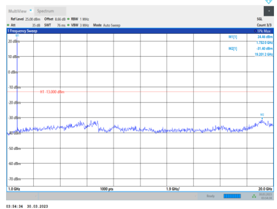
Band4-3MHz-QPSK-20175-1RB#0- Range2:1000~20000MHz
