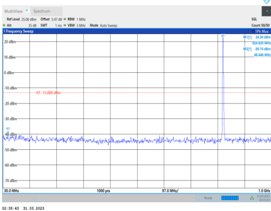
Band5-3MHz-QPSK-20415-1RB#0- Range1:30~1000MHz
