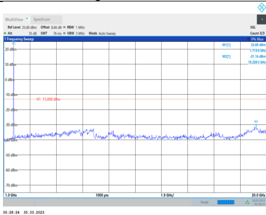
Band4-20MHz-QPSK-20050-1RB#0-Range2:1000~20000MHz
