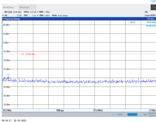
Band4-10MHz-QPSK-20000-1RB#0- Range1:30~1000MHz
