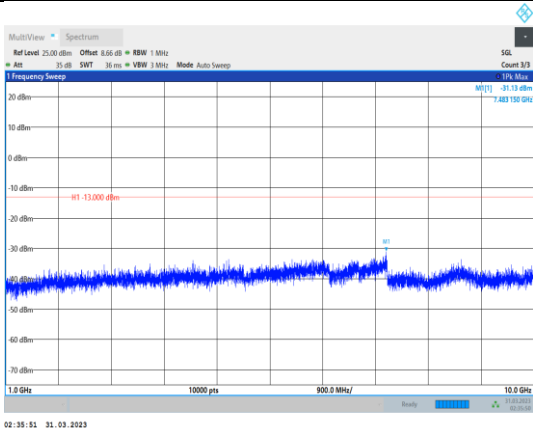
Band5-3MHz-QPSK-20415-1RB#0- Range2:1000~10000MHz
