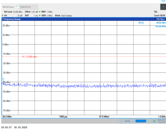
Band4-3MHz-QPSK-19965-1RB#0- Range1:30~1000MHz
