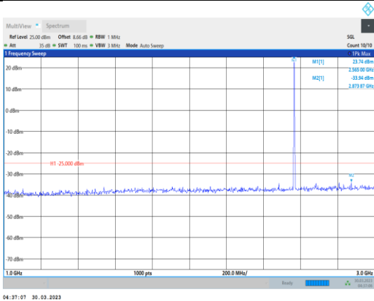
Band7-5MHz-QPSK-21425-1RB#0- Range2:1000~3000MHz
