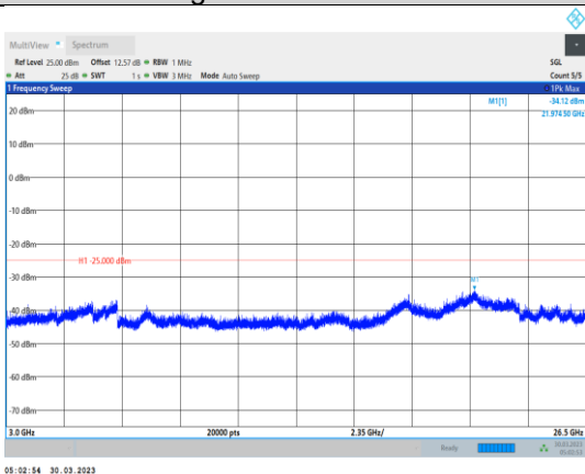
Band7-20MHz-QPSK-21100-1RB#0- Range3:3000~26500MHz
