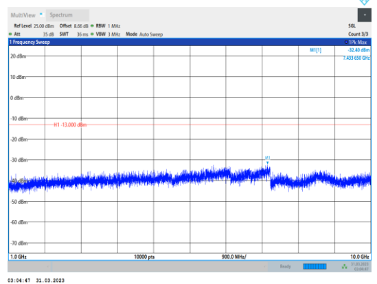
Band5-10MHz-QPSK-20525-1RB#0- Range2:1000~10000MHz
