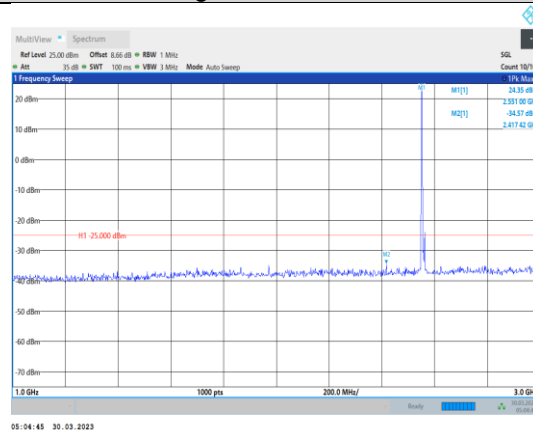
Band7-20MHz-QPSK-21350-1RB#0- Range2:1000~3000MHz
