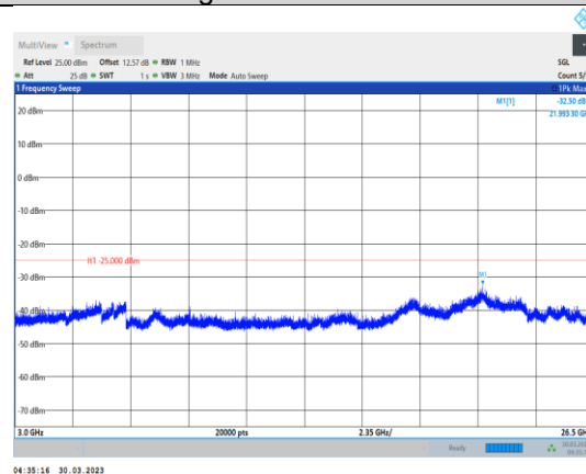
Band7-5MHz-QPSK-21100-1RB#0- Range3:3000~26500MHz
