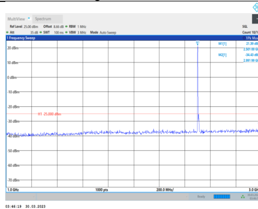
Band7-10MHz-QPSK-20800-1RB#0- Range2:1000~3000MHz
