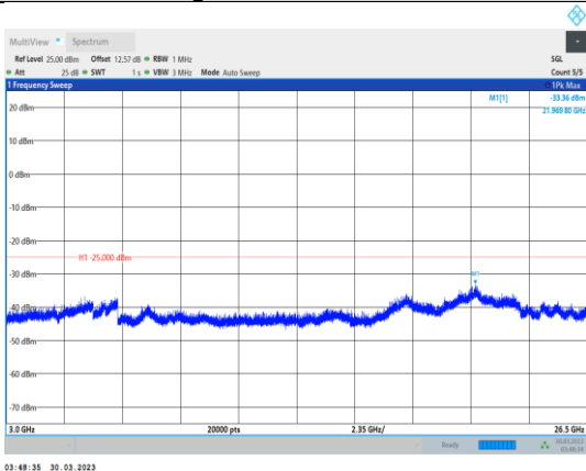
Band7-10MHz-QPSK-21100-1RB#0- Range3:3000~26500MHz
