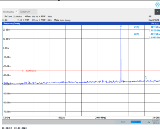
Band7-5MHz-QPSK-20775-1RB#0- Range2:1000~3000MHz
