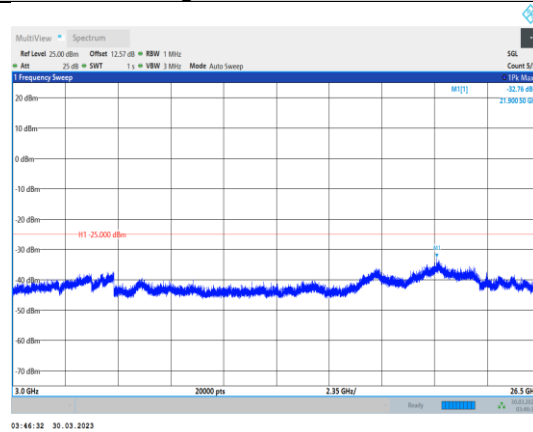
Band7-10MHz-QPSK-20800-1RB#0- Range3:3000~26500MHz
