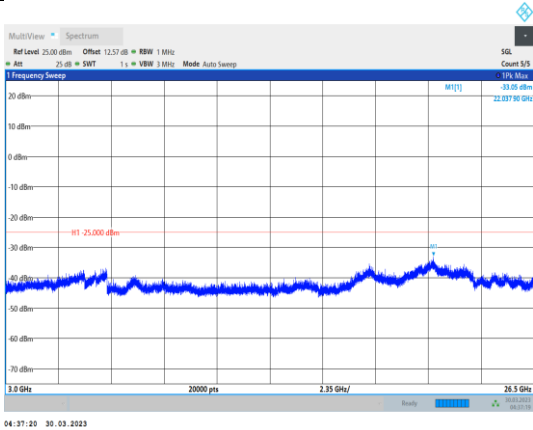
Band7-5MHz-QPSK-21425-1RB#0- Range3:3000~26500MHz
