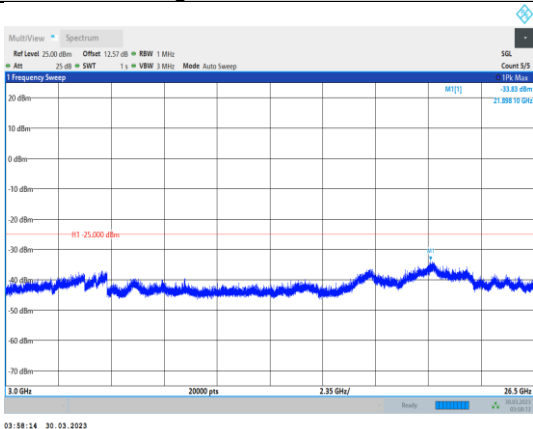
Band7-15MHz-QPSK-20825-1RB#0- Range3:3000~26500MHz
