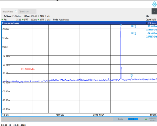
Band7-10MHz-QPSK-21100-1RB#0- Range2:1000~3000MHz
