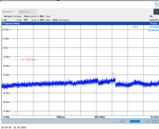
Band5-5MHz-QPSK-20425-1RB#0- Range2:1000~10000MHz
