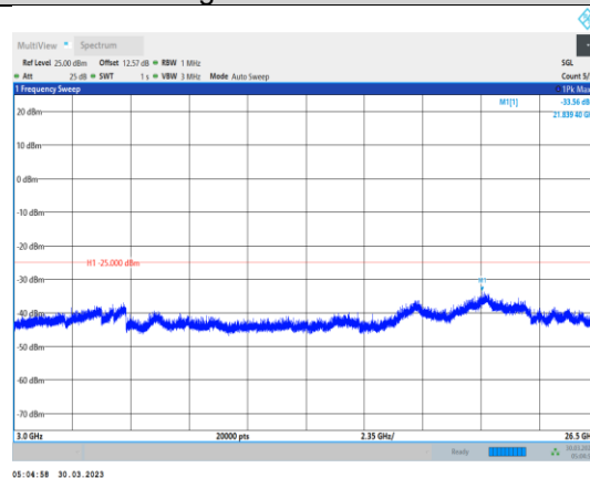
Band7-20MHz-QPSK-21350-1RB#0- Range3:3000~26500MHz
