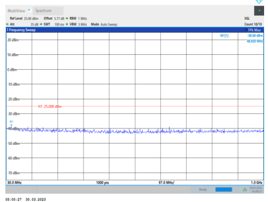
Band7-20MHz-QPSK-20850-1RB#0- Range1:30~1000MHz
