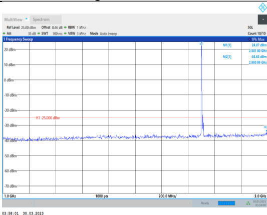
Band7-15MHz-QPSK-20825-1RB#0- Range2:1000~3000MHz
