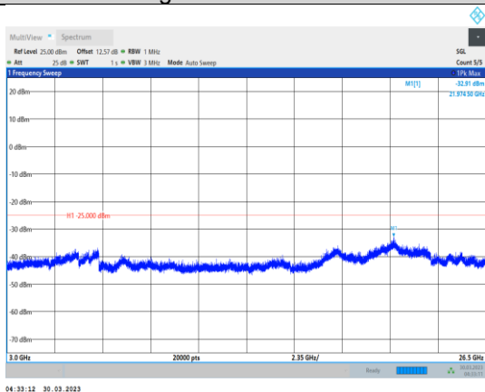
Band7-5MHz-QPSK-20775-1RB#0- Range3:3000~26500MHz
