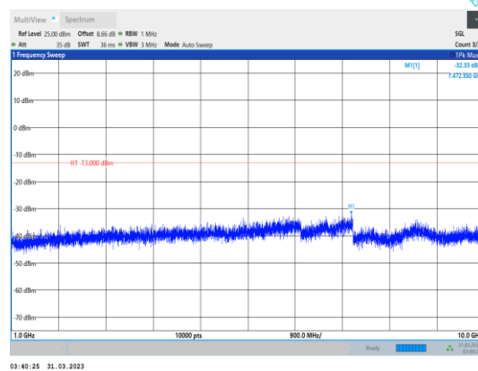
Band5-5MHz-QPSK-20525-1RB#0- Range2:1000~10000MHz
