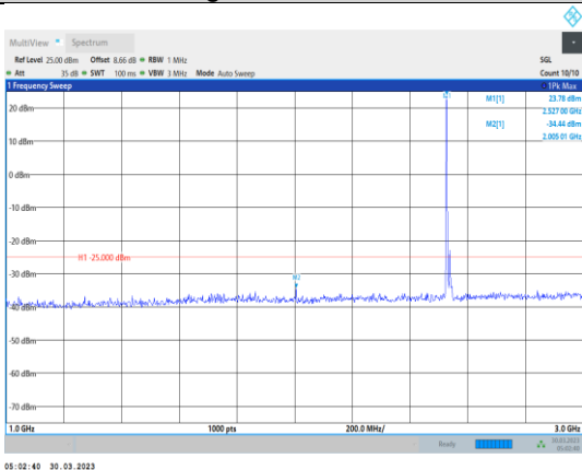
Band7-20MHz-QPSK-21100-1RB#0- Range2:1000~3000MHz
