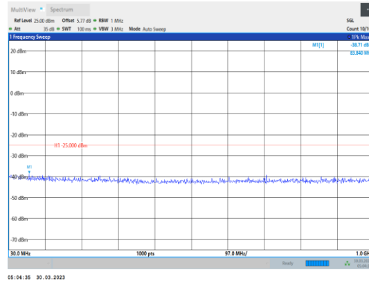
Band7-20MHz-QPSK-21350-1RB#0- Range1:30~1000MHz
