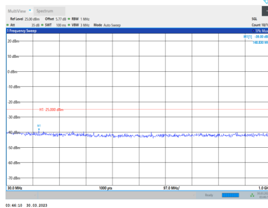
Band7-10MHz-QPSK-20800-1RB#0- Range1:30~1000MHz
