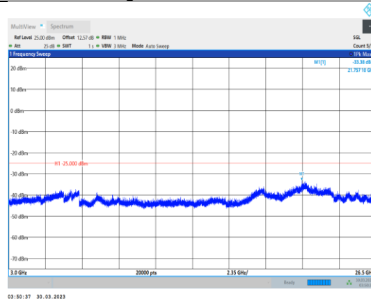
Band7-10MHz-QPSK-21400-1RB#0- Range3:3000~26500MHz
