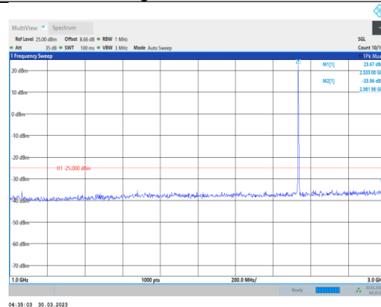
Band7-5MHz-QPSK-21100-1RB#0- Range2:1000~3000MHz
