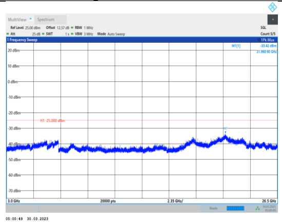
Band7-20MHz-QPSK-20850-1RB#0- Range3:3000~26500MHz
