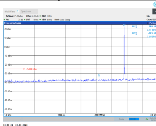
Band7-10MHz-QPSK-21400-1RB#0- Range2:1000~3000MHz
