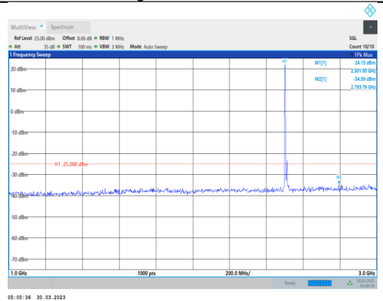
Band7-20MHz-QPSK-20850-1RB#0- Range2:1000~3000MHz
